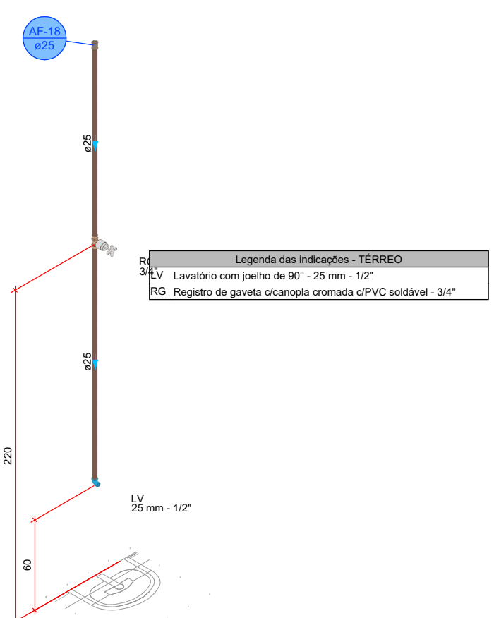
DETALHE HID-18 1:25
