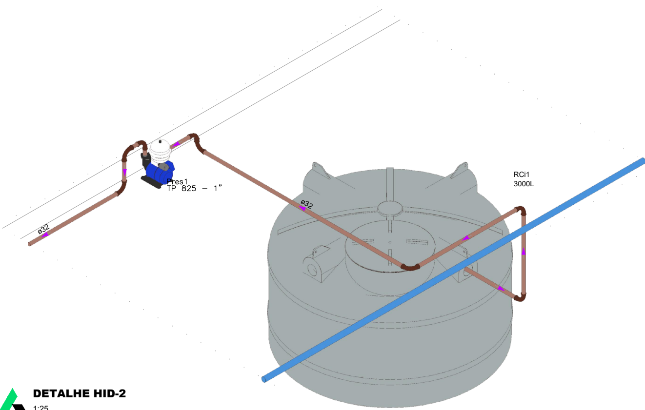
DETALHE HID-2 1/25
