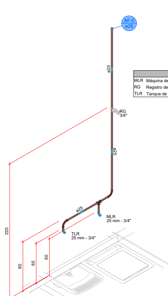
DETALHE HID-6 1/25
