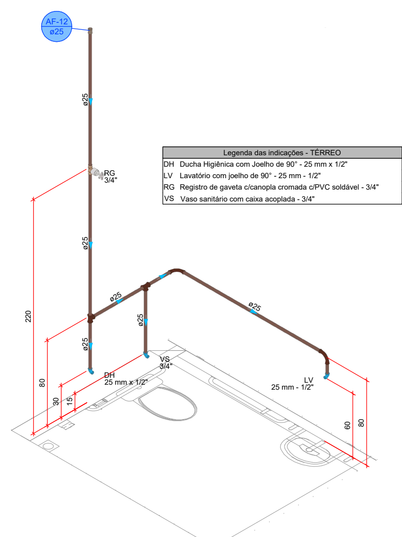
DETALHE HID-12 1/25
