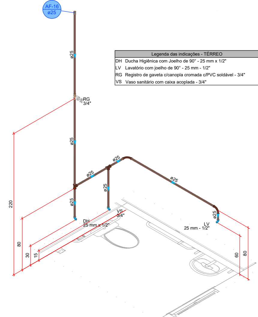
DETALHE HID-17 1:25
