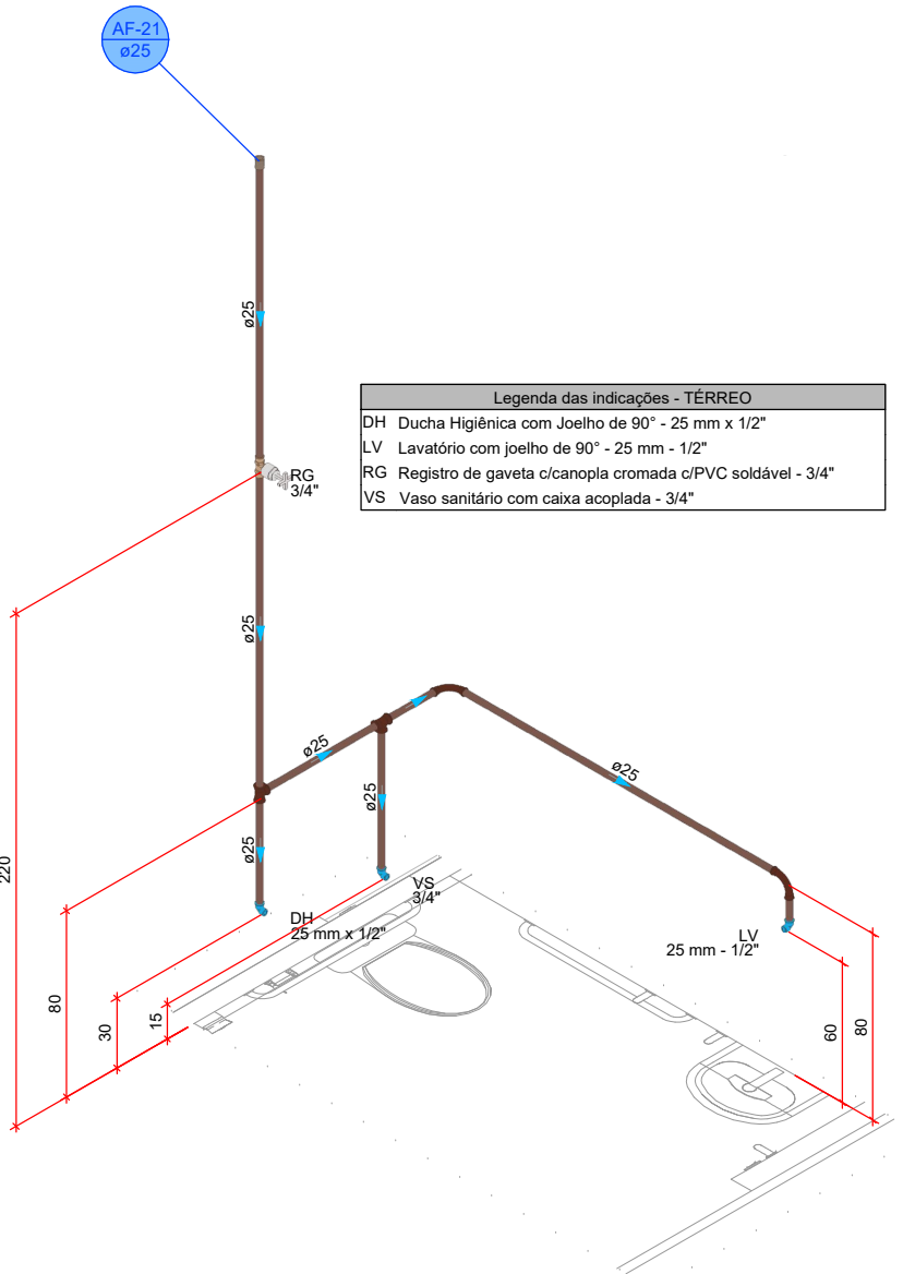
DETALHE HID-21 1:25
