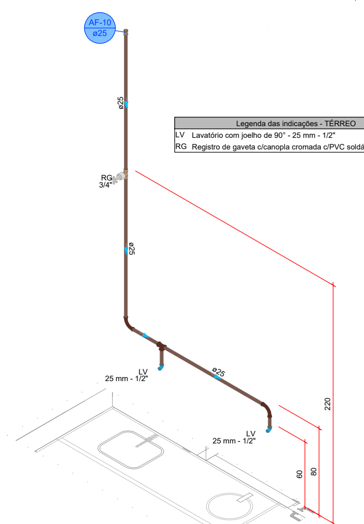
DETALHE HID-10 1/25
