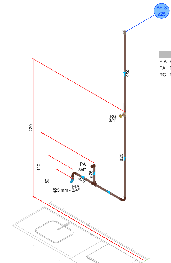
DETALHE HID-3 1/25
