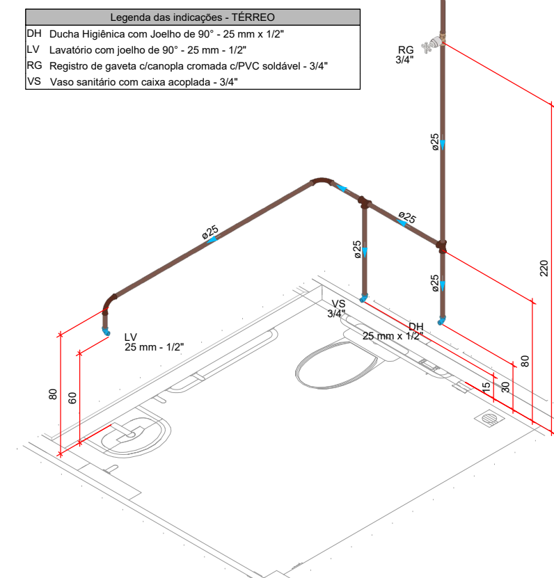
DETALHE HID-16 1:25
