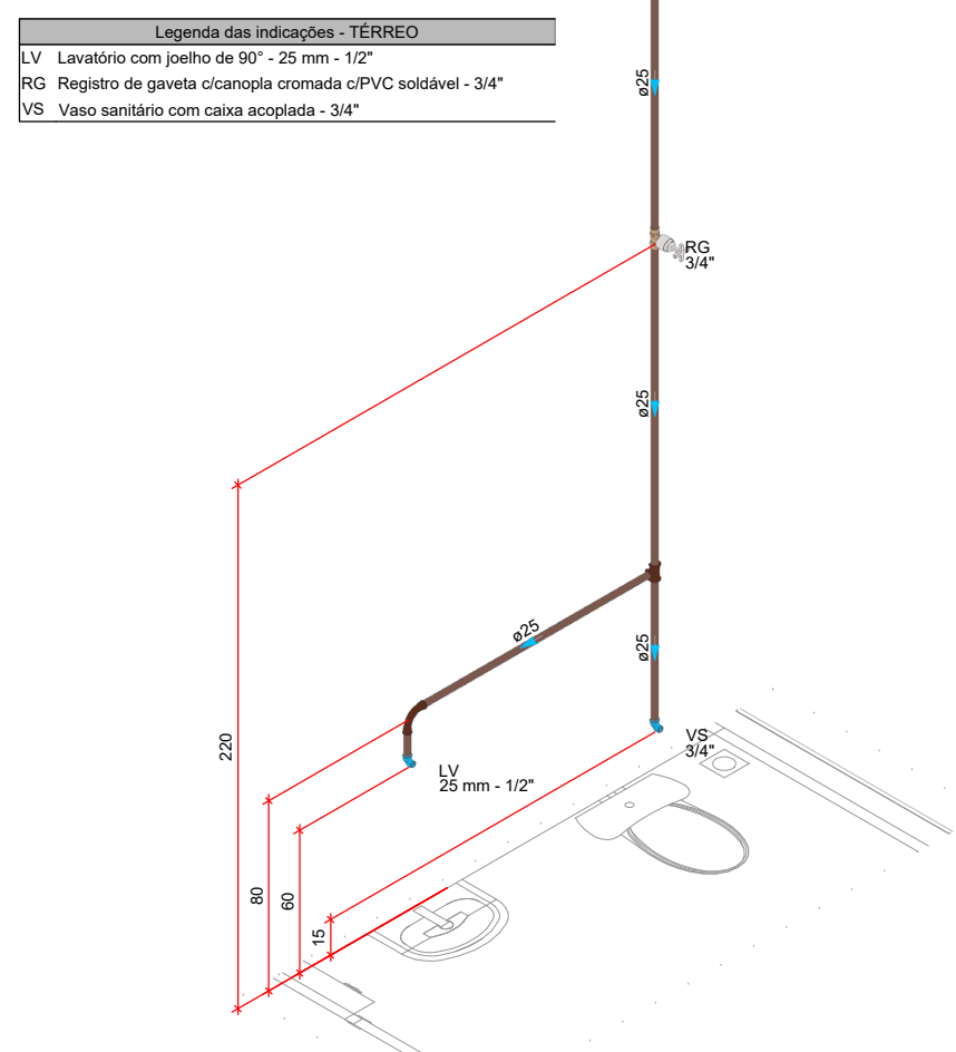
DETALHE HID-22 1:25
