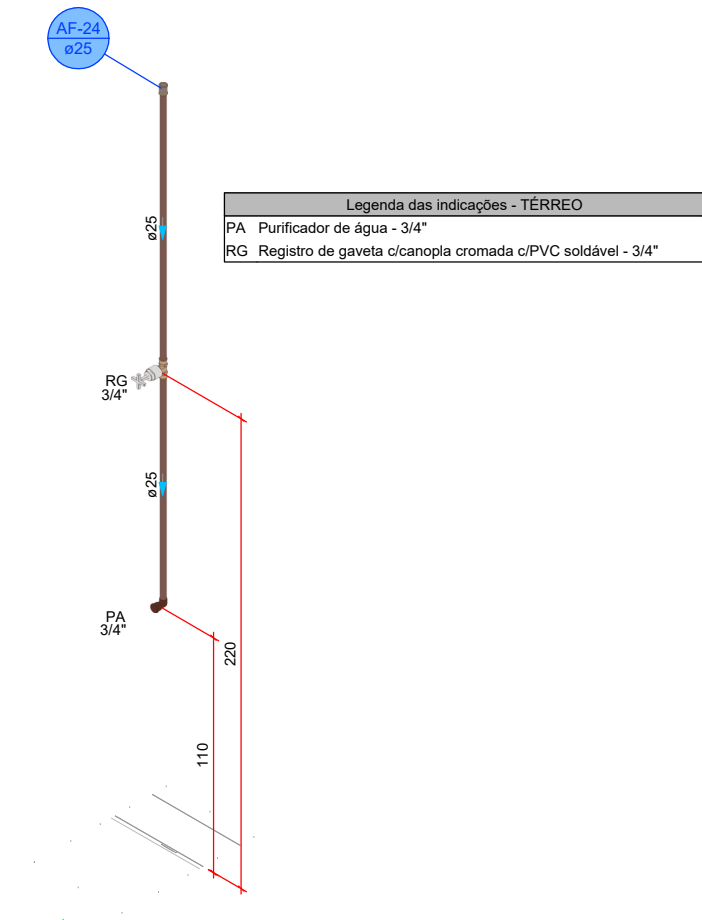
DETALHE HID-24 1:25
