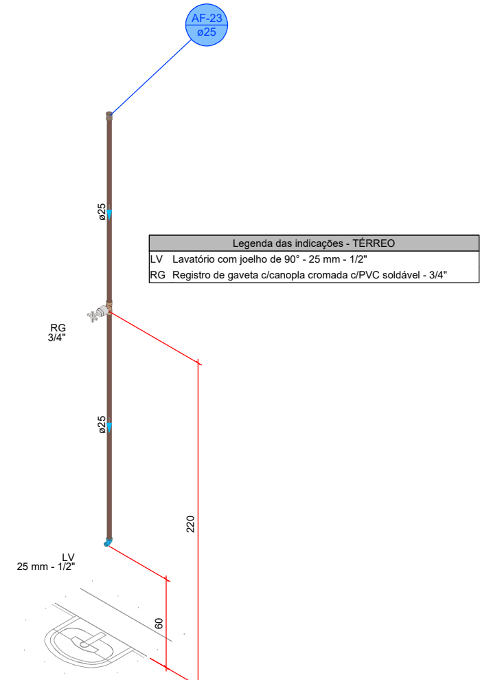
DETALHE HID-23 1:25
