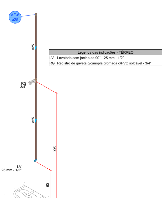
DETALHE HID-7 1/25
