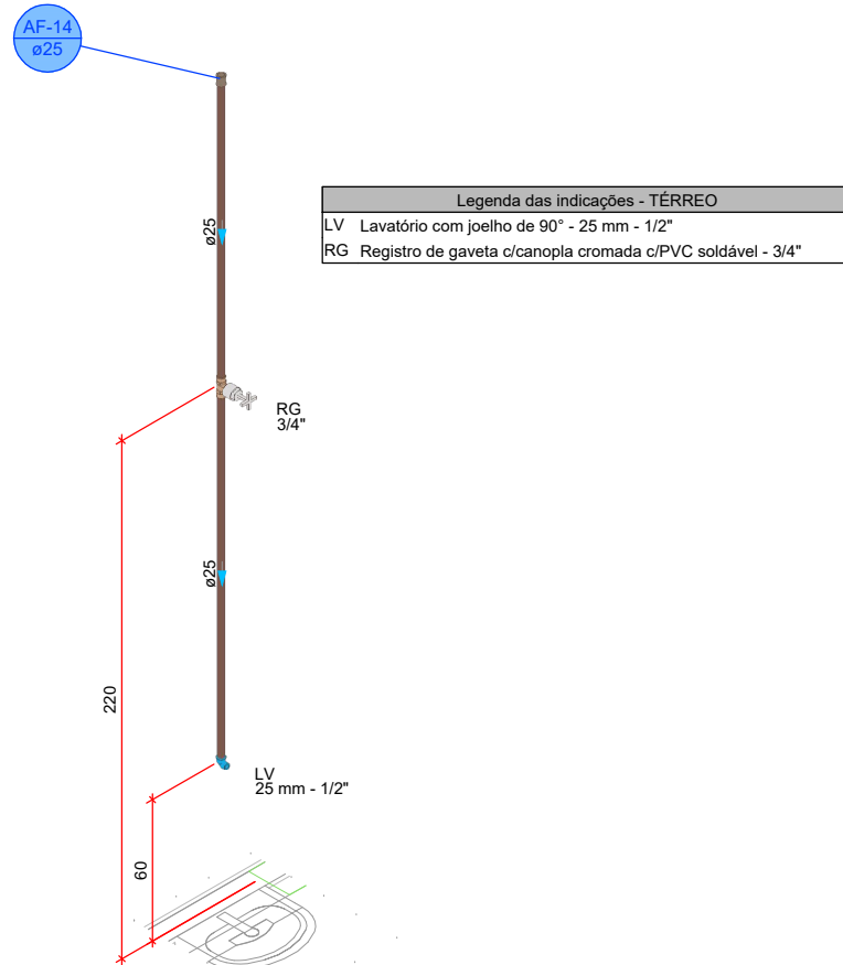
DETALHE HID-15 1:25
