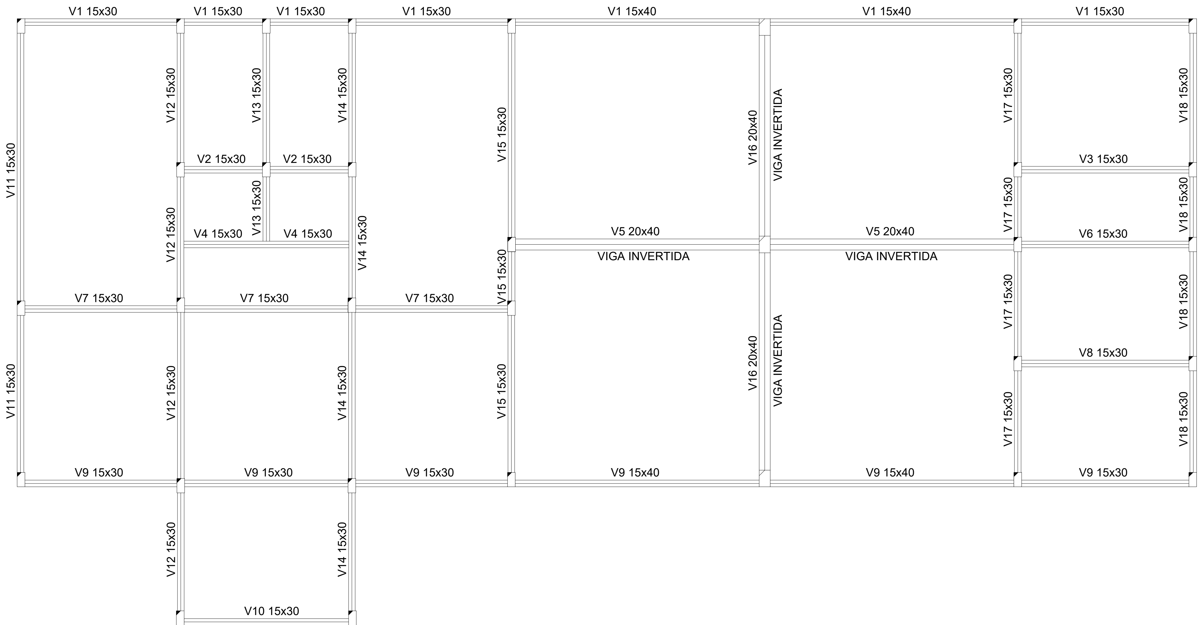
01 VIGAS SUPERIORES ESG: 1/40
