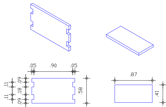
1 DETALHES DAS PEÇAS DAS TESTEIRAS E TAMPA ESCALA 1/50
