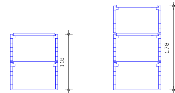
4 CORTES DAS 03 DISPOSIÇÕES ESCALA 1/50
