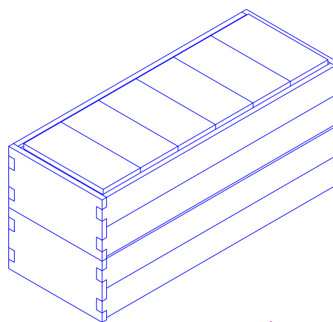
6 VISTA ISOMÉTRICA COM 02 GAVETA ESCALA S/E
