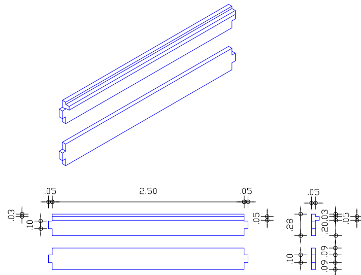
2 DETALHES DAS PEÇAS DE FECHAMENTO LATERAL ESCALA 1/50
