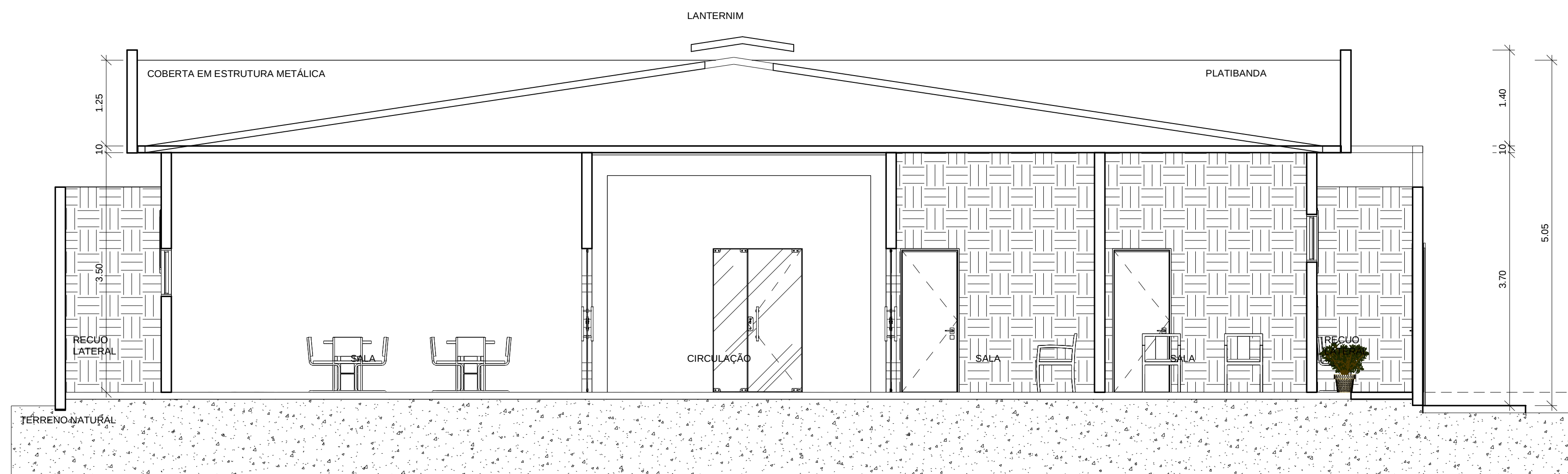
3 CORTE TRANSVERSAL BB 1 : 50
