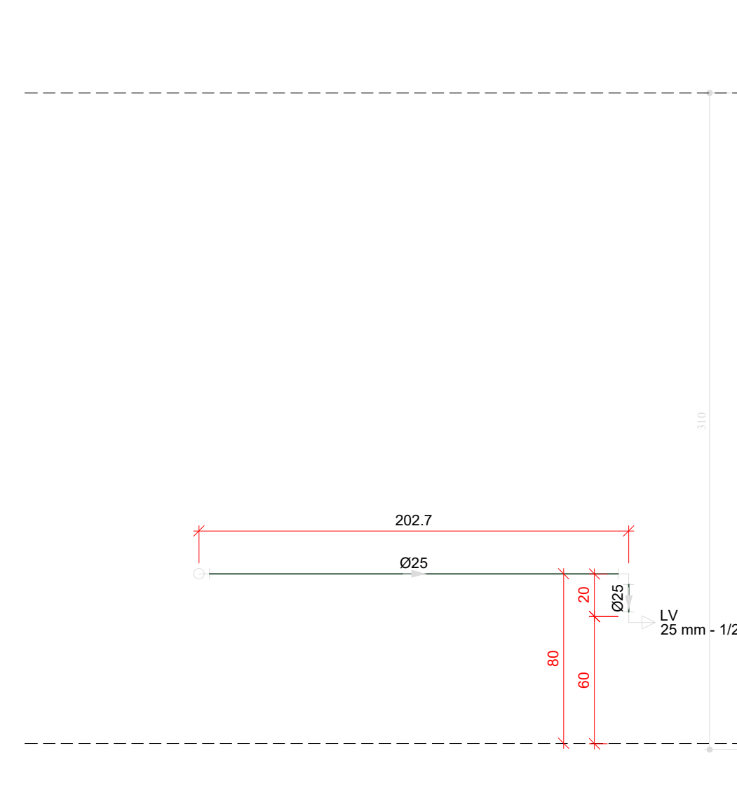
H29 DETALHE H29 ESCALA 1/25
