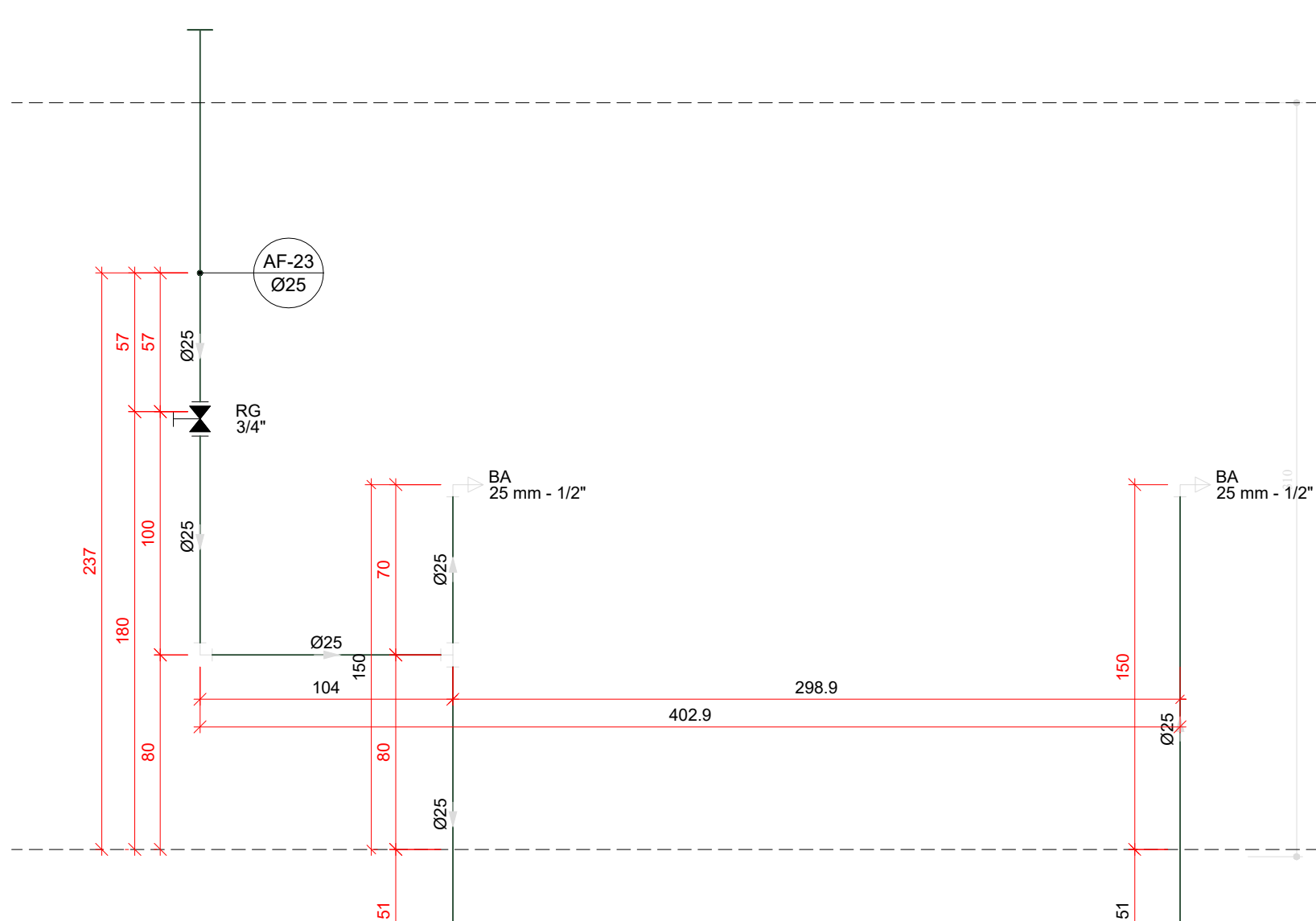
H27 DETALHE H27 ESCALA 1/25
