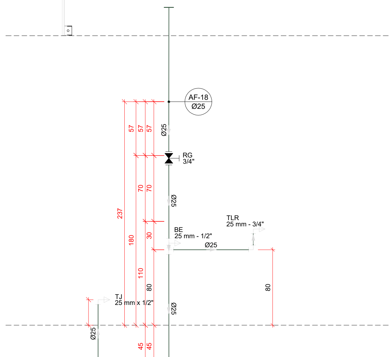
H28 DETALHE H28 ESCALA 1/25
