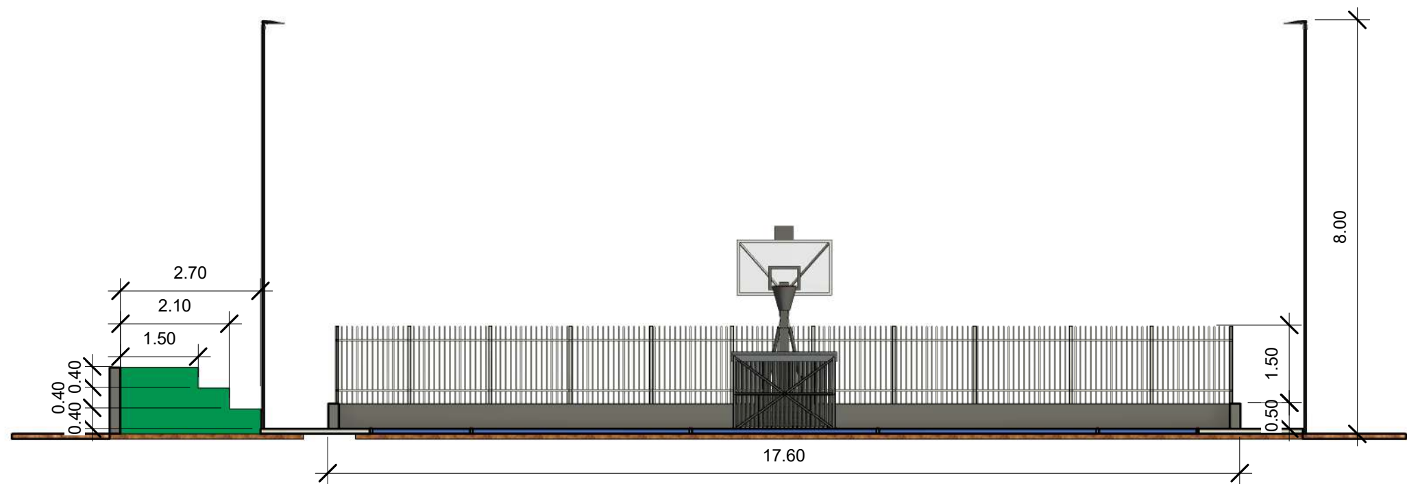
2 Corte 02 1 : 100
