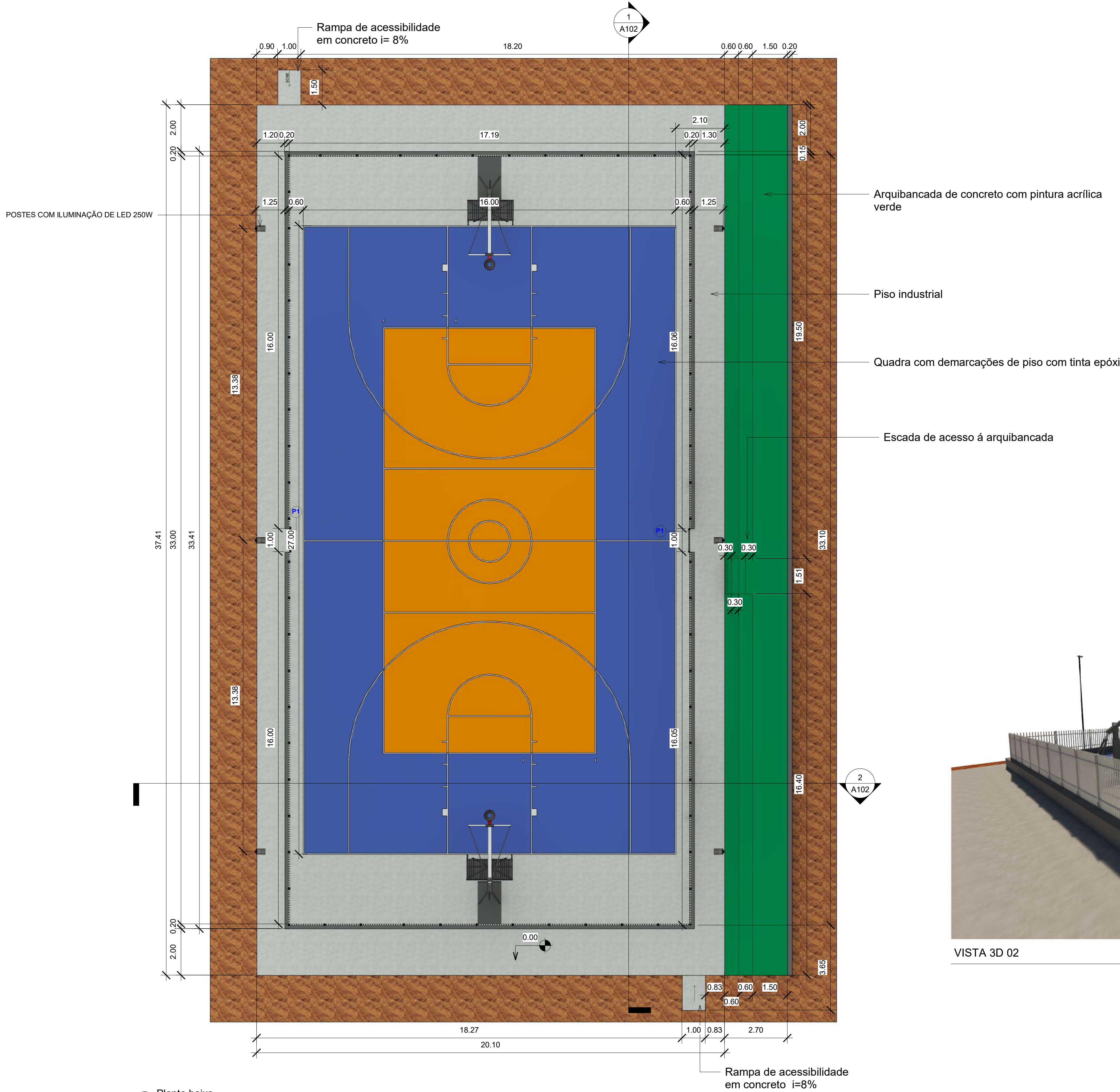
1 Planta baixa 1 : 100
