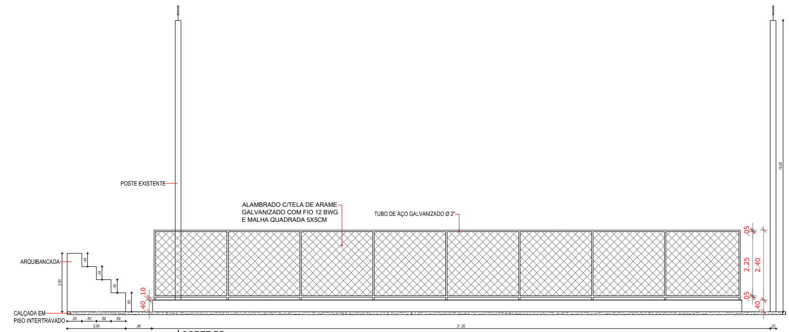
03 | CORTE BB ESC.: 1/130
