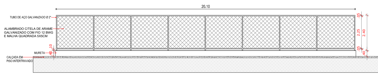
05 | VISTA - 02 ESC.: 1/130
