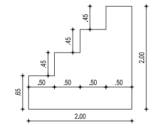
10 | DET. ARQUIBANCADA ESC.: 1/75
