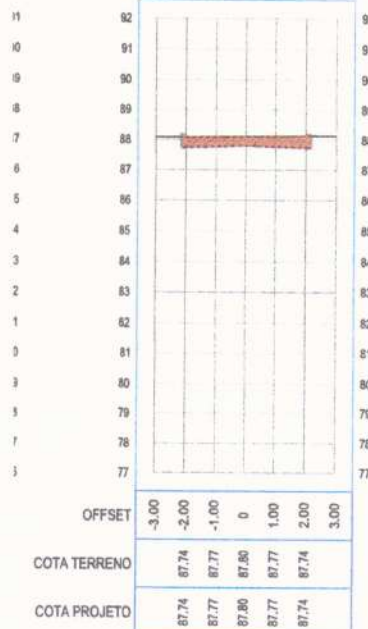
SEÇÃO TRANSVERSAL: 32+0.00
