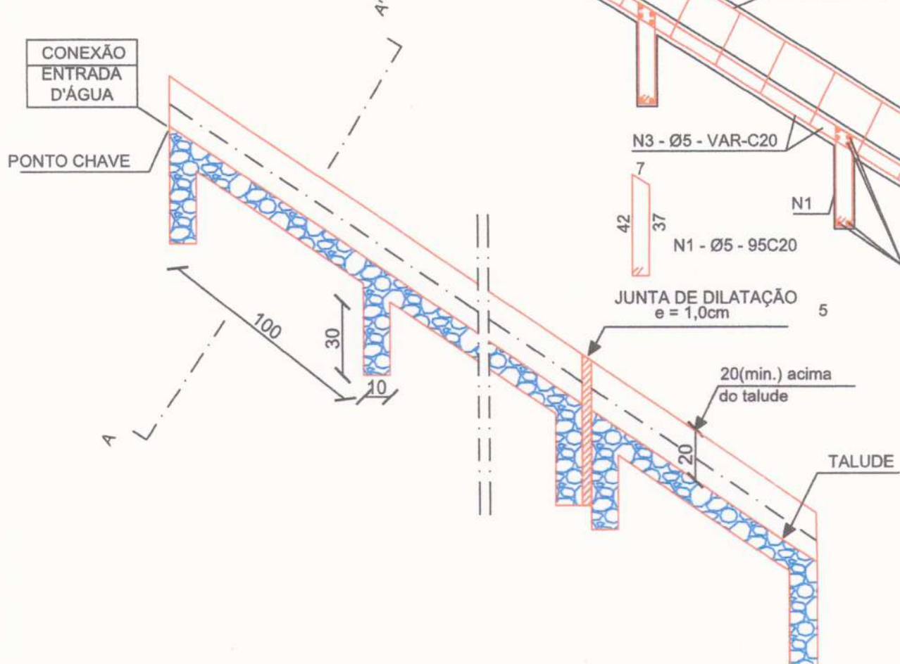
CORTE TRANSVERSAL AA'
