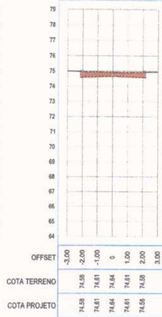
SEÇÃO TRANSVERSAL: 6+0.00
