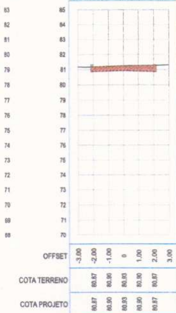
SEÇÃO TRANSVERSAL: 14+0.00
