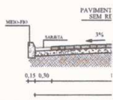
4 DETALHE MEIO - FIO SEM ESCALA
