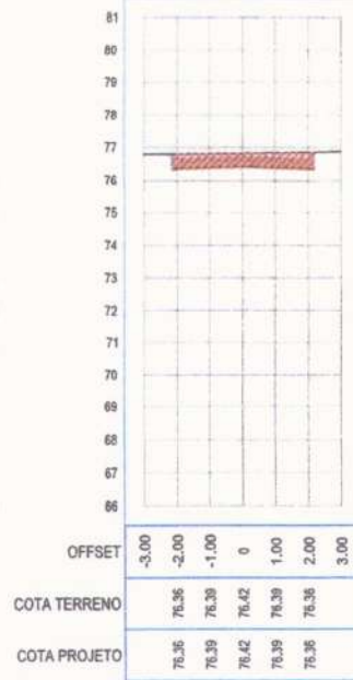
SEÇÃO TRANSVERSAL: 8+0.00
