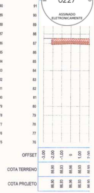
SEÇÃO TRANSVERSAL: 28+0.00
