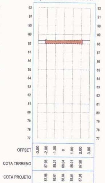
SEÇÃO TRANSVERSAL: 34+0.00
