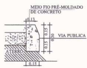
4 DETALHE MEIO - FIO SEM ESCALA
