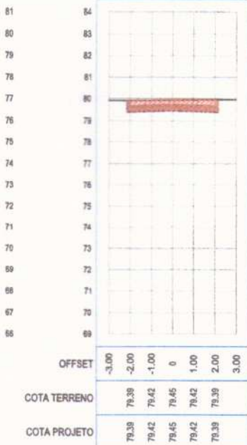
SEÇÃO TRANSVERSAL: 12+0.00
