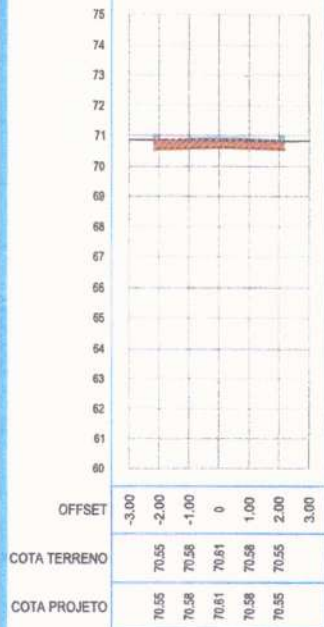
SEÇÃO TRANSVERSAL: 1+0.00
