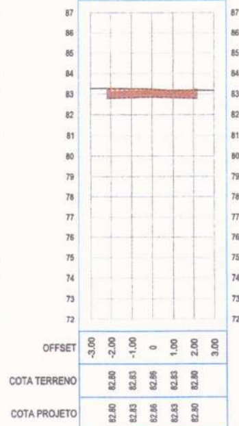
SEÇÃO TRANSVERSAL: 17+0.00
