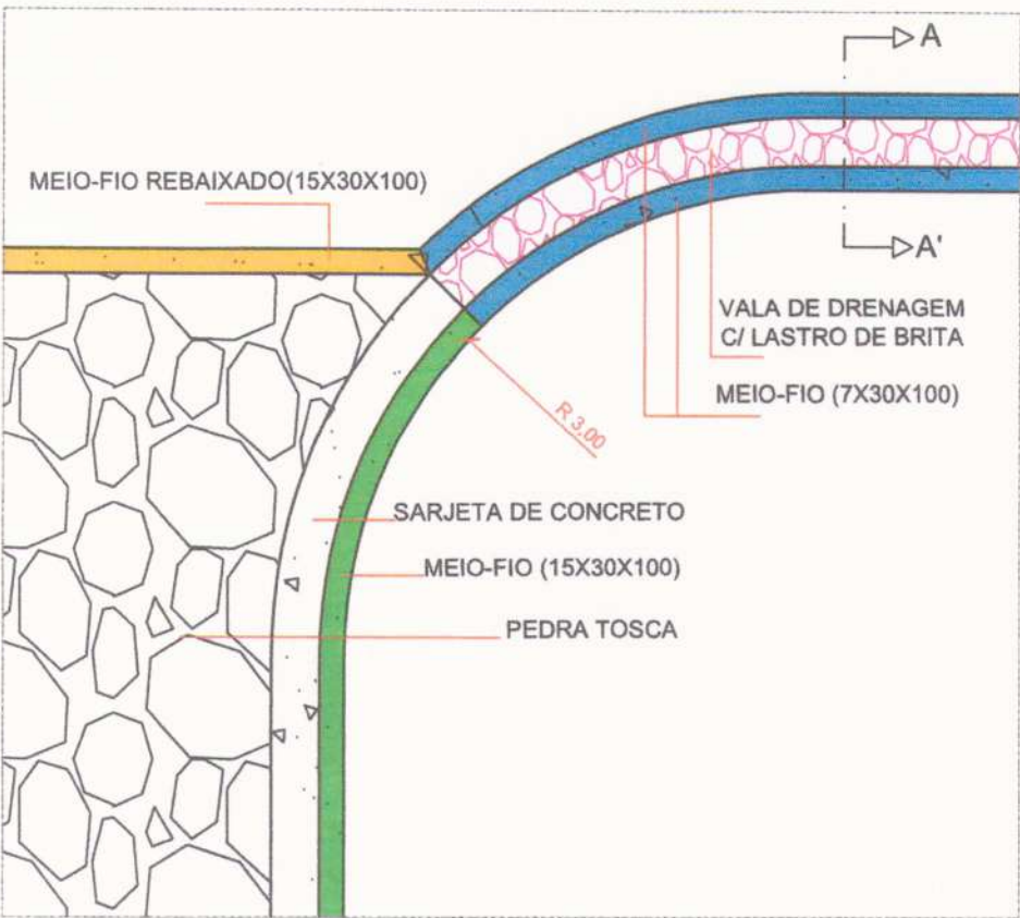
DET 01 SEM ESCALA
