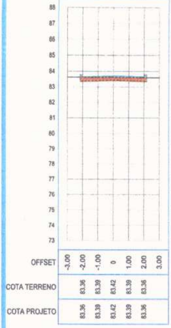
SEÇÃO TRANSVERSAL: 19+0.00
