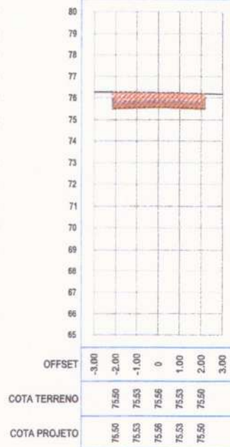
SEÇÃO TRANSVERSAL: 7+0.00
