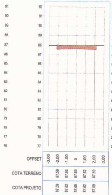
SEÇÃO TRANSVERSAL: 31+0.00
