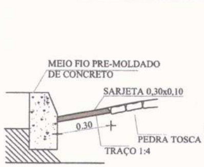
2 DETALHE SARJETA SEM ESCALA
