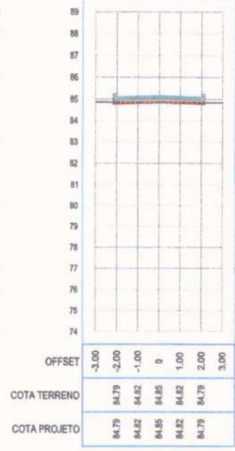
SEÇÃO TRANSVERSAL: 22+0.00
