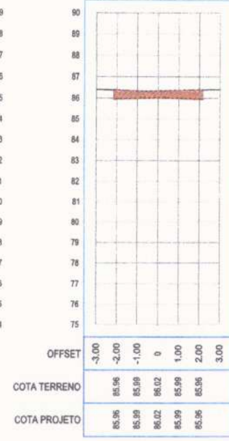
SEÇÃO TRANSVERSAL: 25+0.00
