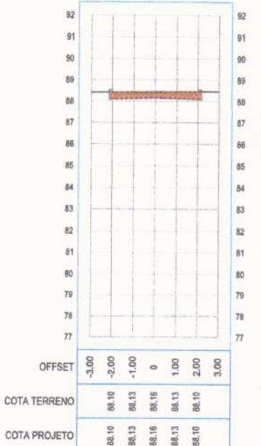
SEÇÃO TRANSVERSAL: 35+0.00
