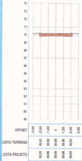
SEÇÃO TRANSVERSAL: 0+0.00
