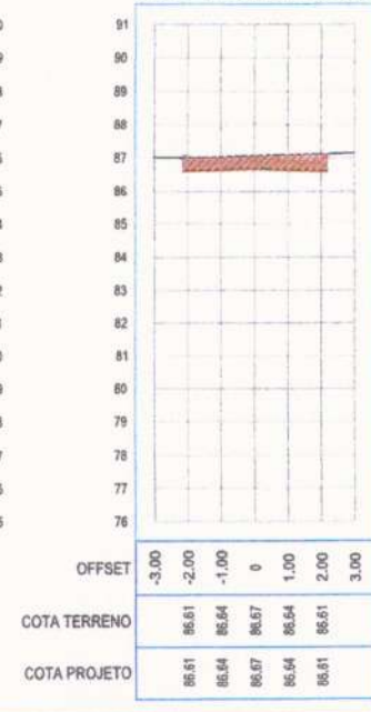
SEÇÃO TRANSVERSAL: 26+0.00
