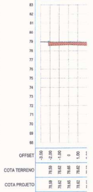
SEÇÃO TRANSVERSAL: 11+0.00
