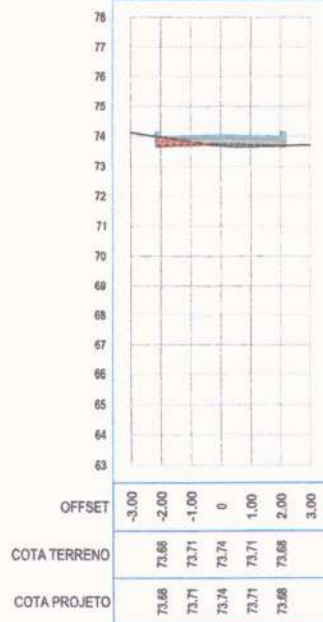
SEÇÃO TRANSVERSAL: 5+0.00
