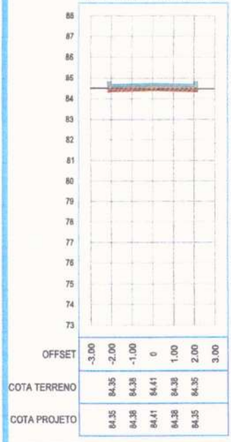
SEÇÃO TRANSVERSAL: 20+0.00
