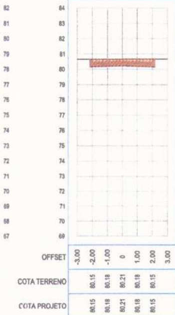
SEÇÃO TRANSVERSAL: 13+0.00
