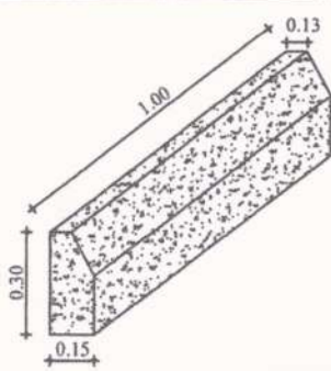
3 DETALHE MEIO - FIO SEM ESCALA
