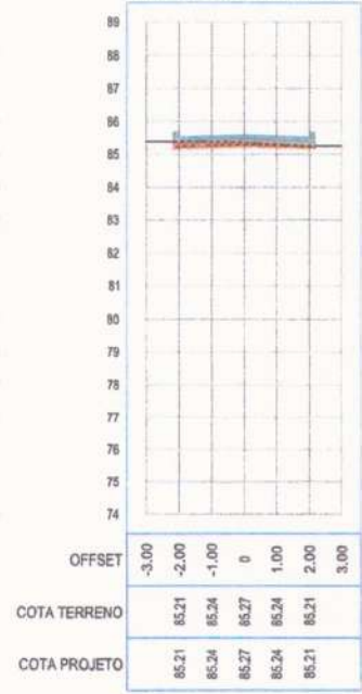
SEÇÃO TRANSVERSAL: 23+0.00
