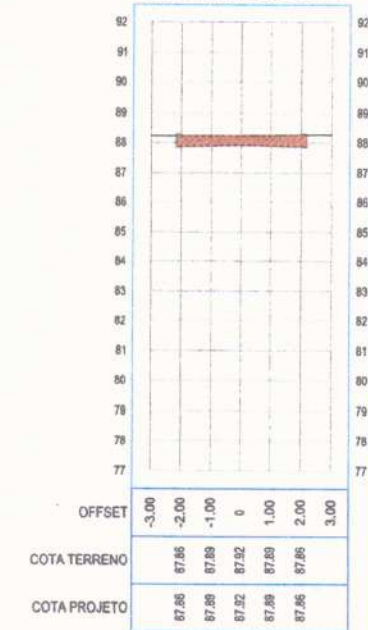
SEÇÃO TRANSVERSAL: 32+0.00
