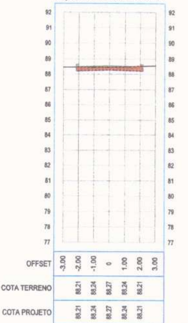
SEÇÃO TRANSVERSAL: 35+0.00
