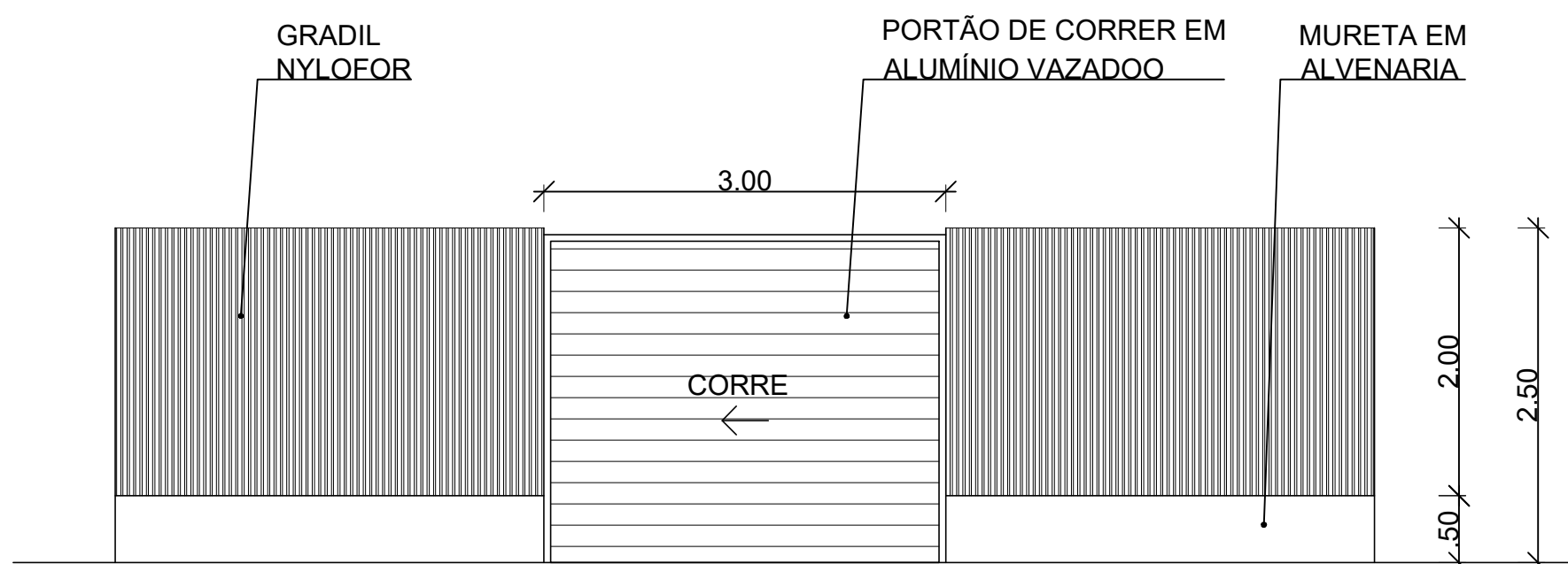
2 DETALHE MURO FACHADA ESCALA 1/100
