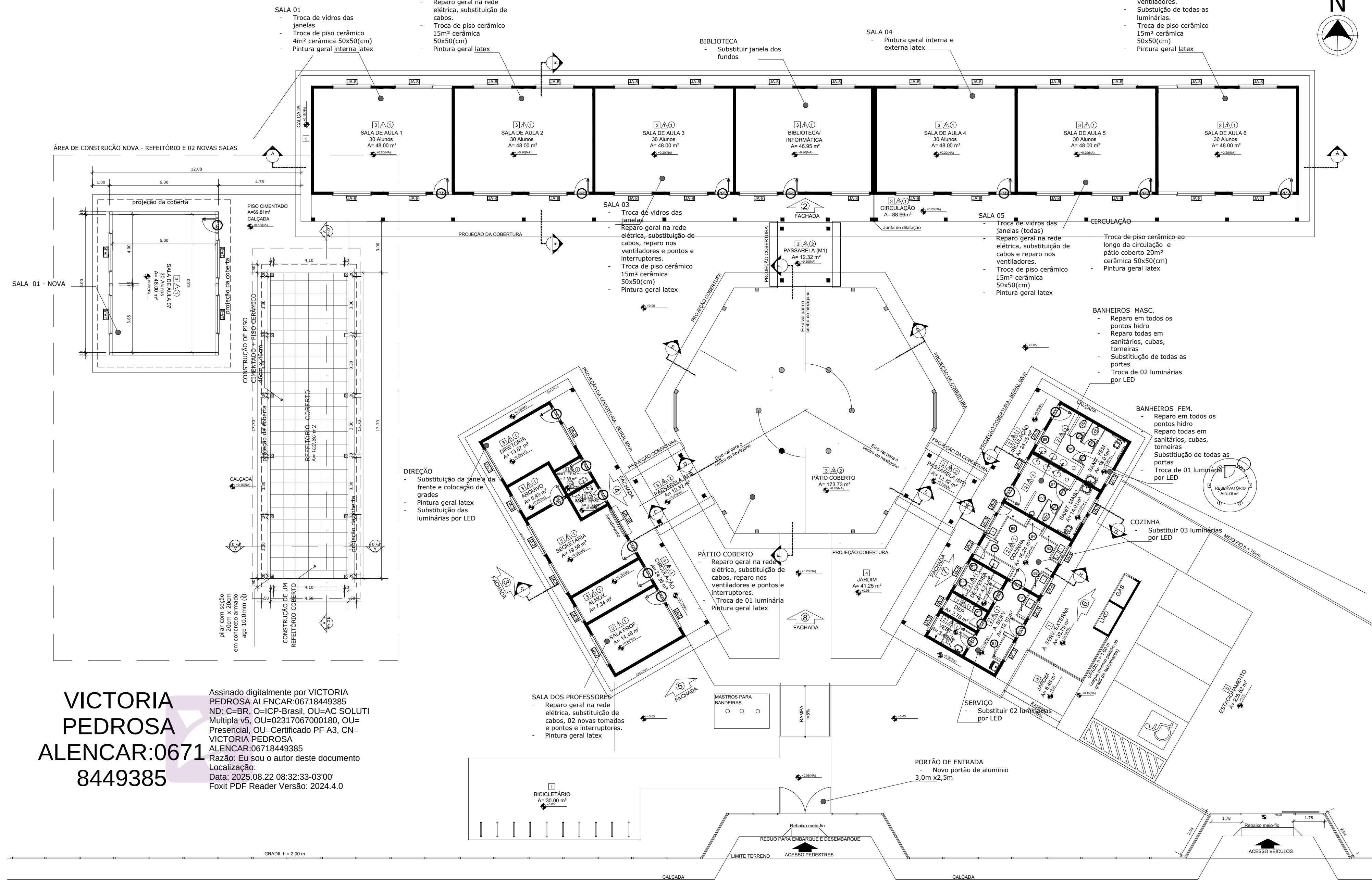
01 PLANTA BAIXA - ILUMINADA
