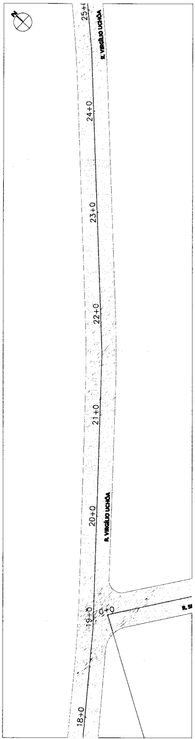
02 | PLANTA BAIXA - R. VIRGÍLIO UCHÔA esc.: 1:250
