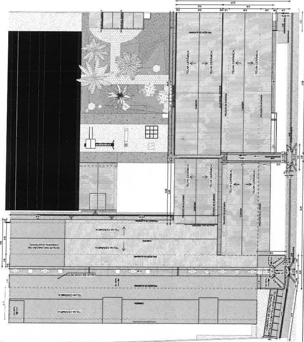
2 | PLANTA DE COBERTA E LOCAÇÃO - CONSTRUIR 1:150
