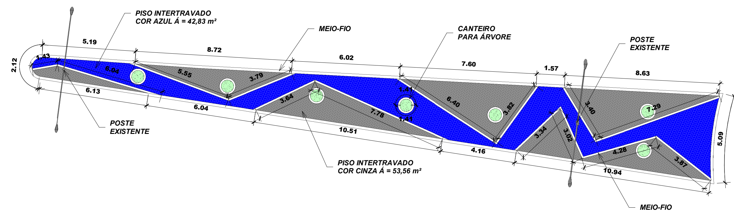
2 CANTEIRO 02 E ROTATÓRIA 01 - PROJETOADO 1 : 125
