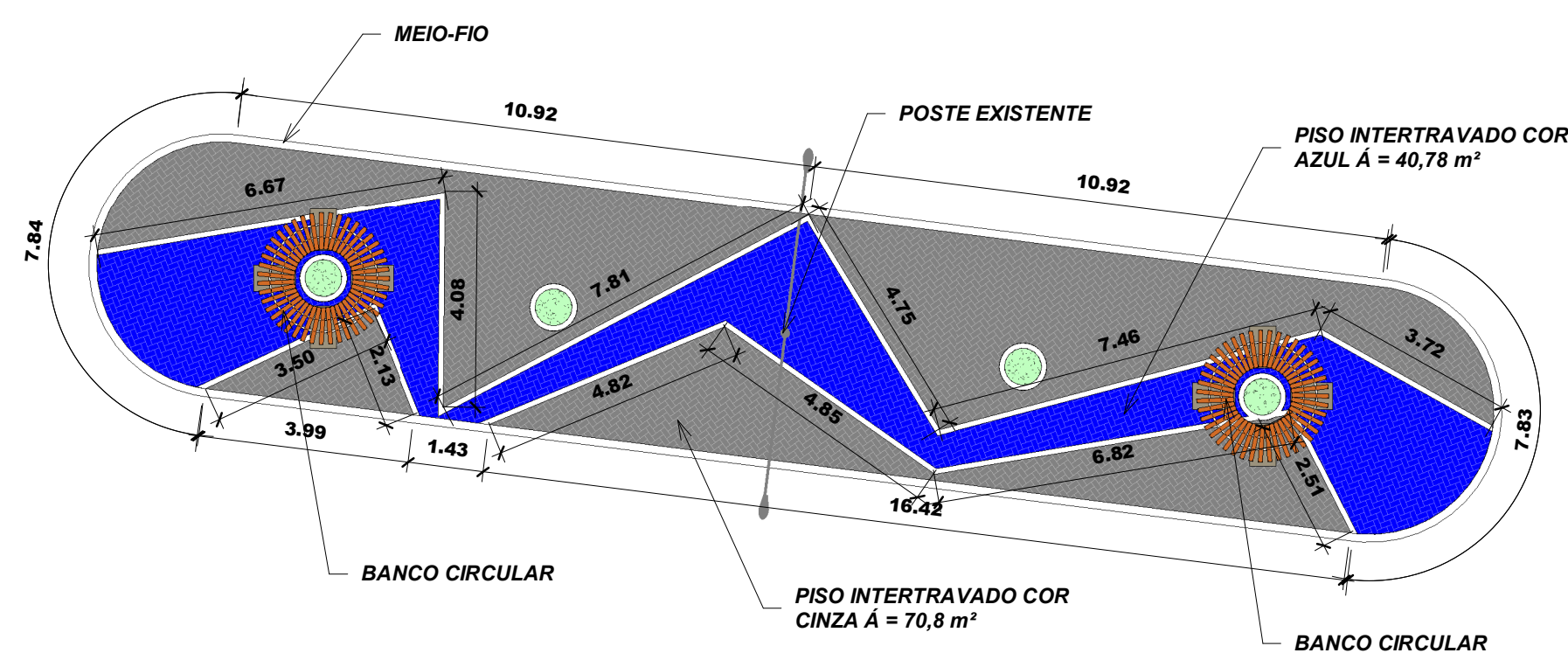
4 CANTEIRO 04 E 05 - PROJETOADO 1 : 125
