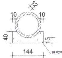
DETALHE DO BERÇO E DENTE INTERMEDIÁRIO DE BUEIRO SIMPLES TUBULAR DE CONCRETO BSTC Ø 100 cm
