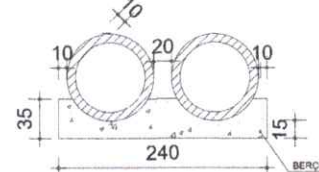
DETALHE DO BERÇO E DENTE INTERMEDIÁRIO DE BUEIRO DUPLO TUBULAR DE CONCRETO BDTC Ø 80 cm
