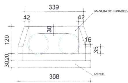
VISTA FRONTAL esc: S/E
