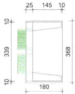
PLANTA BAIXA esc: S/E
