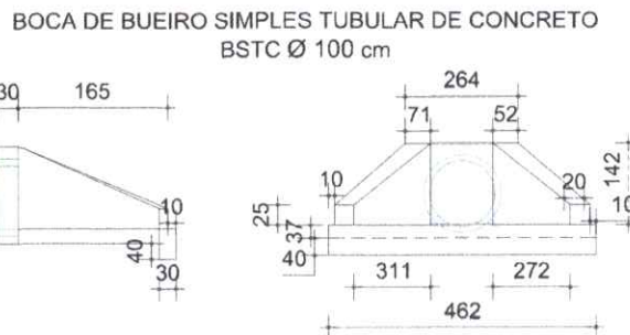
VISTA LATERAL esc: S/E
