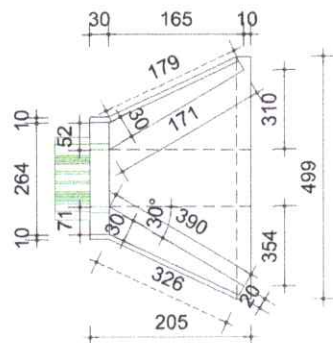
PLANTA BAIXA esc: S/E
