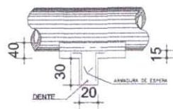
CORTE LONGITUDINAL esc: S/E
