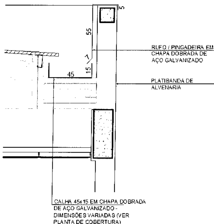
Figura 12 – imagem exemplificativa de detalhe da calha e ruf/pingadeira
