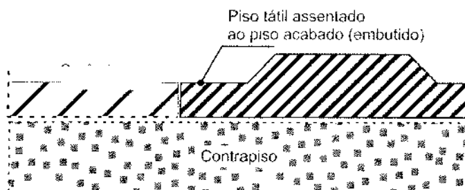
Figura 18 – imagem exemplificativa do assentamento de piso tátil de concreto. Fonte: wstatil.com.br/produto/piso-tatil .
