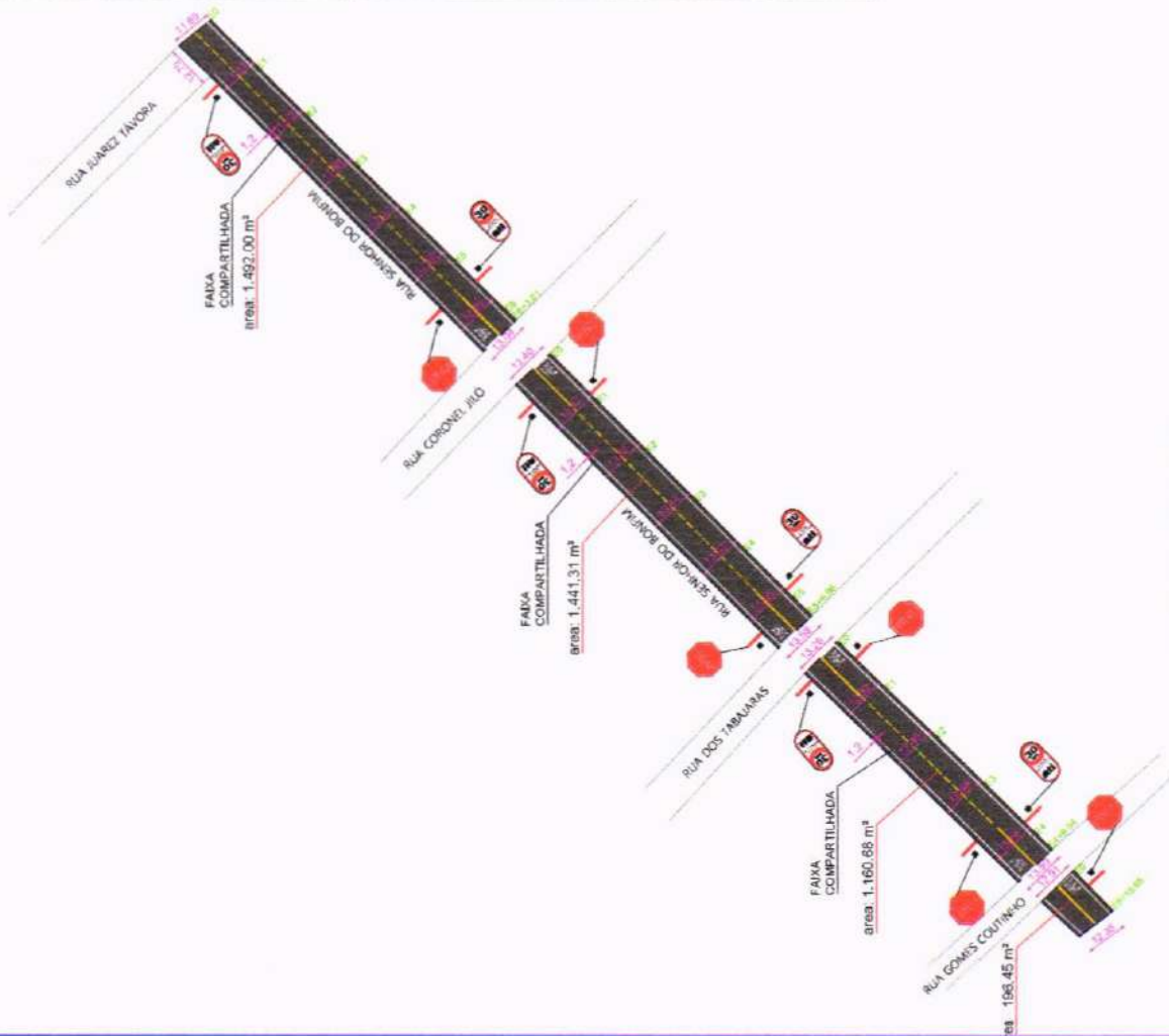
01 PLANTA BAIXA ASFALTO ESCALA — 1 : 750
