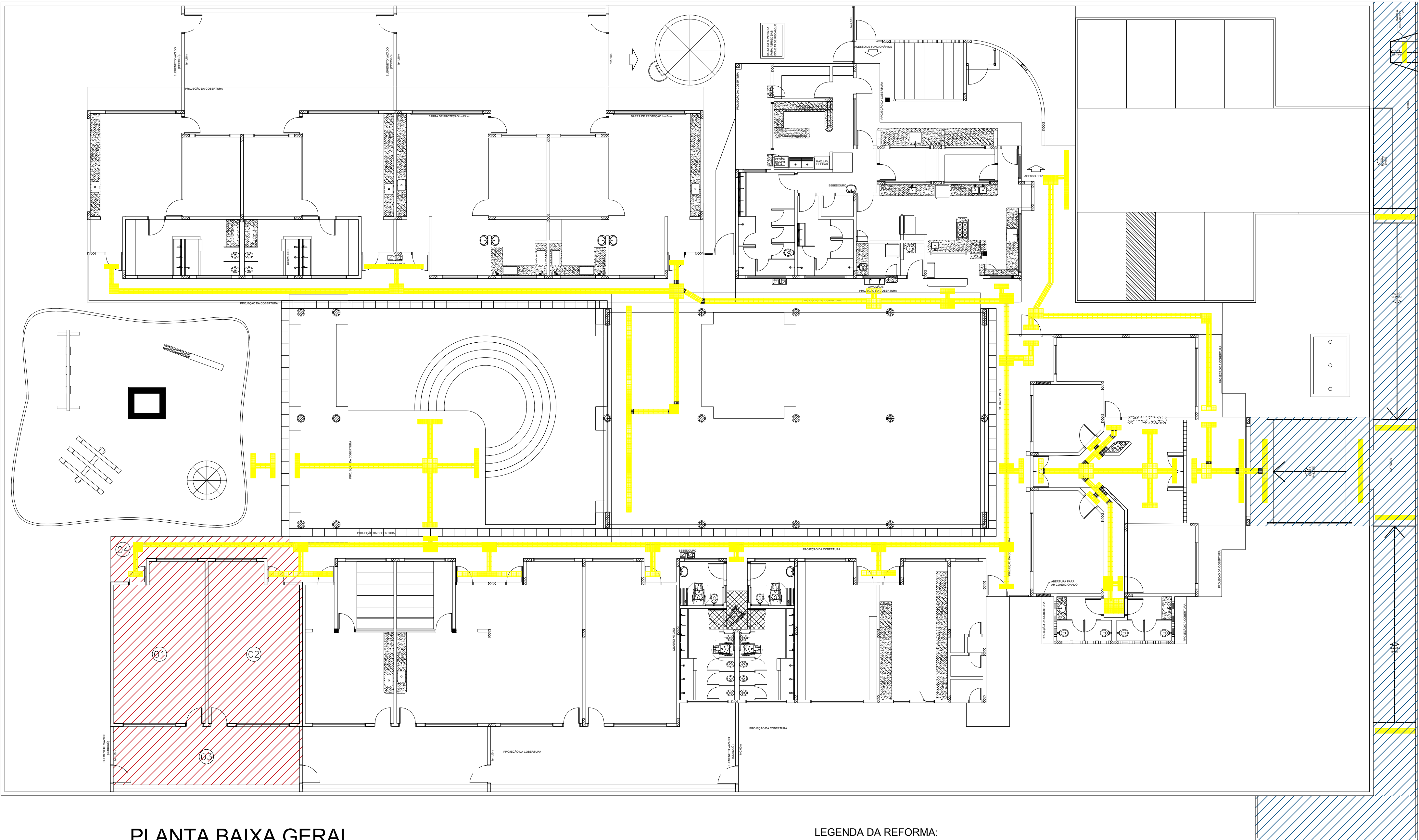
PLANTA BAIXA GERAL esc 1:125
