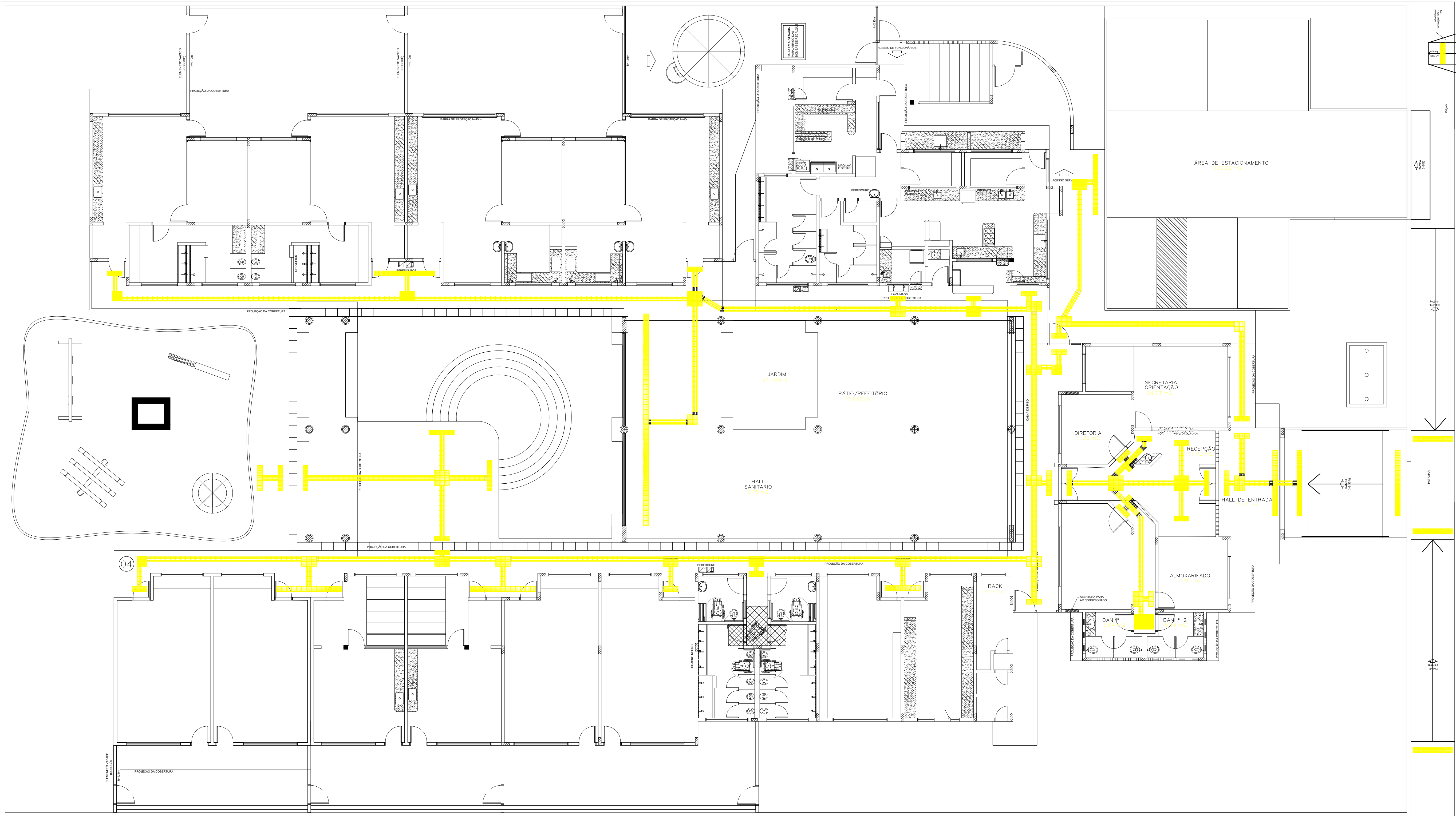
PLANTA BAIXA DE SINALIZAÇÃO DO PISO TÁTIL esc 1:125
