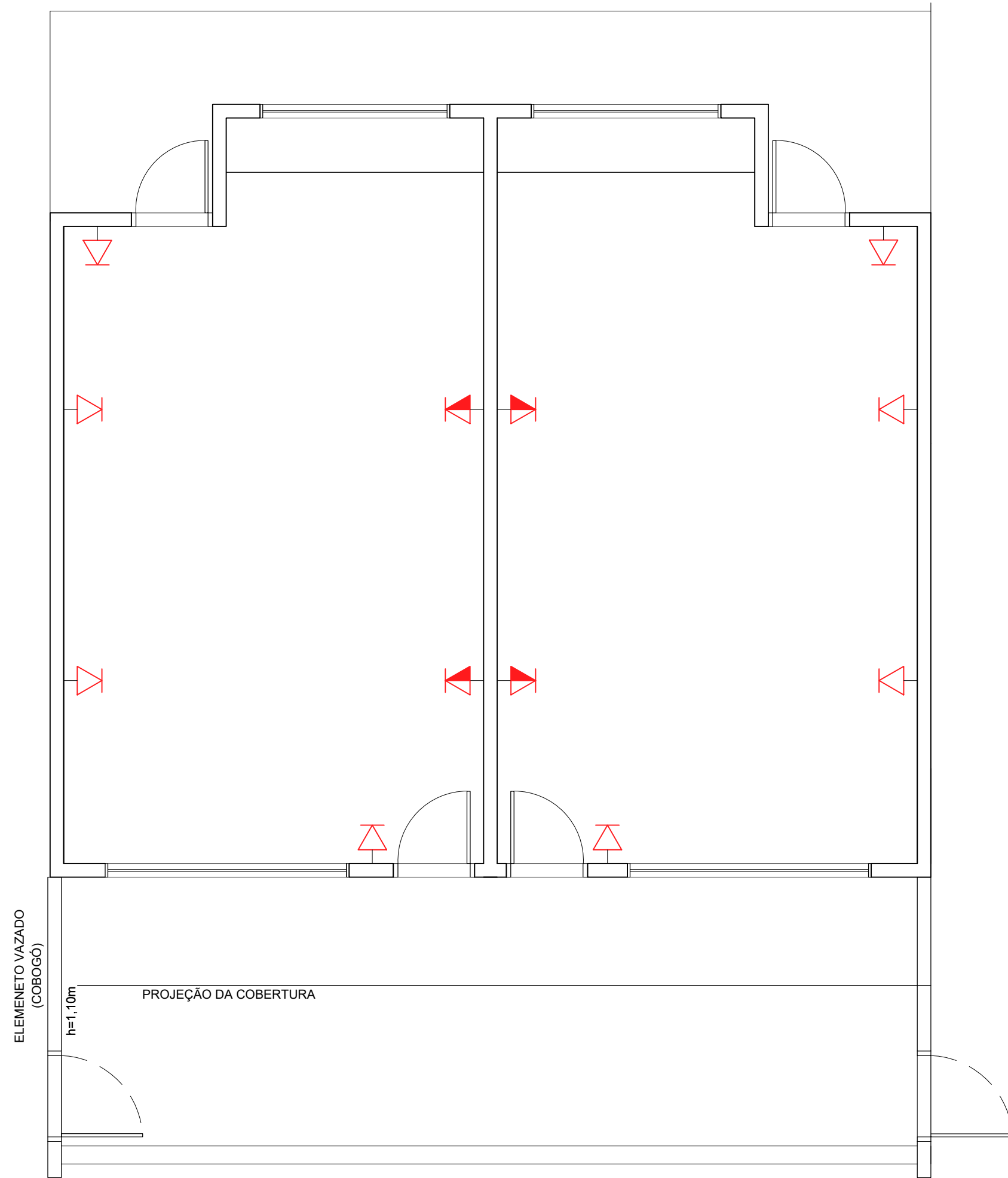
MAPA DE PONTOS ELETRICOS esc 1:50
