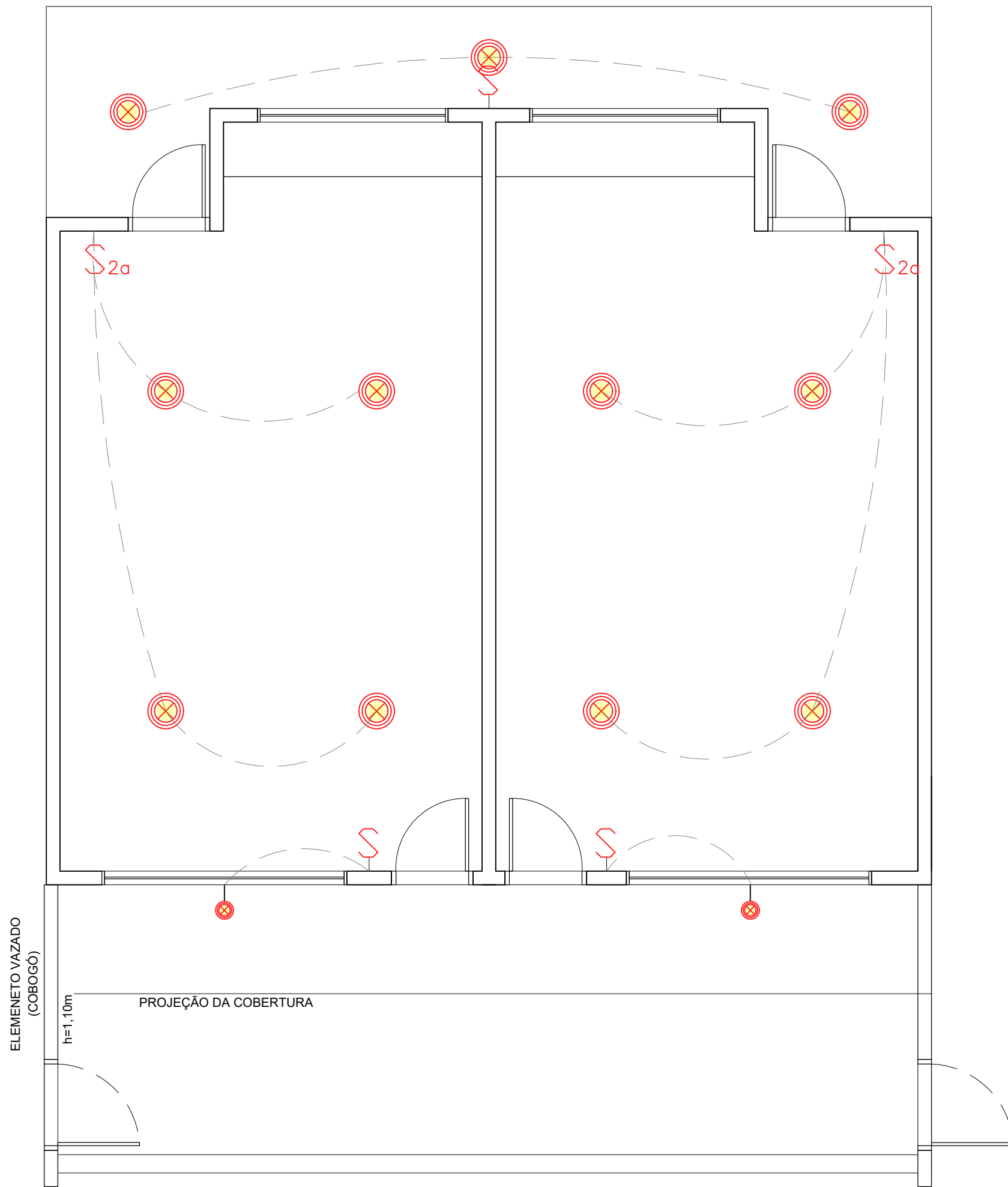
MAPA DE ILUMINAÇÃO esc 1:50
