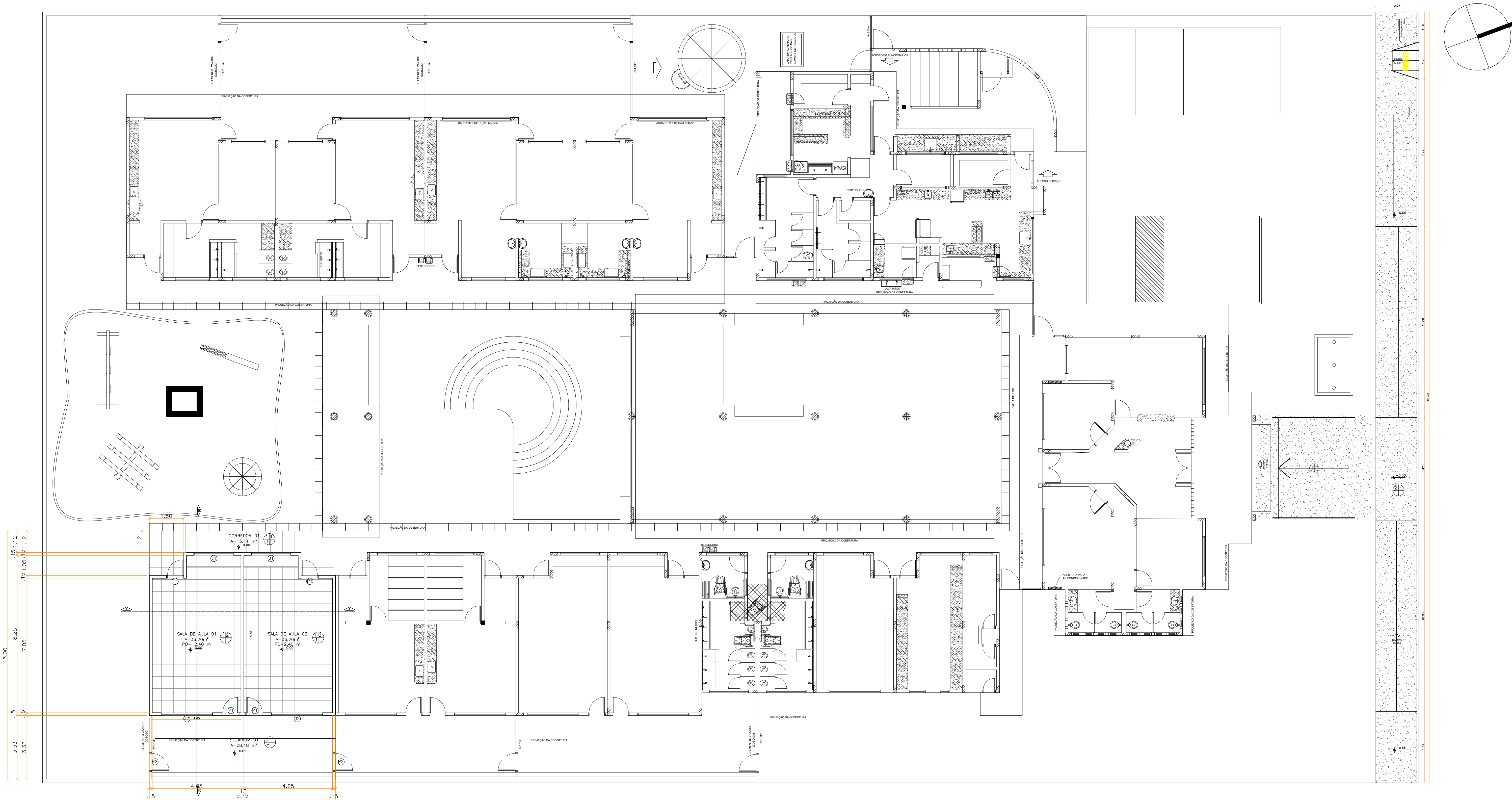
PLANTA BAIXA DE AMPLIAÇÃO esc 1:125
