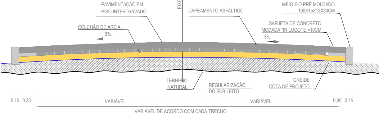
03 SEÇÃO TIPO
