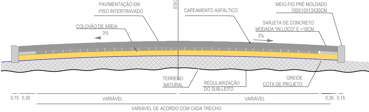
03 SEÇÃO TIPO
