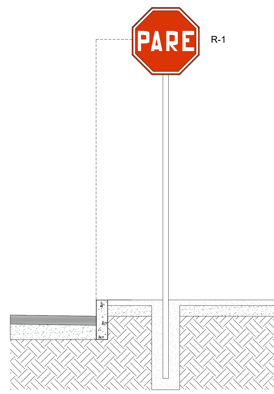
01 PLACA PARA PARADA OBRIGATÓRIA ESC.: 1/20
