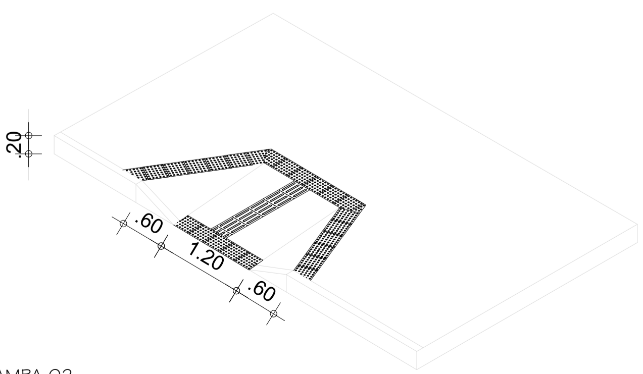
06 VISTA RAMPA 02 SEM ESCALA
