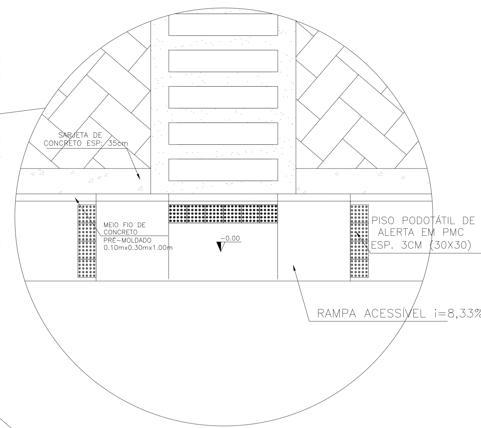
02 DET. RAMPA 01 SEM ESCALA
