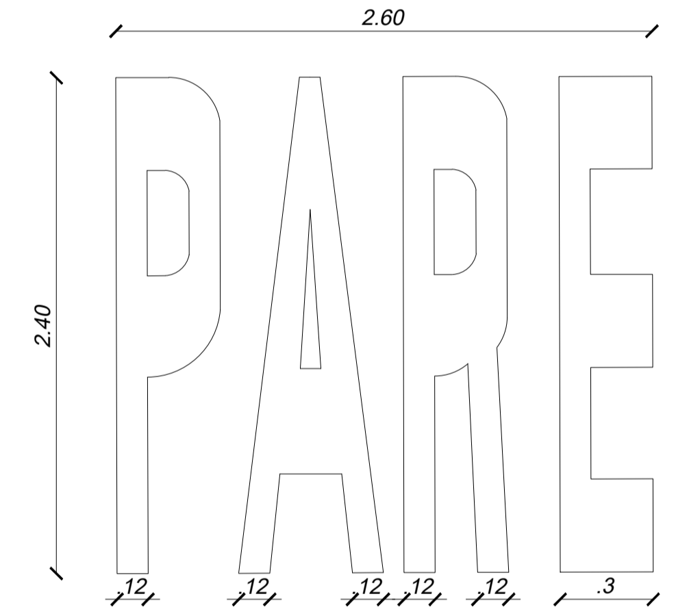
02 DET. LEGENDA NO SOLO 'PARE' SEM ESCALA
