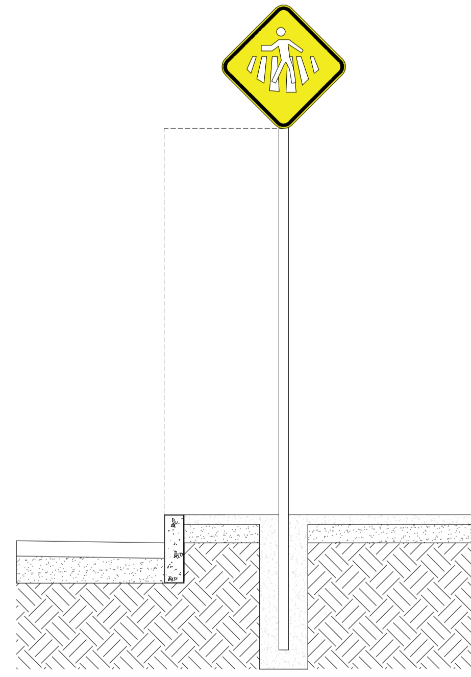
02 PASSAGEM SINALIZADA DE PEDESTRES ESC.: 1/20
