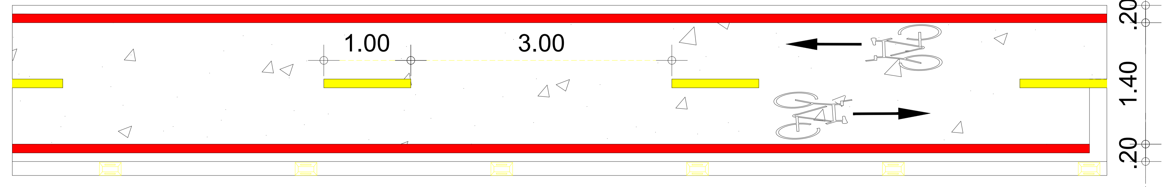
03 DETALHE DA CICLOVIA ESC.: 1/25
