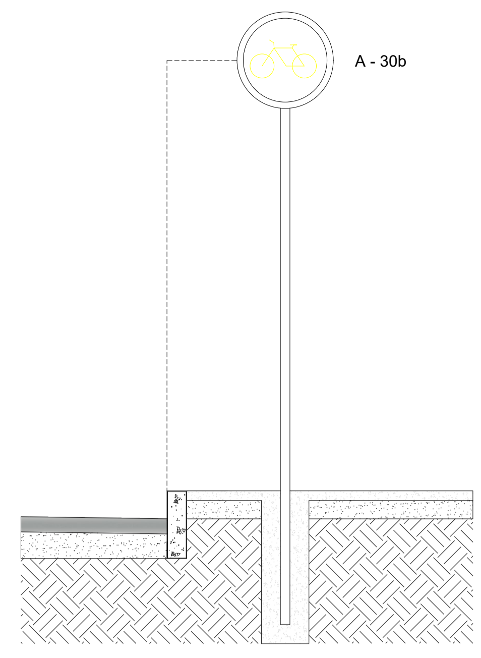
02 PLACA DE SINALIZAÇÃO PARA CICLISTAS ESC.: 1/20
