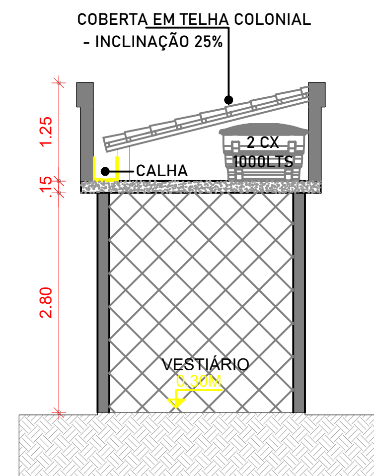
10 CORTE VEST. SEM ESCALA
