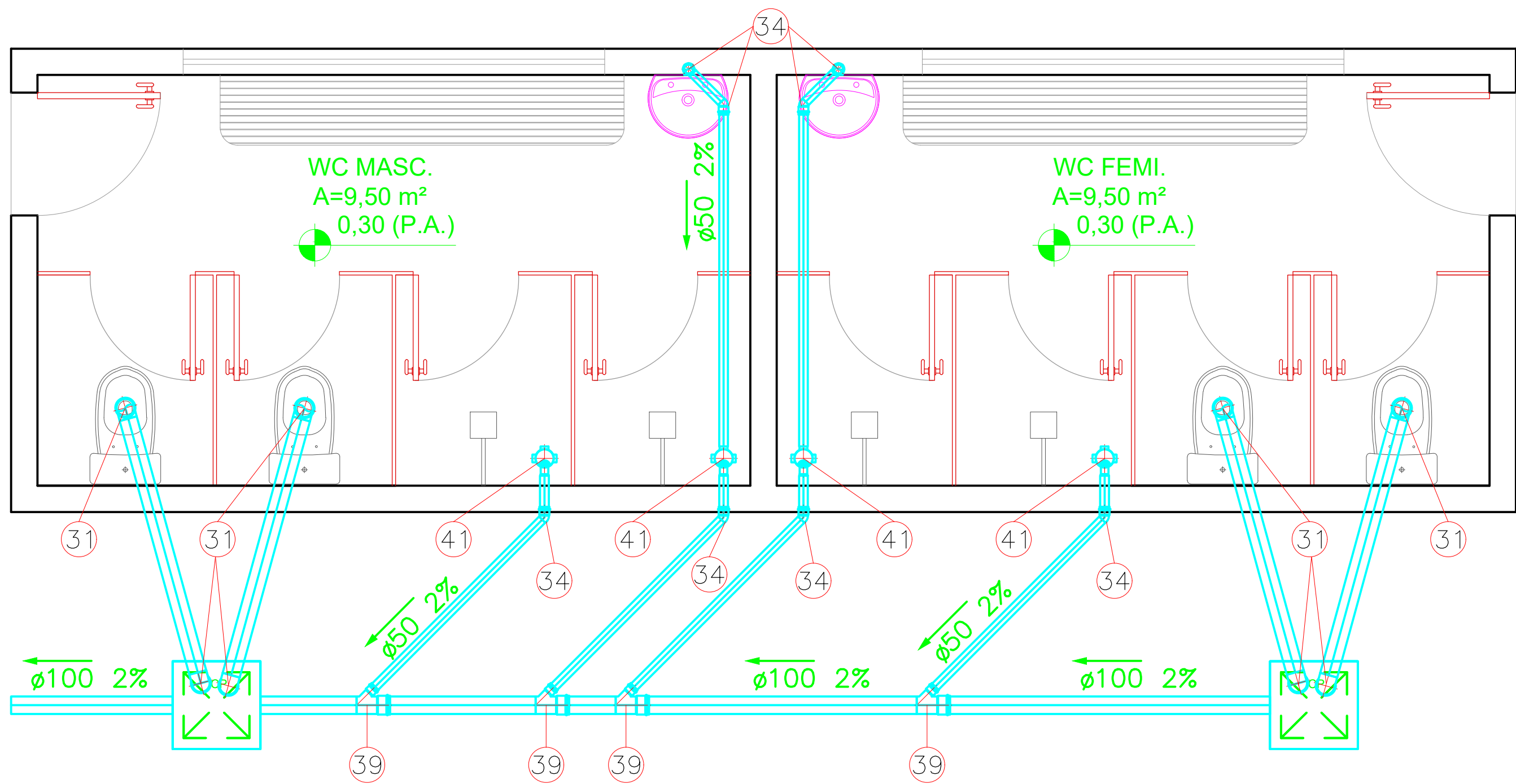
12 ESGOTO ESCALA 1/50
