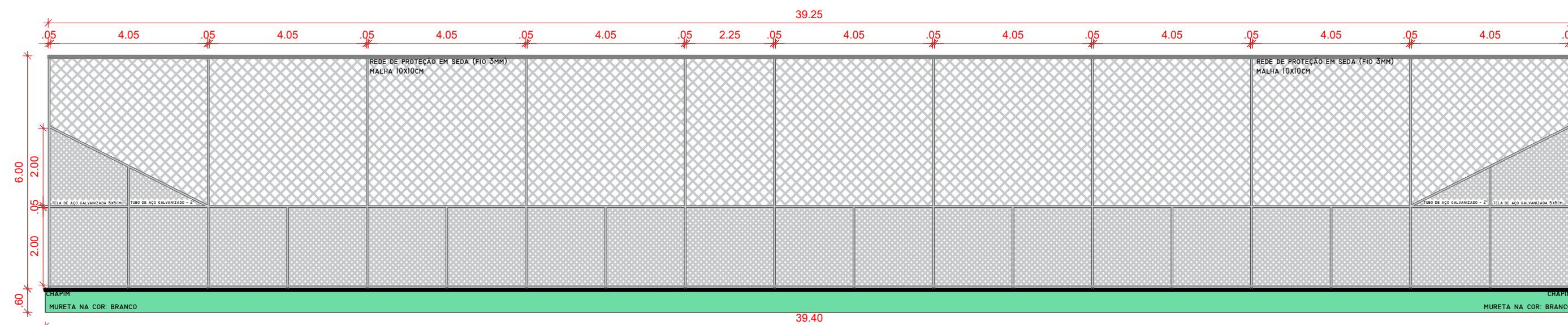
06 VISTA CC SEM ESCALA
