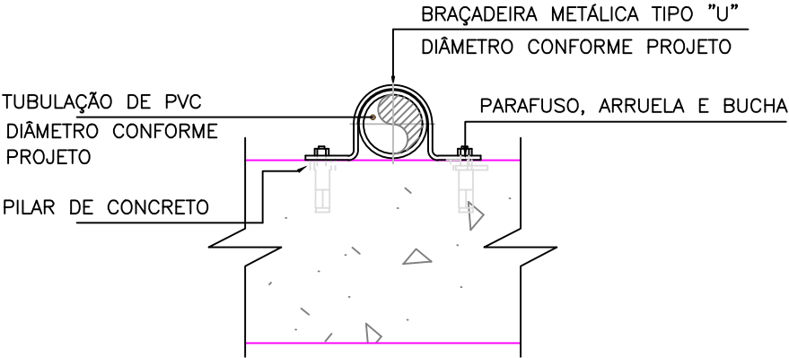
04 DETALHE DA FIXAÇÃO DE DESCIDAS SEM ESCALA
