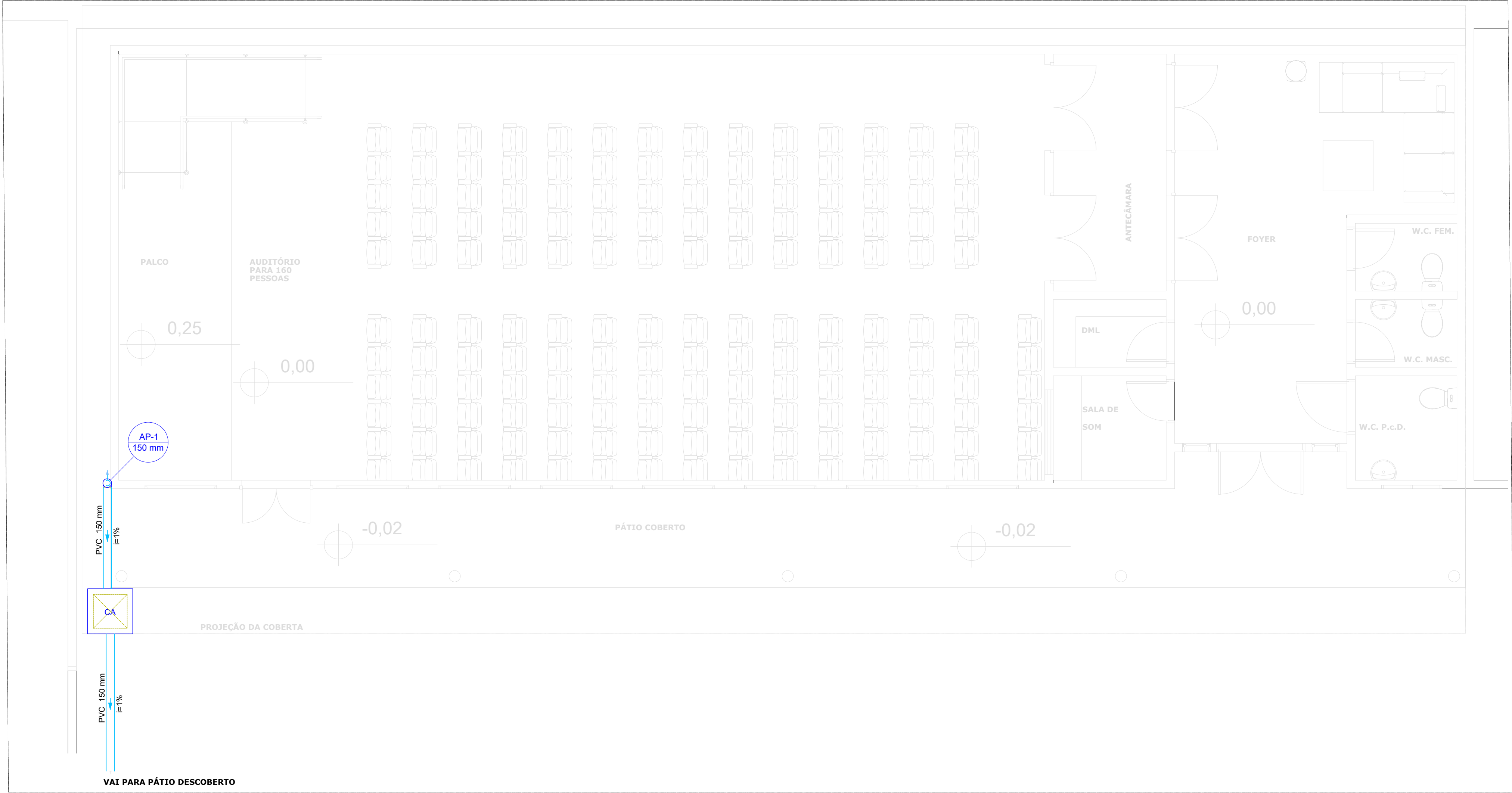
02 PLANTA BAIXA ESCALA 1/50
