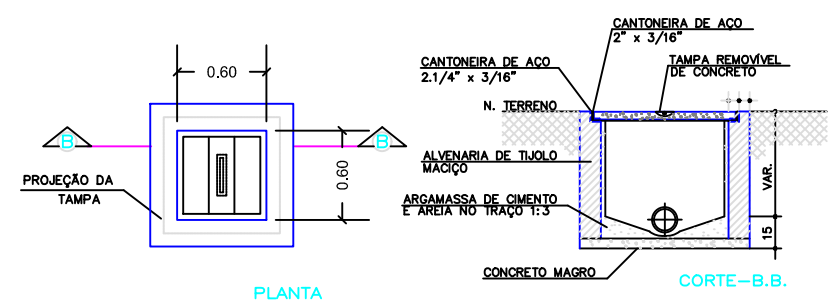
03 DETALHE DA CAIXA SEM ESCALA
