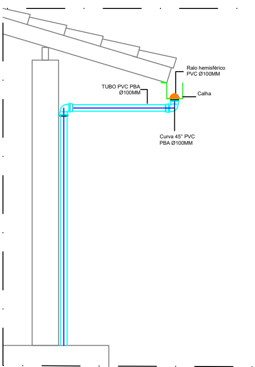
05 DETALHE DO RALO SEM ESCALA
