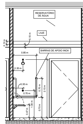
4 CC 04 1 : 25
