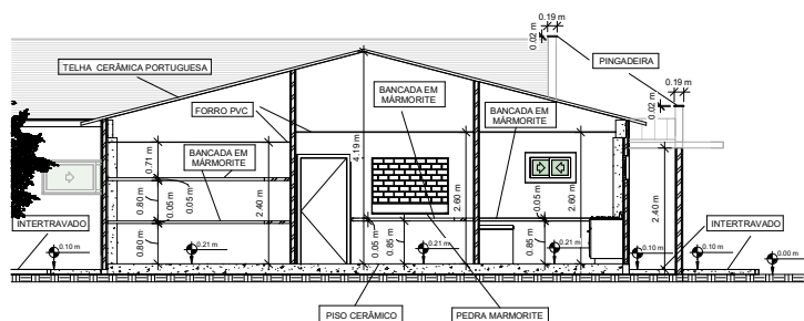
4 AA 04 1 : 50
