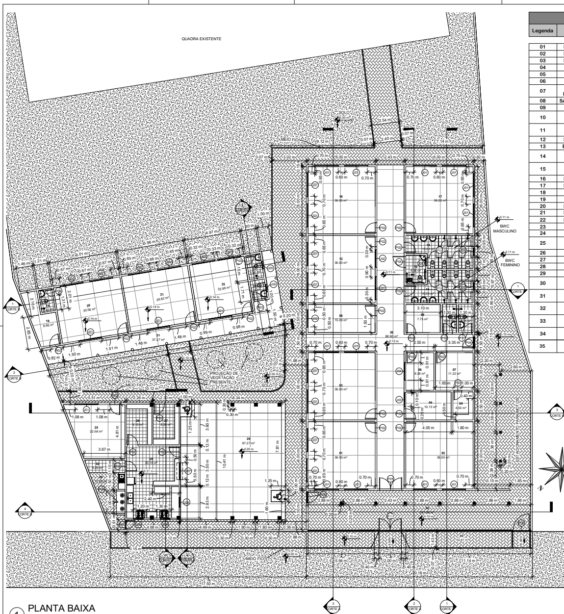
1 PLANTA BAIXA 1 : 100
