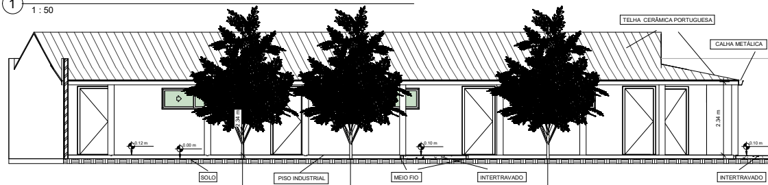
2 BB 02 1 : 50
