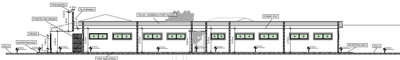
3 AA 03 1 : 75
