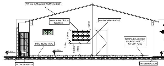
5 AA 05 1 : 50
