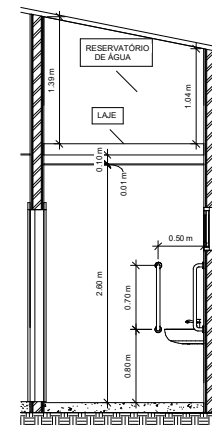
5 CC 05 1 : 25
