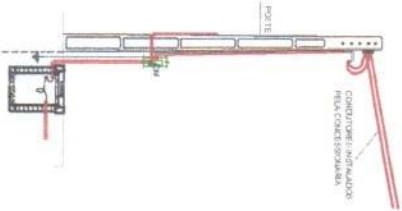
2 DETALHE POSTE esc 5/7E
