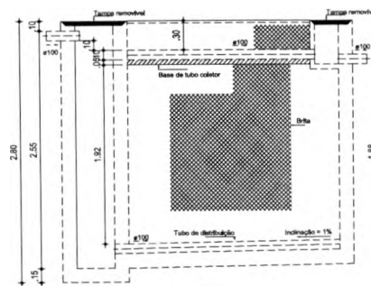
Filtro anaeróbio Corte 1 - ESC. 1:25
