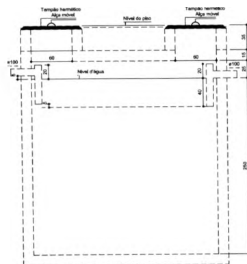
Tanque séptico Corte 1 - ESC. 1:25
