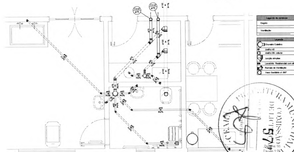
Detalhe S5 Escala 1:25
