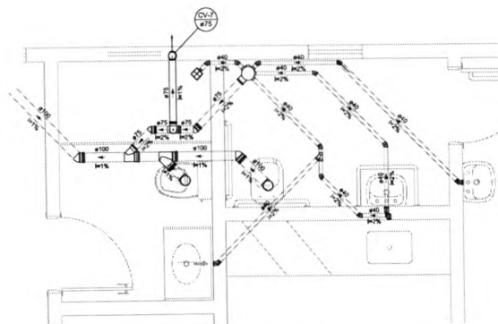
Detalhe S4 Escala 1:25
