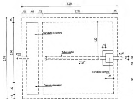
Filtro anaeróbio Planta baixa - ESC. 1:25
