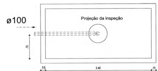
Sumidouro Planta baixa - ESC. 1:25
