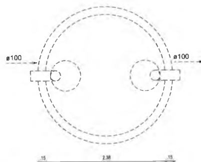
Tanque séptico Planta baixa - ESC. 1:25
