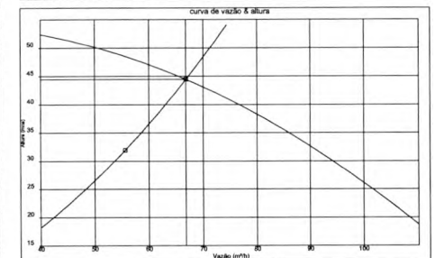
Curvas características de bomba hidráulica BC-23 R/F 2 - 15 CV 15
