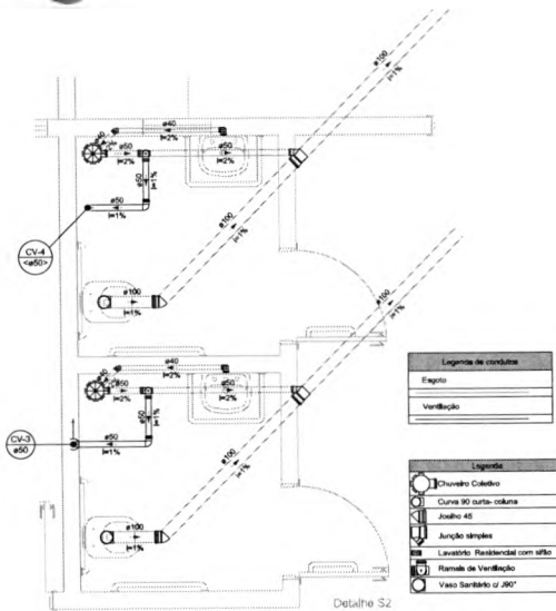
Detalhe S2 Escala 1:25
