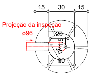
04 SUMIDOURO - PLANTA BAIXA ESCALA 1/25
