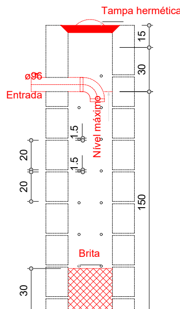
04 SUMIDOURO - CORTE ESCALA 1/25
