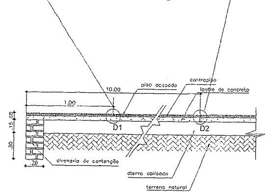
② CORTE AA Escala: SEM
