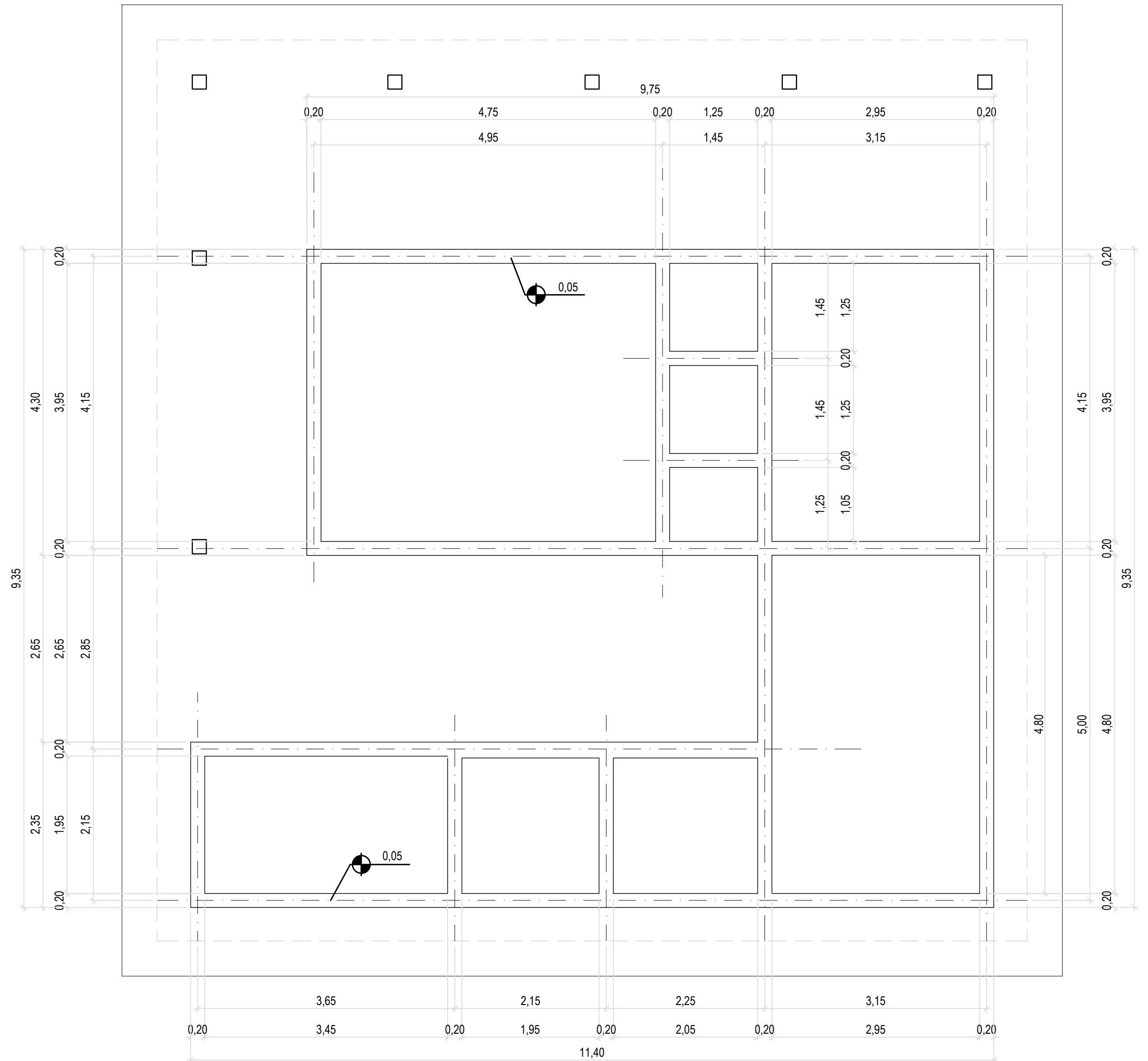
PLANTA DE LOCAÇÃO DAS VIGAS BALDRAME ESC. 1:50
