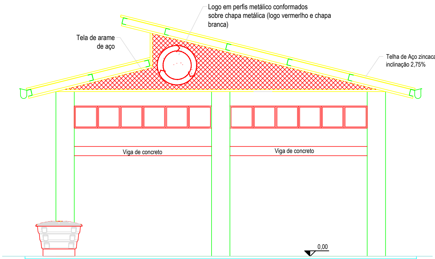
VISTA 2 ESC. 1:50
