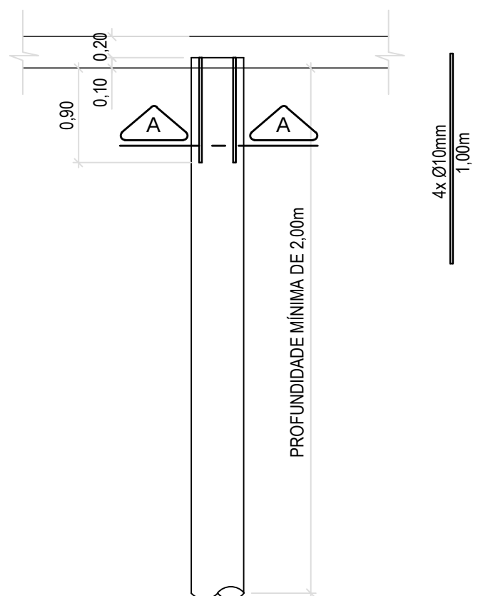
ARMAÇÃO DAS BROCAS ESC. 1:20
