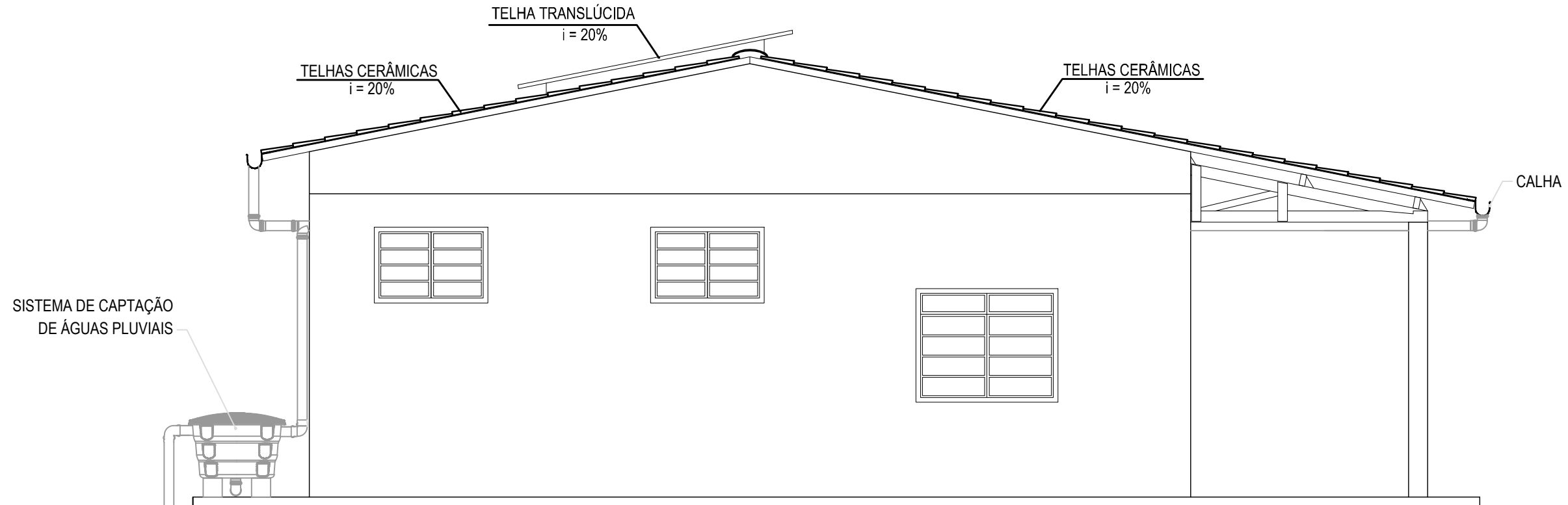
VISTA - 1 ESC. 1:50
