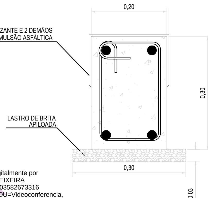
SEÇÃO TÍPICA DA VIGA BALDRAME ESC. 1:5
