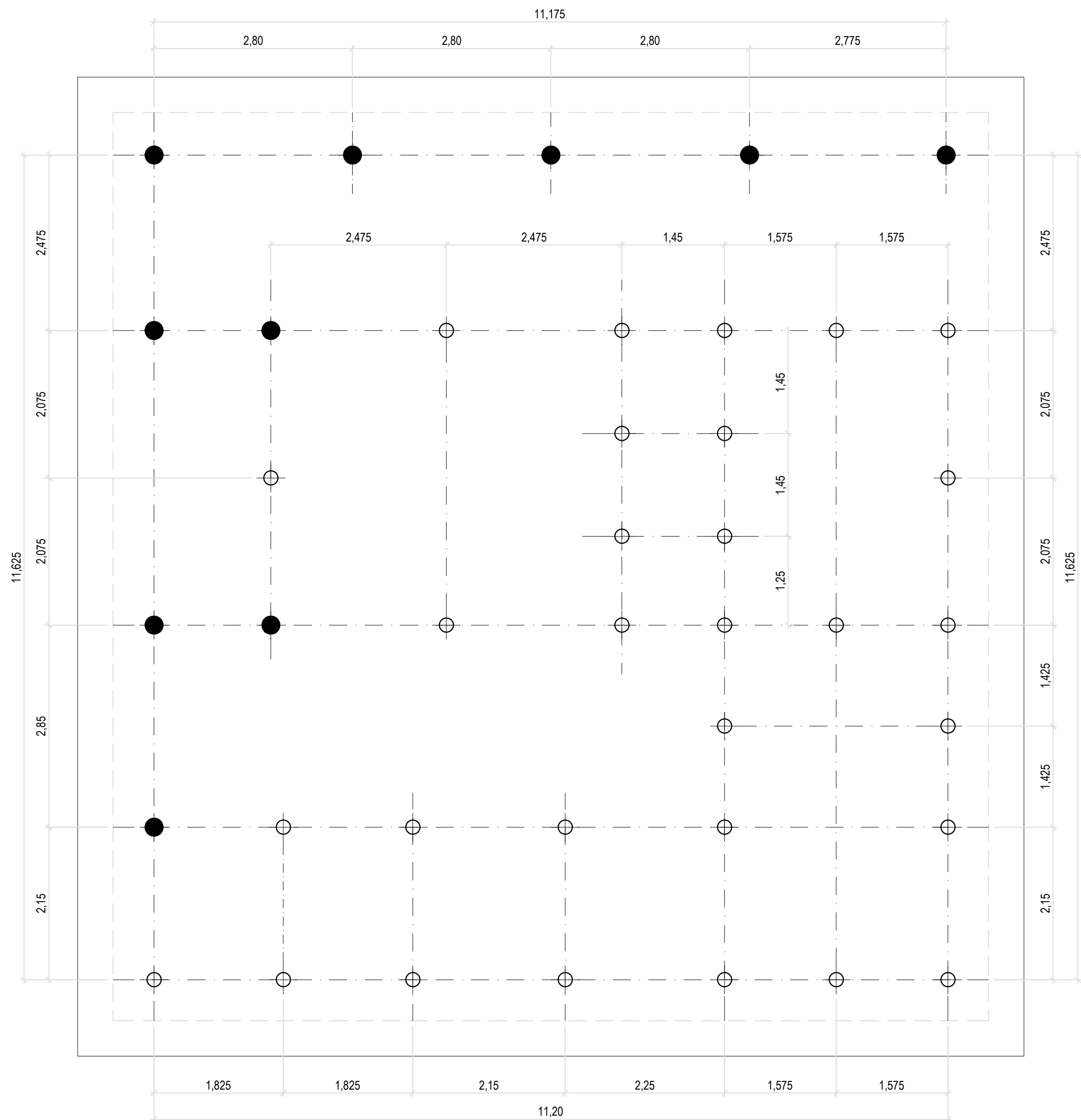
PLANTA DE LOCAÇÃO DAS BROCAS ESC. 1:50
