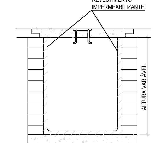
CAIXA DE INSPEÇÃO - CORTE (REDE DE ESGOTO SANITÁRIO) ESC. 1:10
