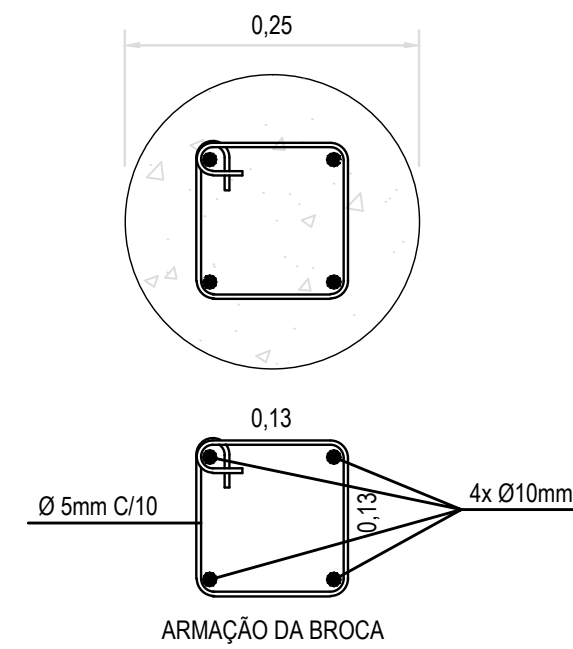
CORTE A-A BROCA A TRADO S/ESC.
