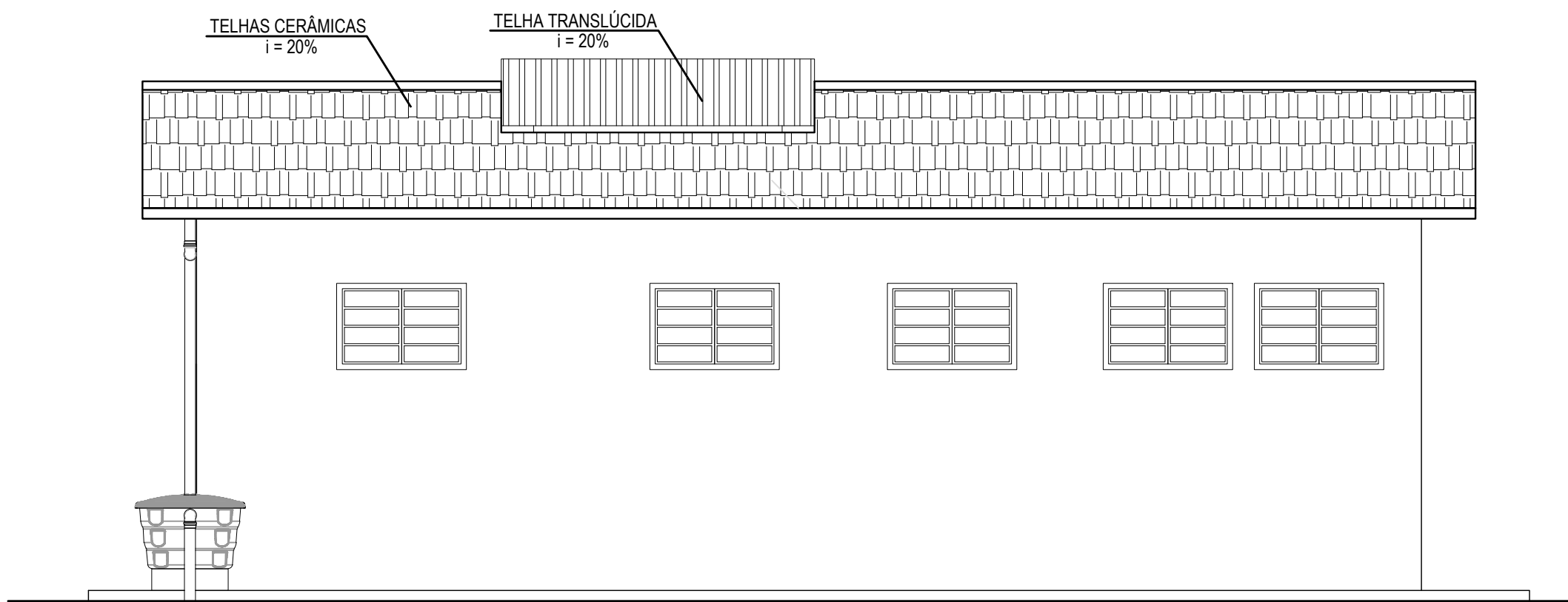
VISTA - 1 ESC. 1:50
