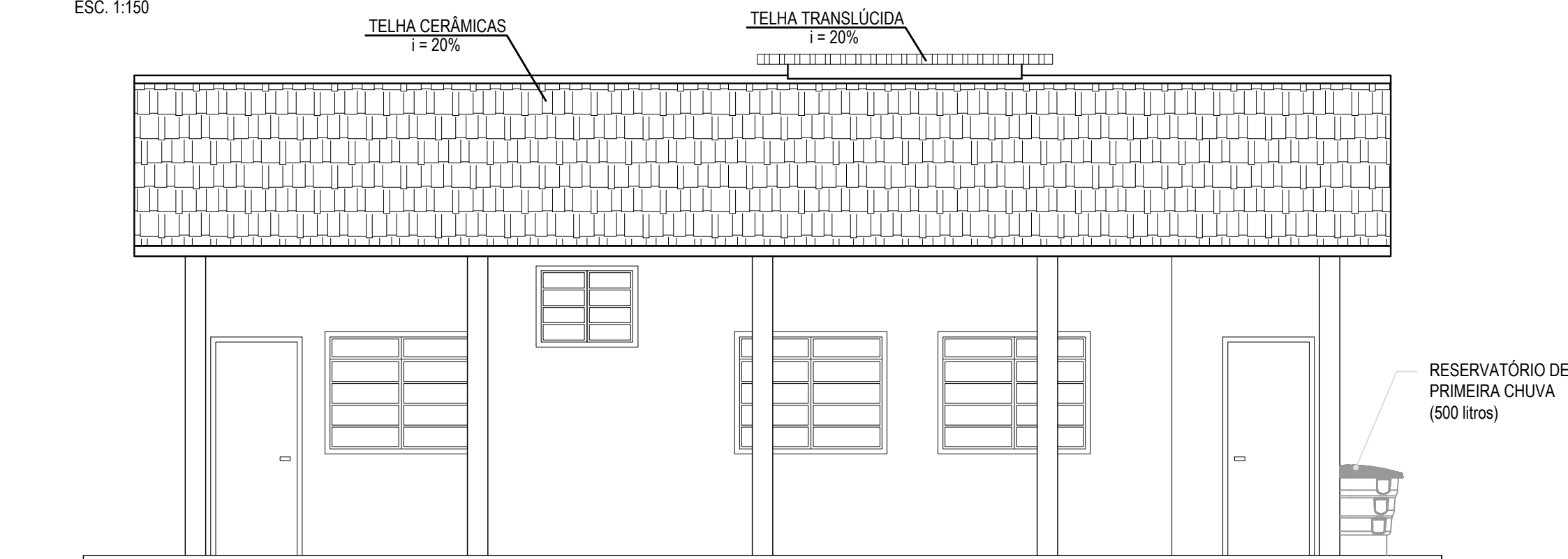
VISTA - 4 ESC. 1:50
