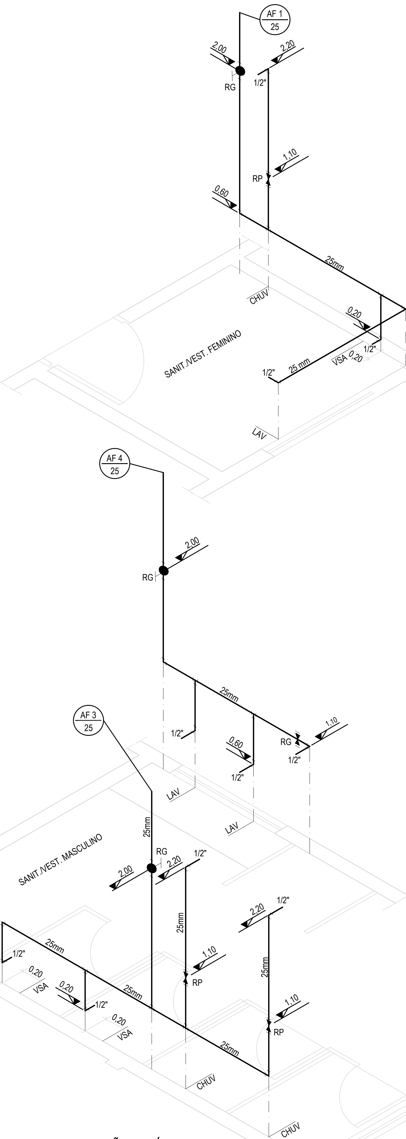
PERSPECTIVAS - INSTALAÇÃO DE ÁGUA ESC. 1:20
