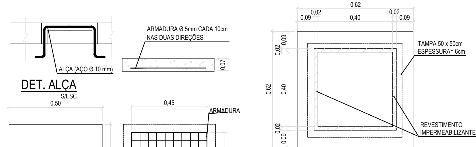
DET. ALÇA S/ESC. TAMPA DA CAIXA DE INSPEÇÃO ESC. 1:10
