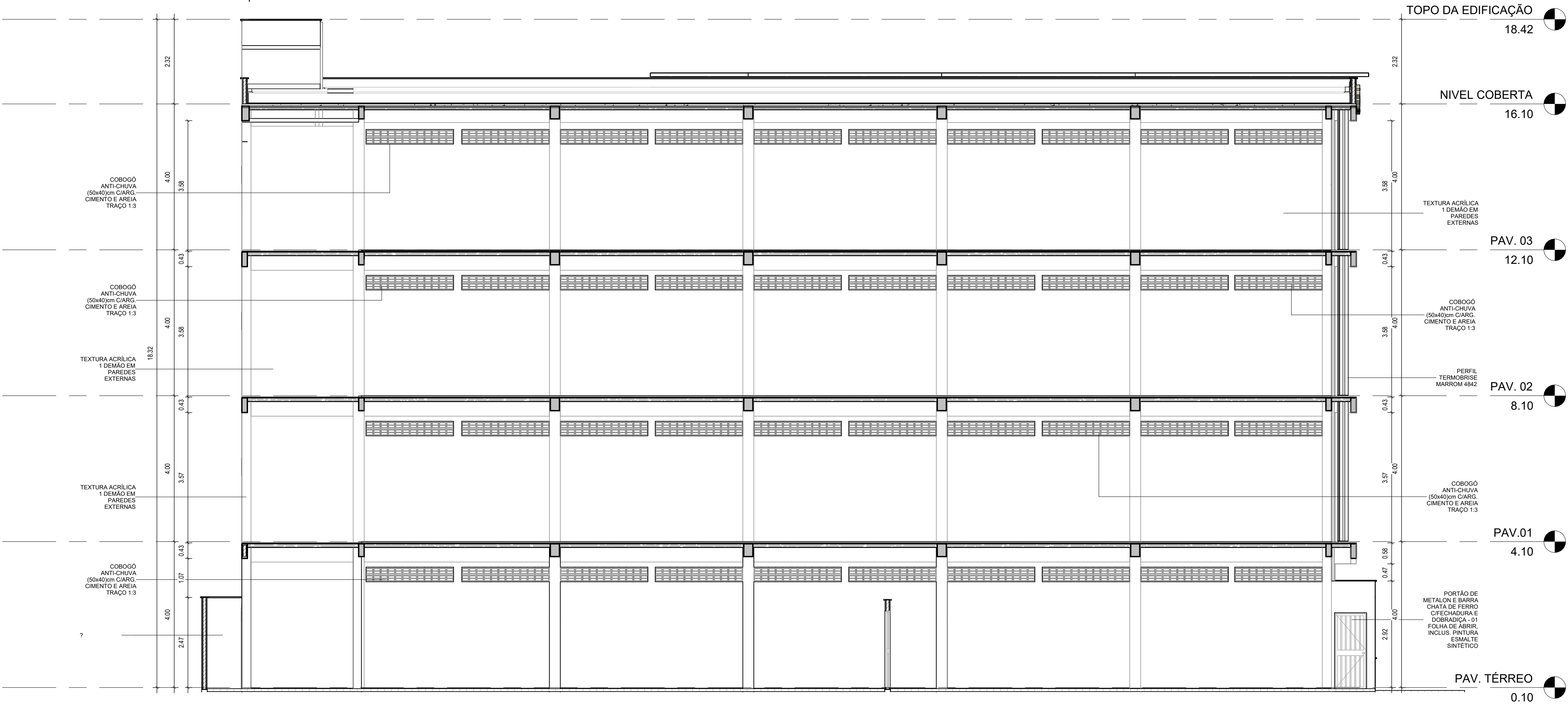
1 VISTA - E3 1:75
