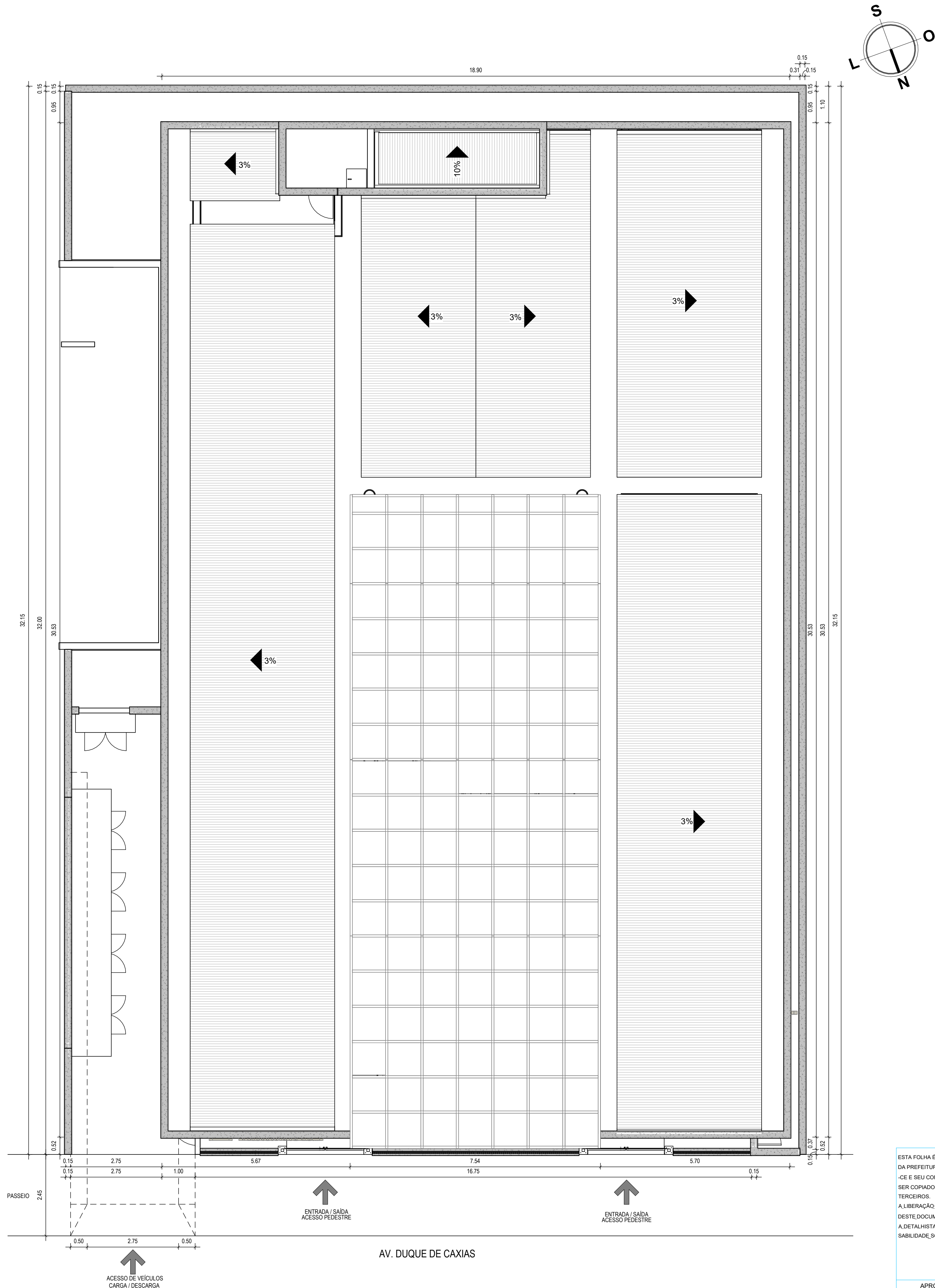
3 | IMPLANTAÇÃO 1 : 75
