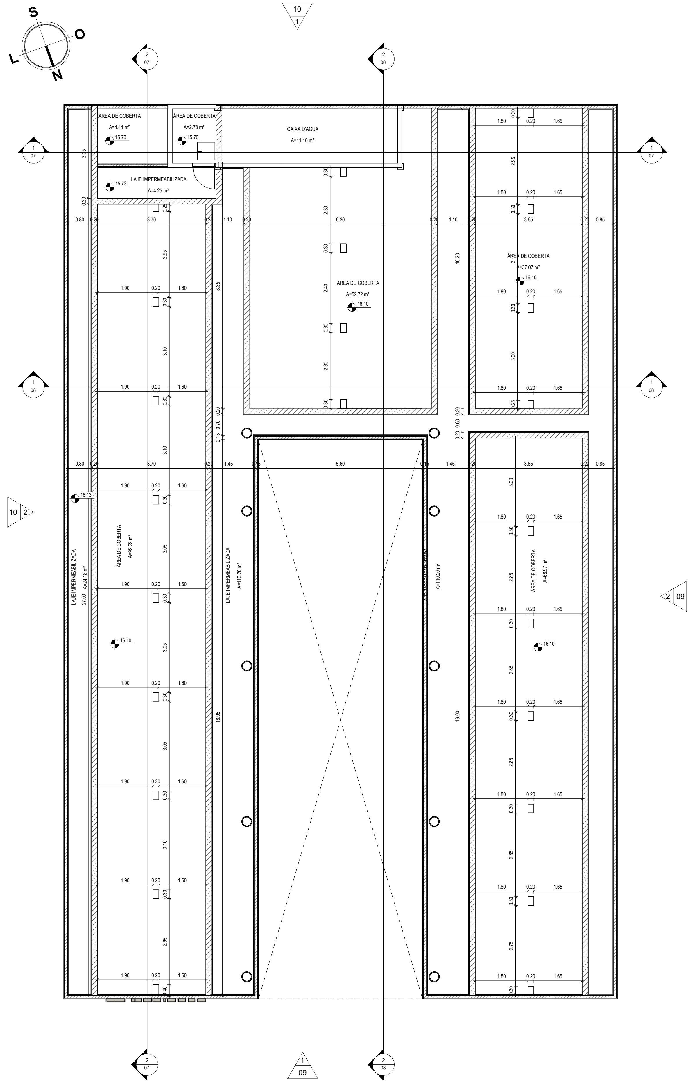
2 | PL. COBERTA - LAJE EMERMEABILIZADA 1:75
