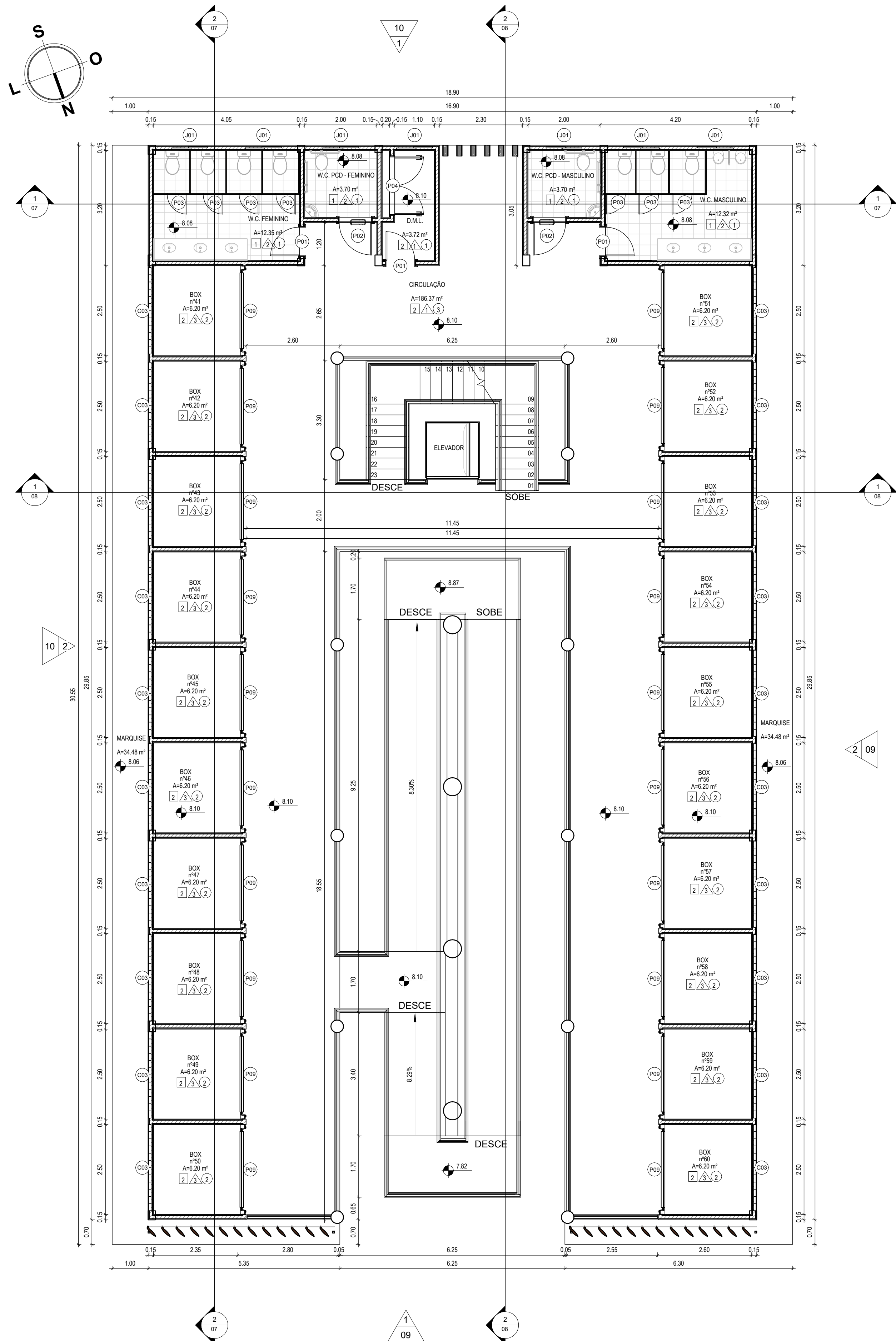
1 PL. BAIXA PAV 02 1 : 75
