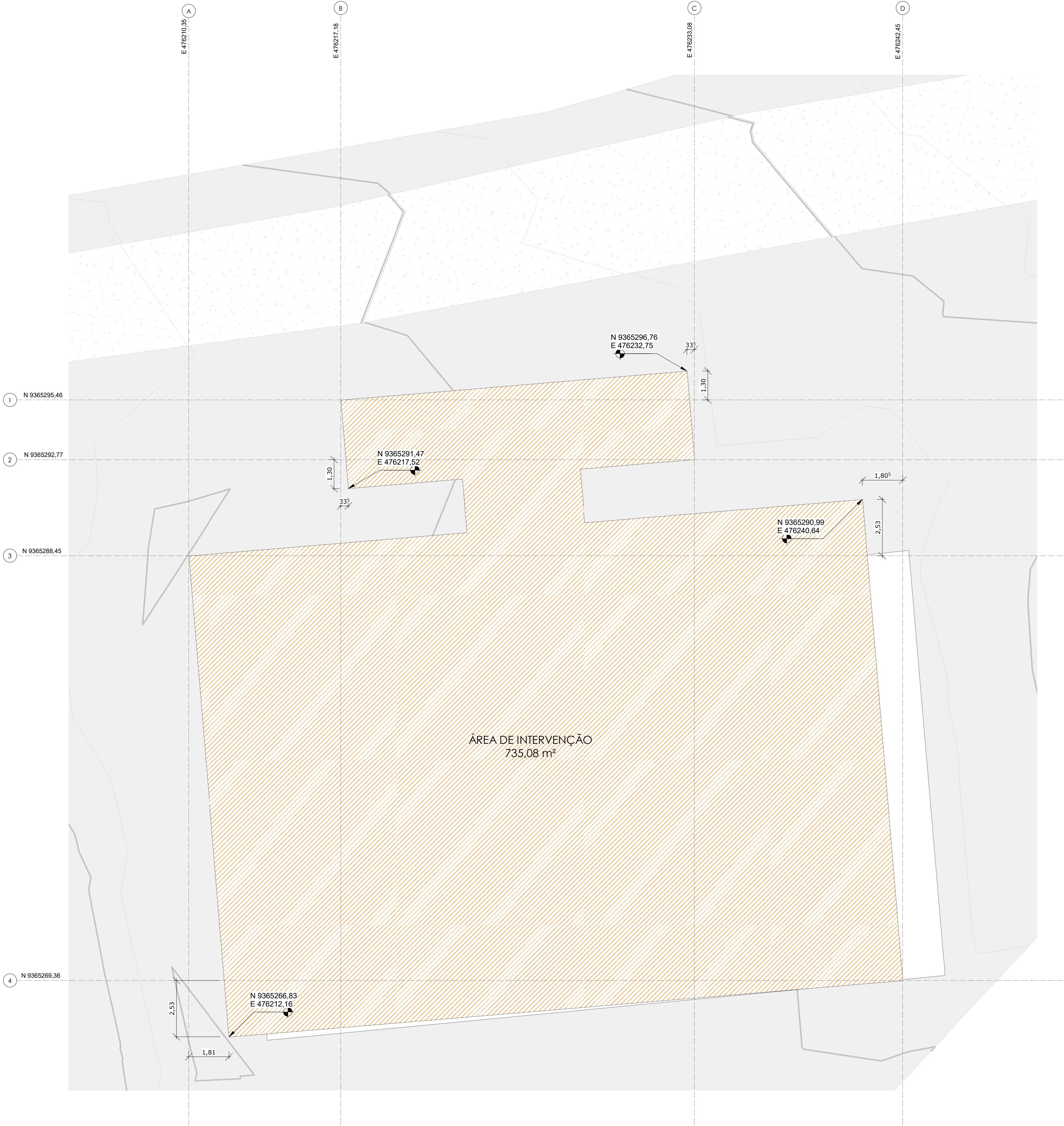
1 | LOCALIZAÇÃO 1:100
