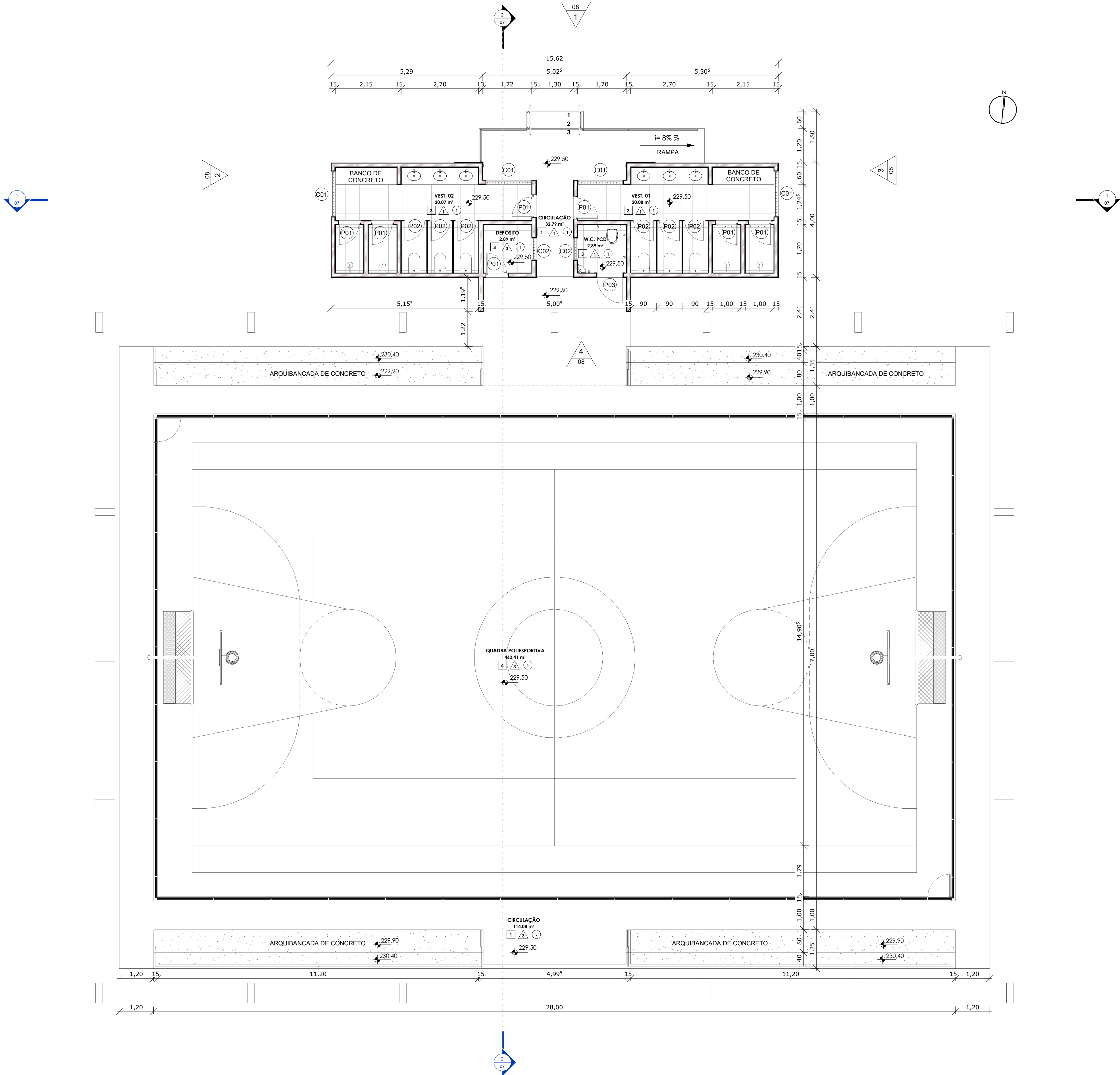
1 | PLANTA BAIXA 1:75
