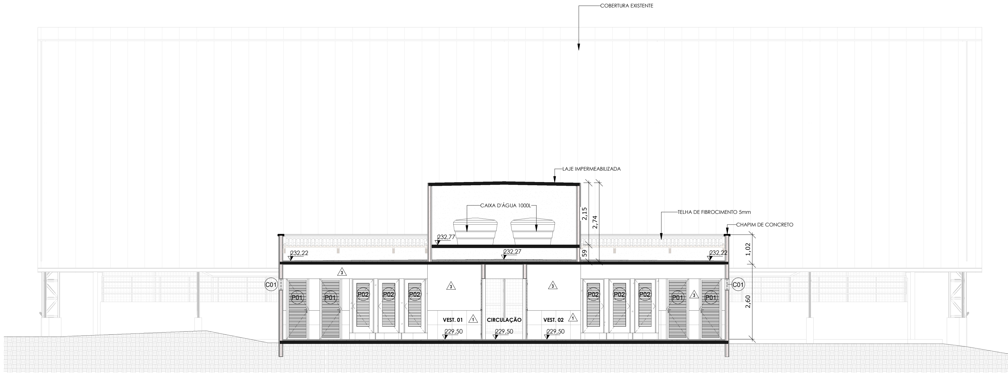
1 | CORTE 01 1:75
