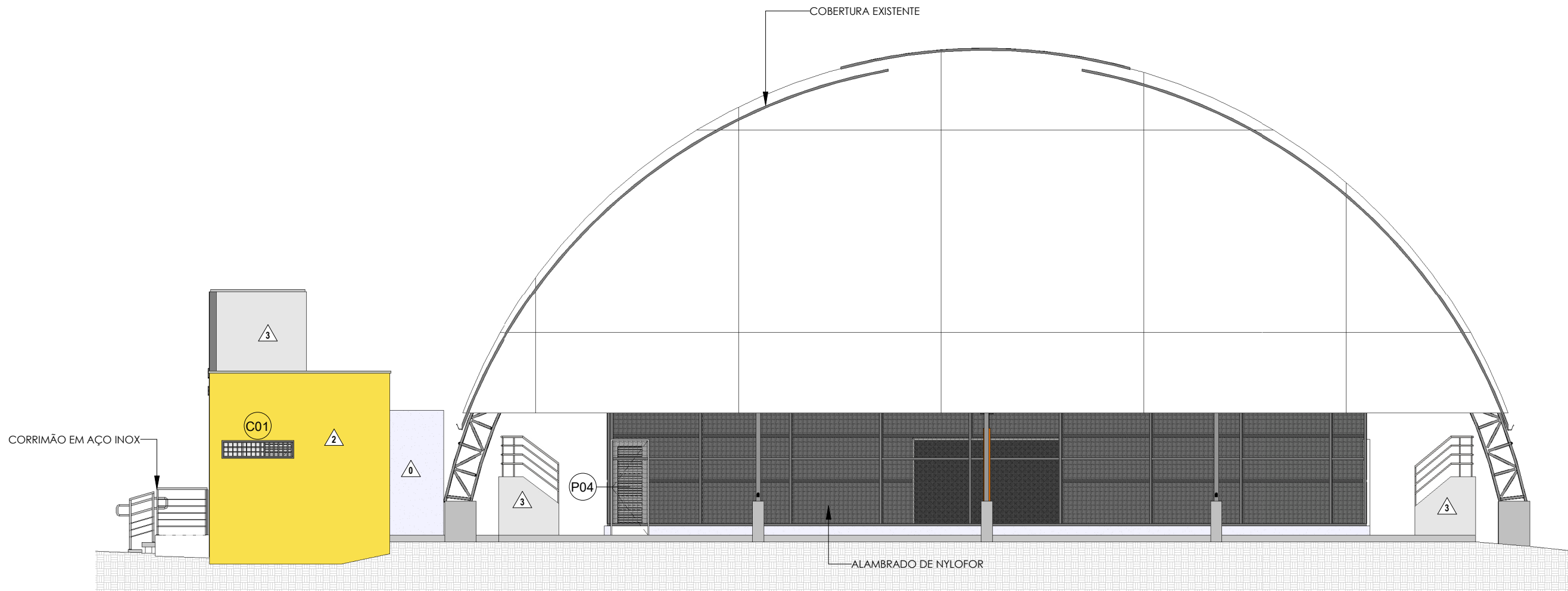
2 FACHADA LATERAL 1 1 : 100
