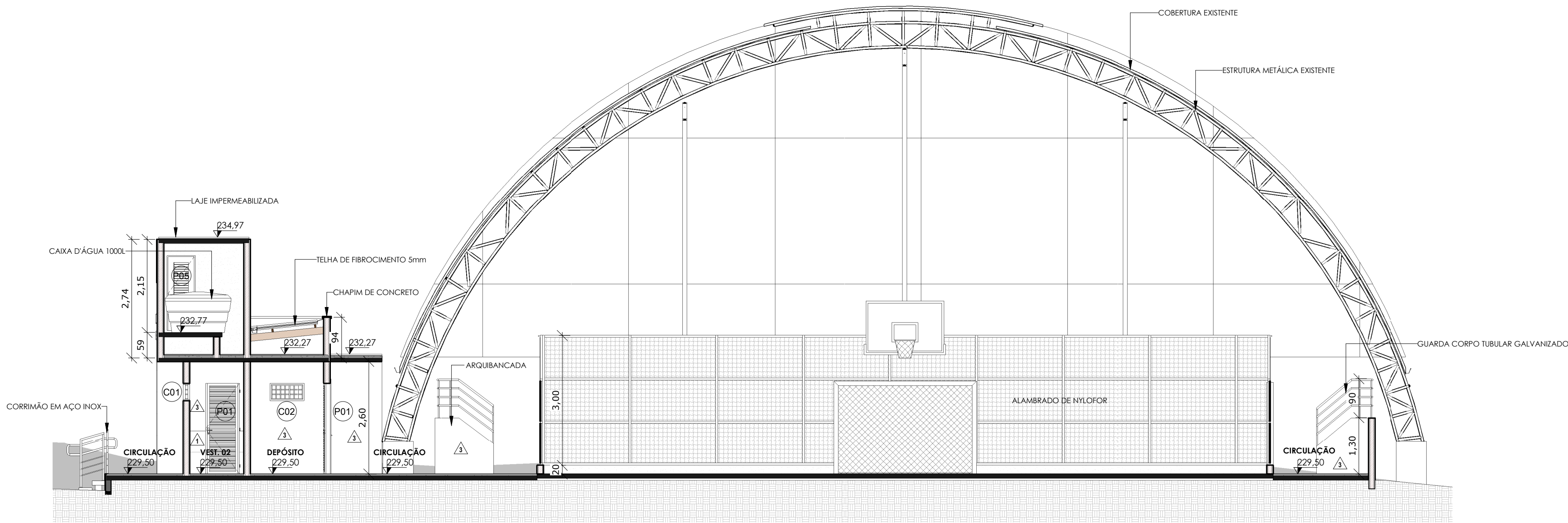
2 | CORTE 02 1:75
