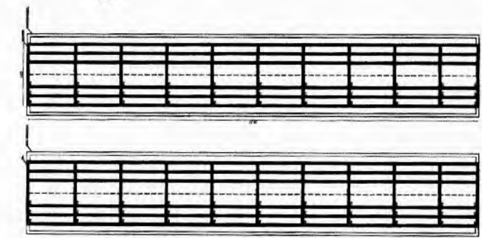
03 SEÇÃO DOS PILARES - ESTRIBO SEM ESCALA
