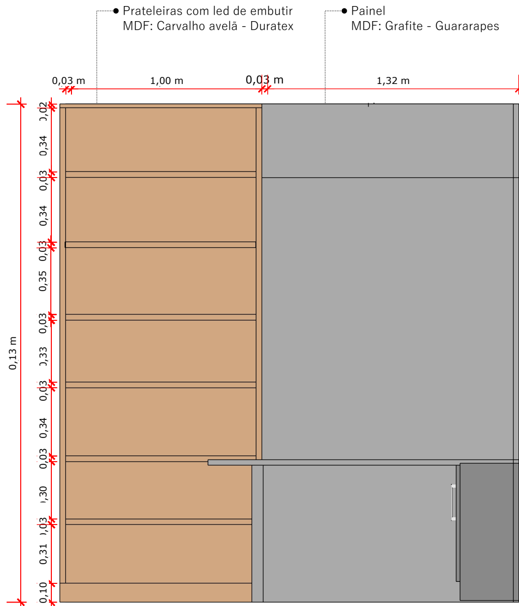
VISTA FRONTAL ESCALA: 1:20
