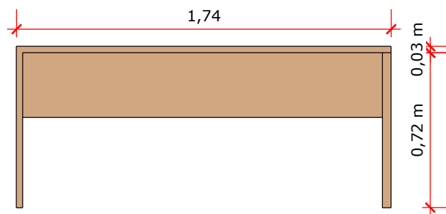
MESA 01
