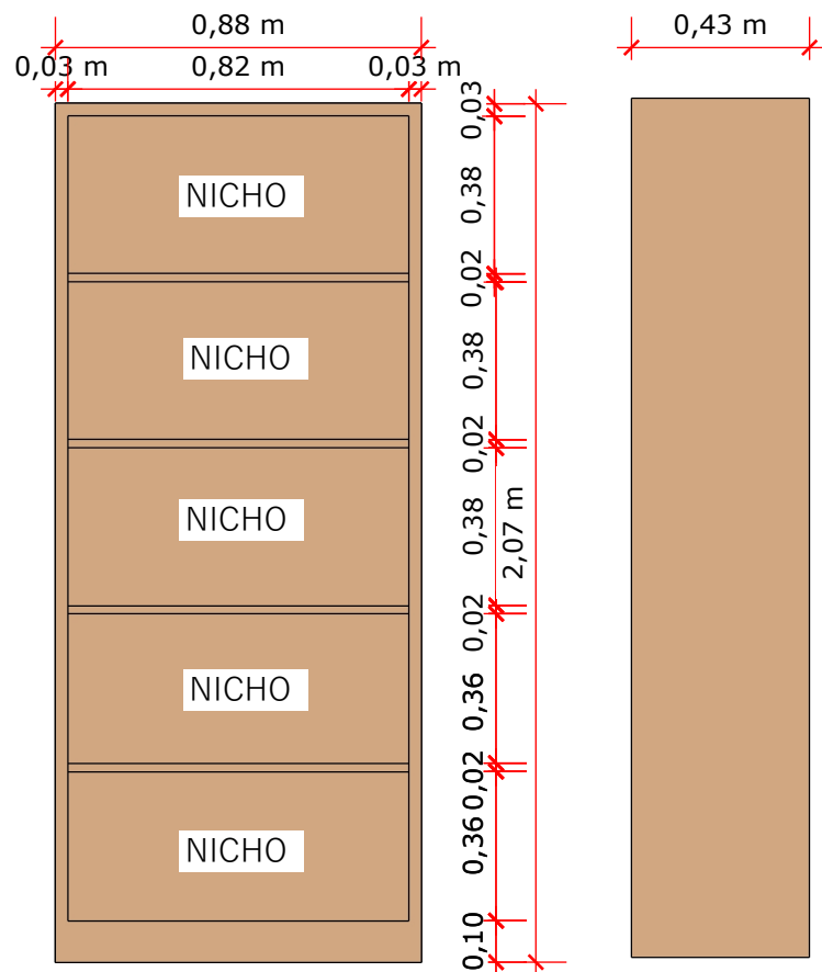
PRATELEIRA VISTA FRONTAL E VISTA LATERAL
