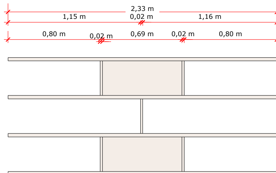
PRATELEIRAS VISTA FRONTAL
