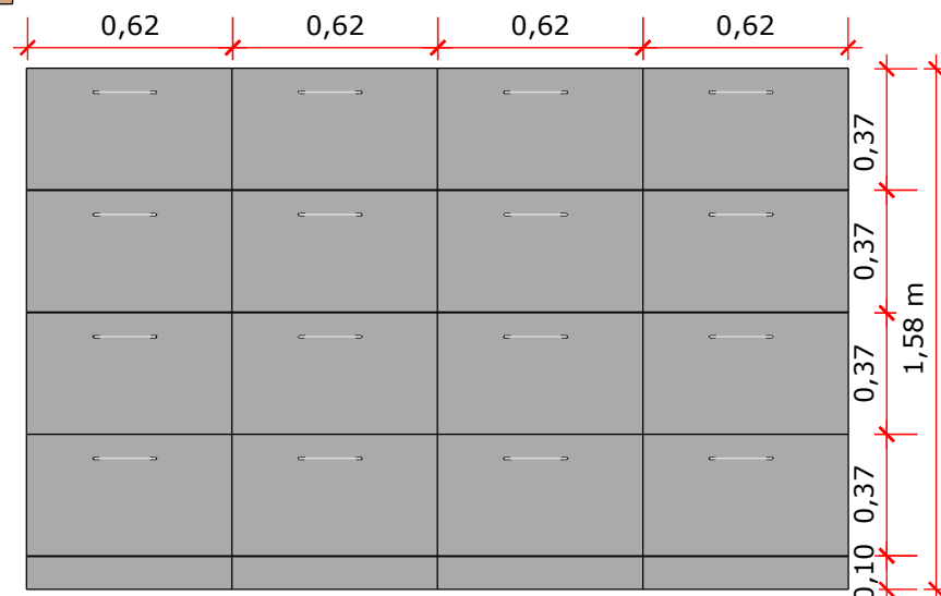
GAVETEIRO
