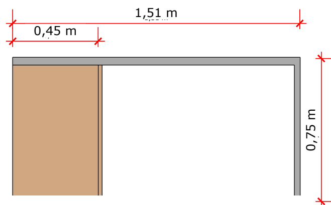
ARMÁRIO INF. VISTA FRONTAL
