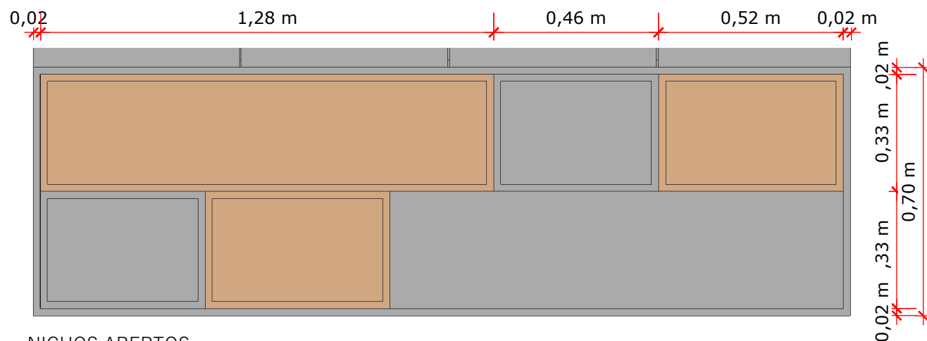
NICHOS ABERTOS
