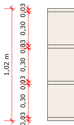
PRAT. LATERAL
