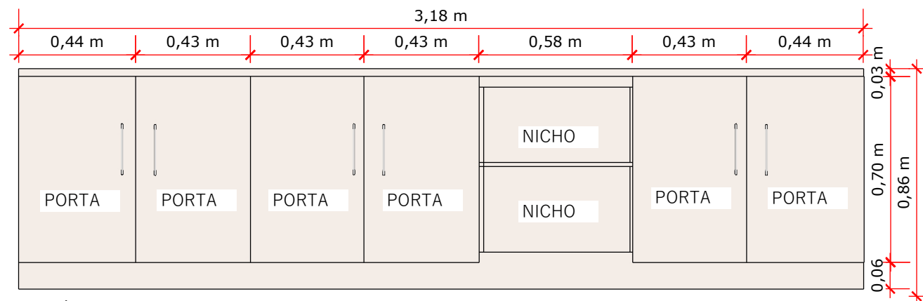
ARMÁRIO INFERIOR
