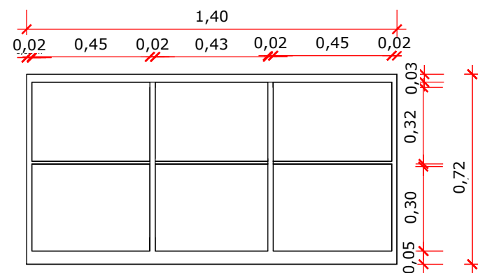
ARMÁRIO INF. VISTA INTERNA
