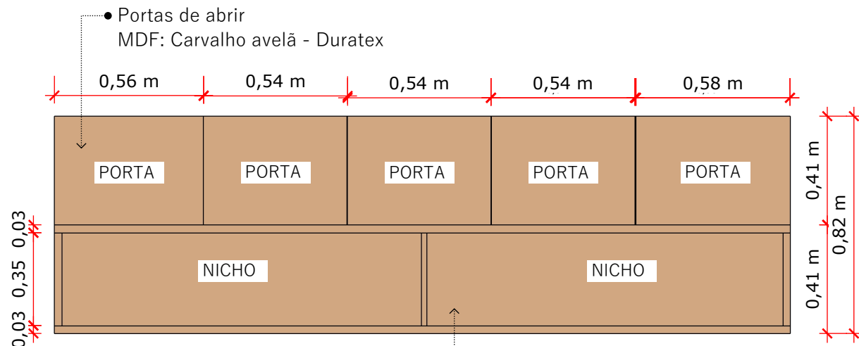
ARMÁRIO SUPERIOR COM NICHOS
