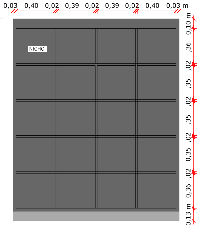
ARMÁRIO INTERNO
