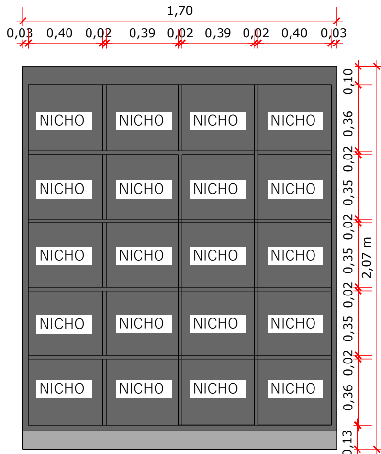
ARMÁRIO SUPERIOR ABERTO
