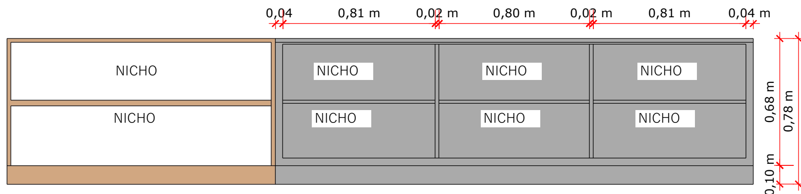
BANCADA INFERIOR ABERTO
