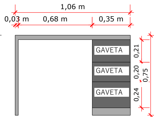
MESA - VISTA 02
