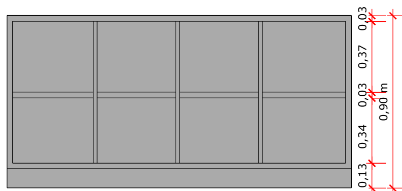
ARMÁRIO ABERTO
