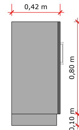
ARMÁRIO - VISTA LATERAL
