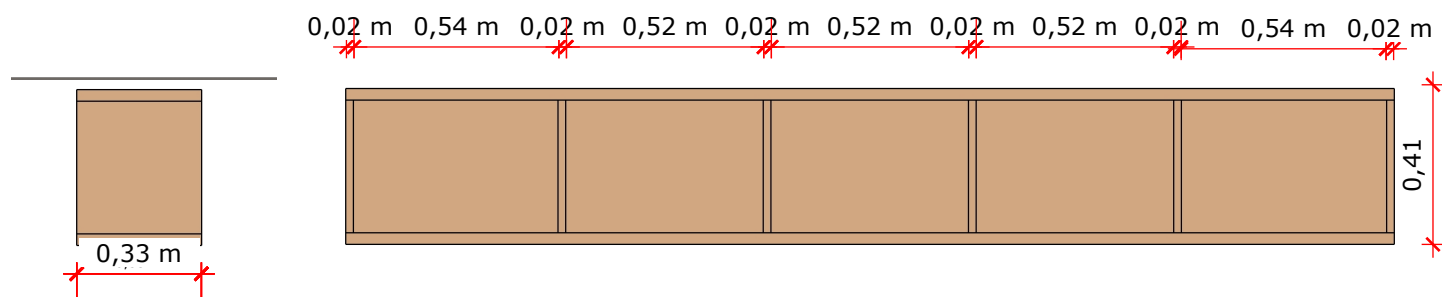
DETALHES DO ARMÁRIO SUPERIOR
