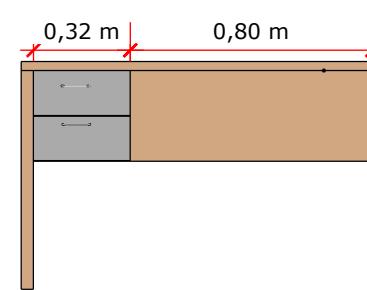
MESA 02 - VISTA INTERNA
