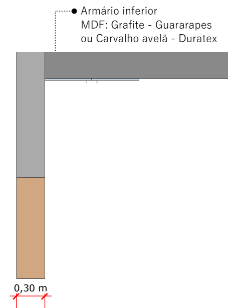
VISTA SUPERIOR
