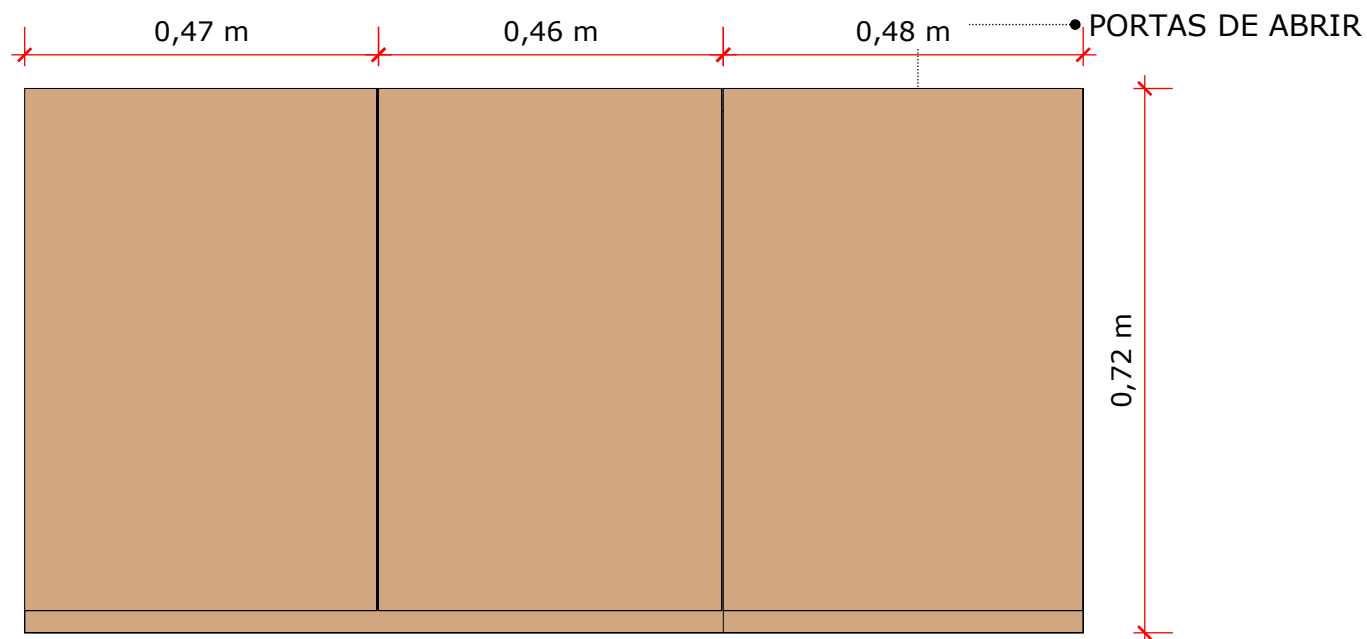
ARMÁRIO INFERIOR
