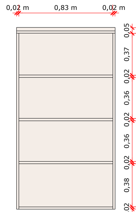
ARMÁRIO ABERTO
