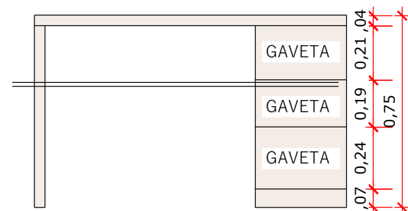
VISTA INTERNA
