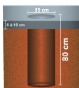
CHUMBADOR TIPO CADEIRINHA
