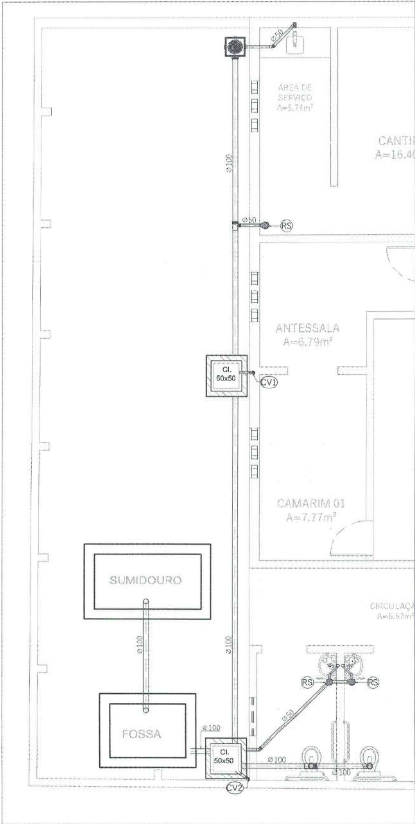
SANITÁRIO - PLANTA BAIXA esc: 1:50
