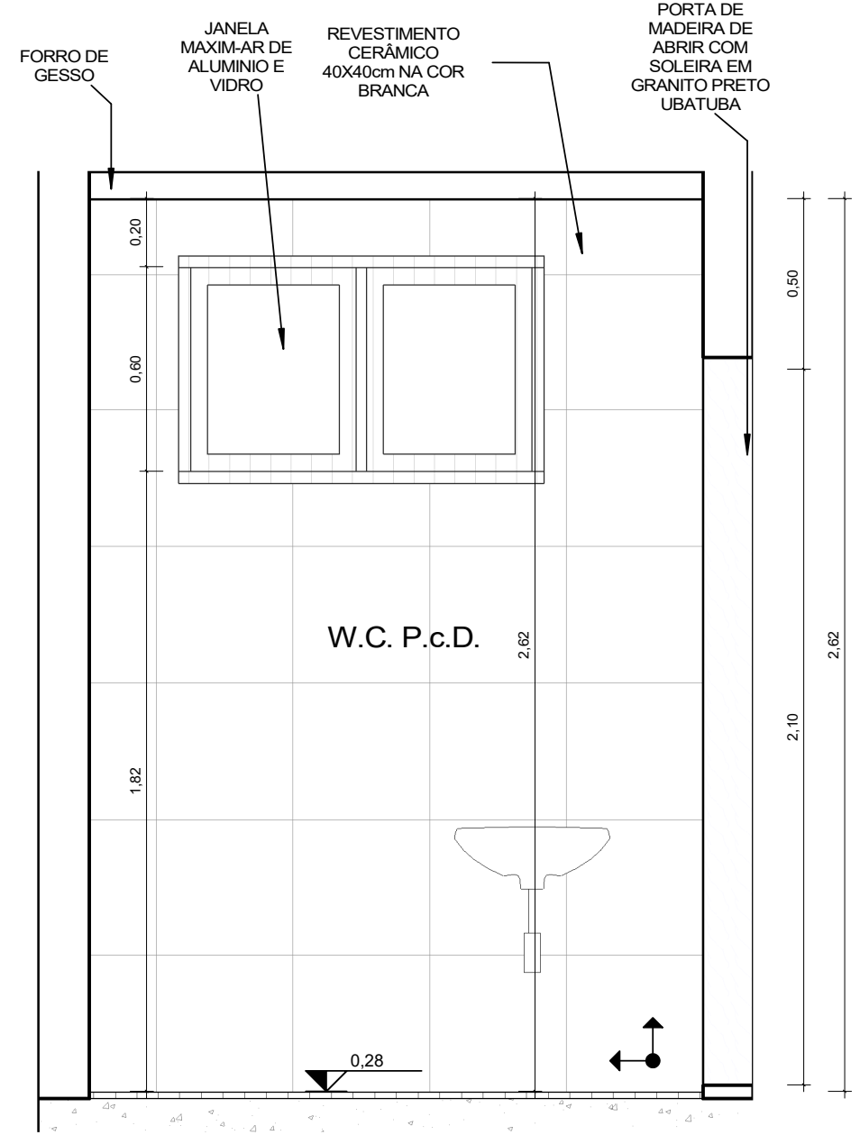
4 | VISTA 04 - W.C. P.c.D. 1 : 20
