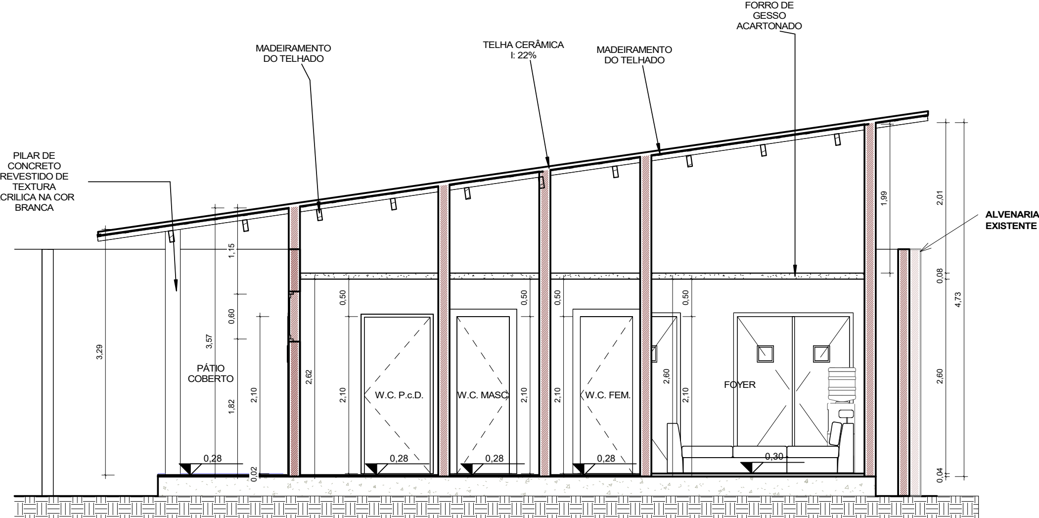
2 | CORTE BB 1 : 50
