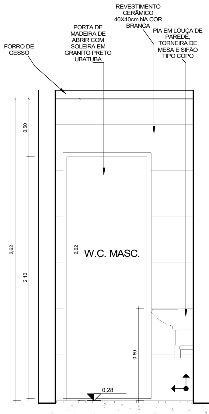
1 | VISTA 01 - W.C. MASC. 1 : 20
