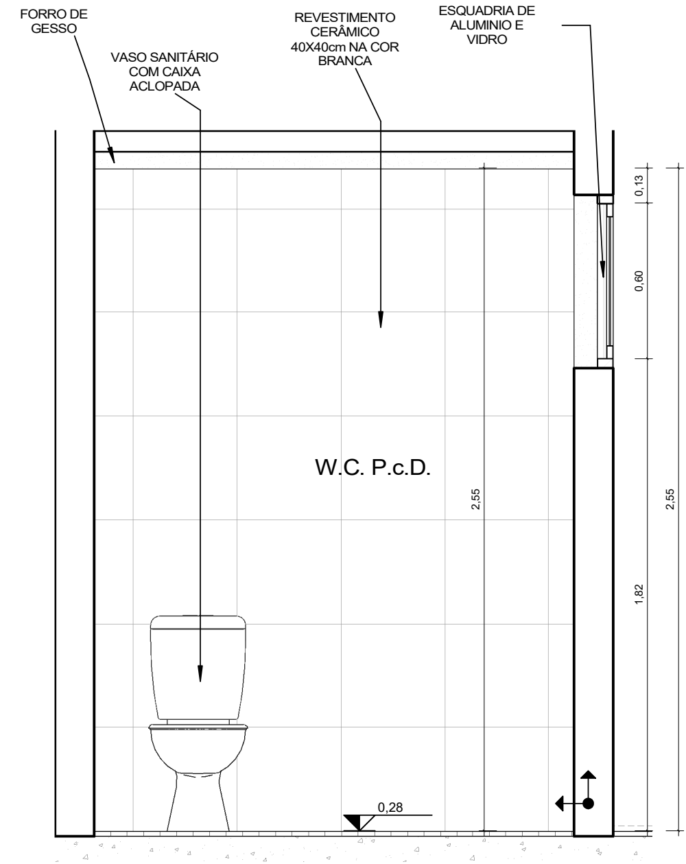
5 | VISTA 05 - W.C. P.c.D. 1 : 20
