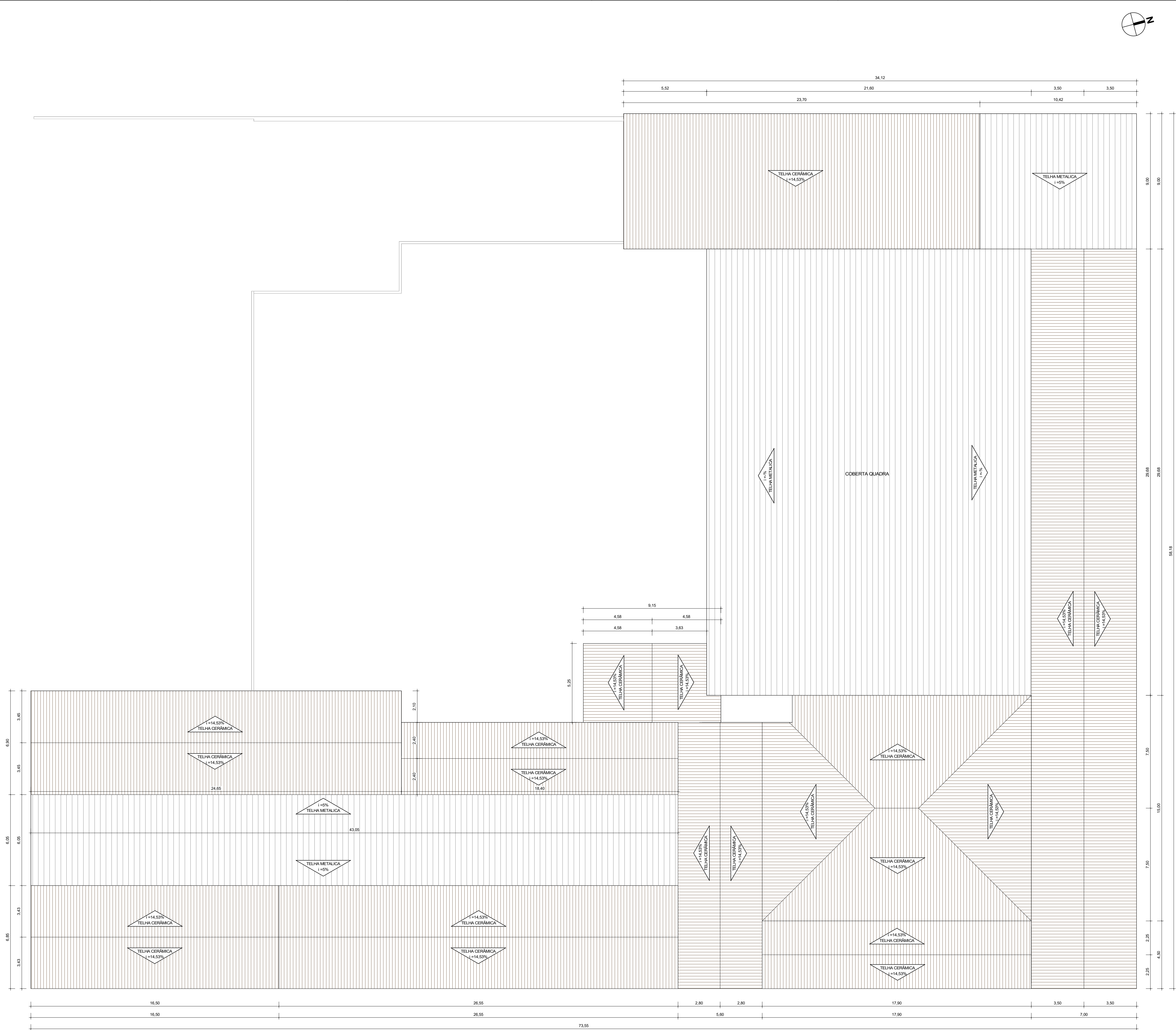
1 | PLANTA DE COBERTA EXISTENTE 1 : 125
