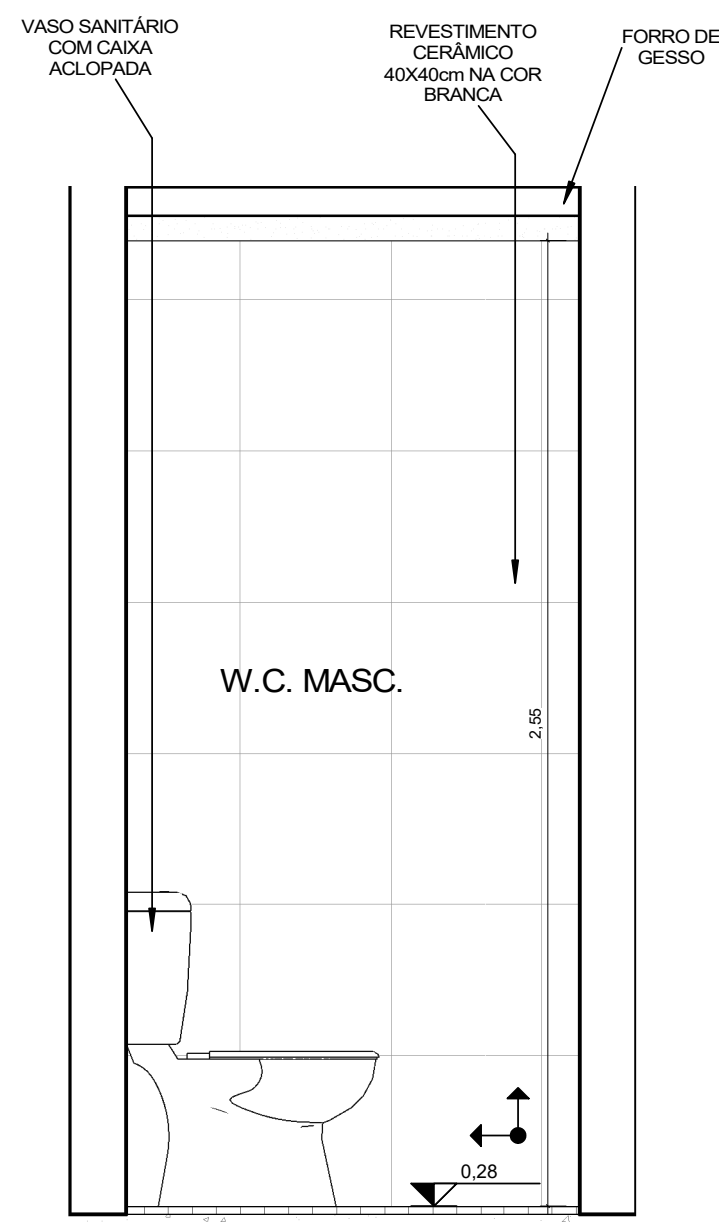
3 | VISTA 03 - W.C. MASC. 1 : 20
