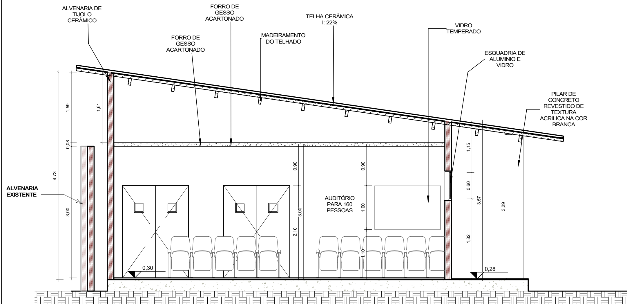
1 | CORTE AA 1 : 50
