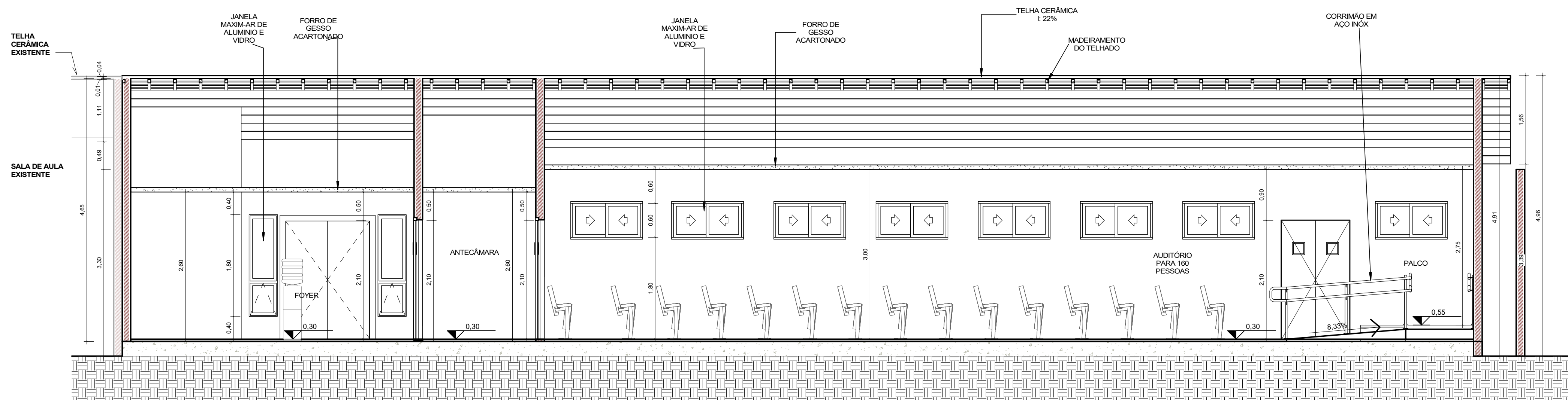
3 | CORTE CC 1 : 50
