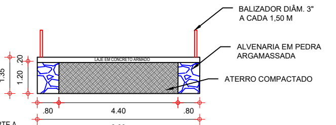
06 CORTE A ESCALA 1/50
