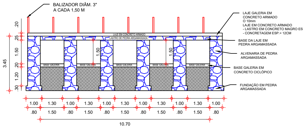
05 CORTE B ESCALA 1/50
