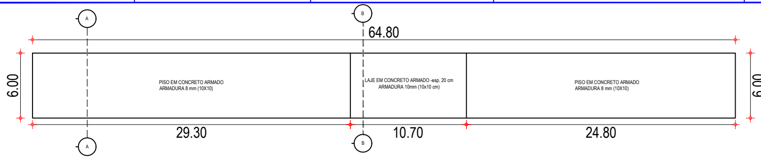
01 PLANTA BAIXA 01 ESCALA 1/125
