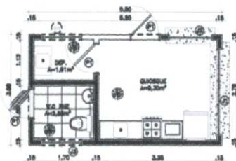
PLANTA BAIXA
