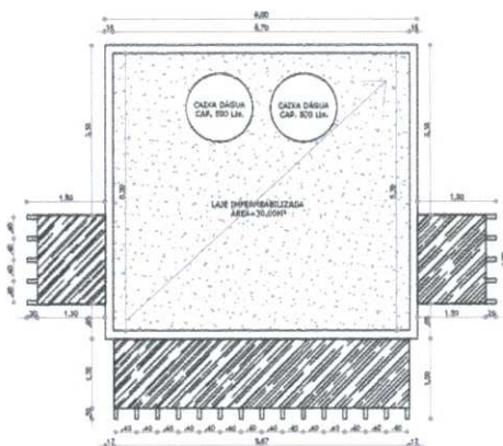
COBERTA
