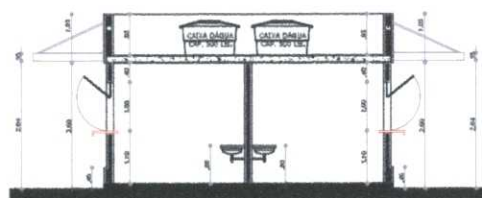
CORTE AA
