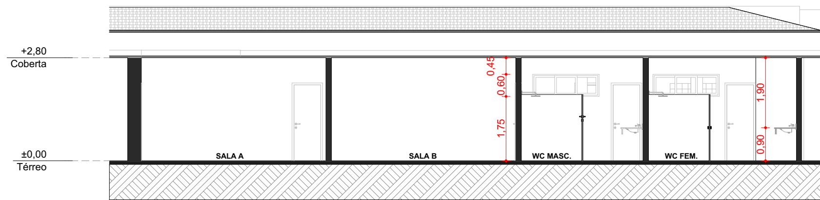
2 CORTE A ESC.: 1:100
