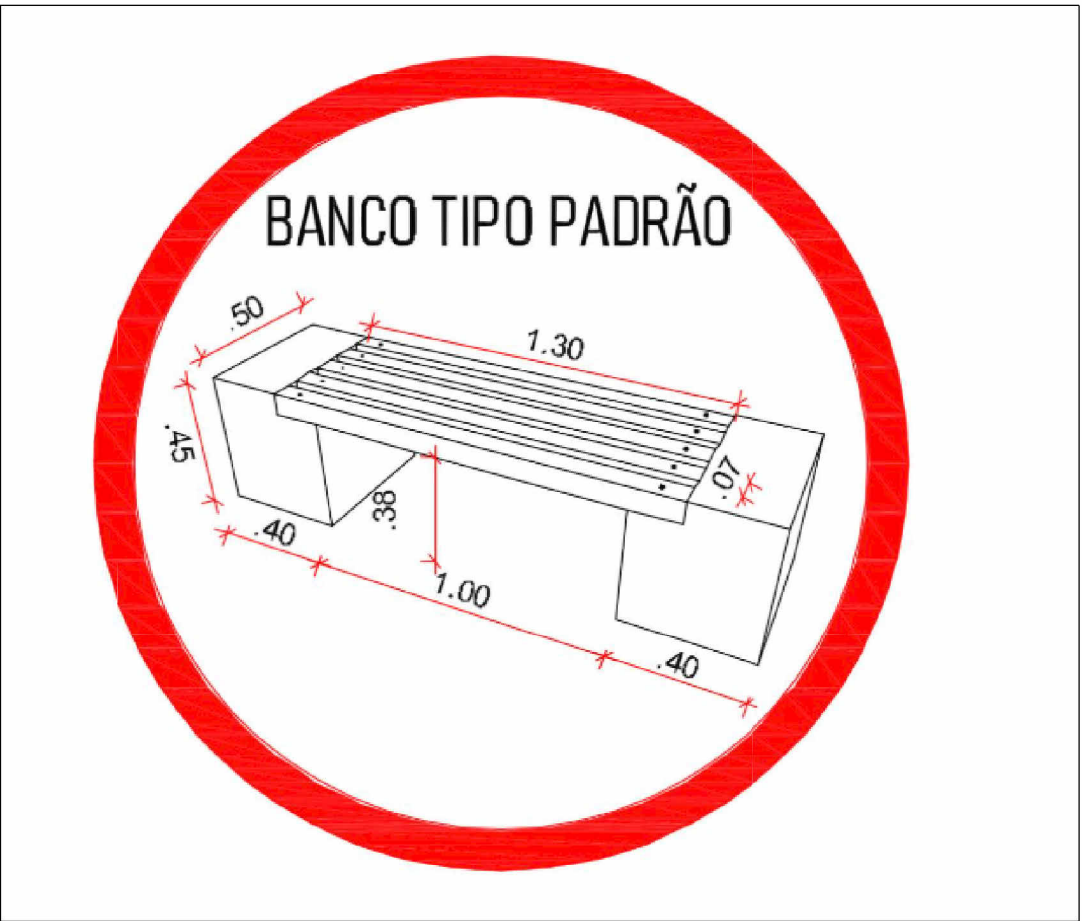
DETALHAMENTO BANCO
