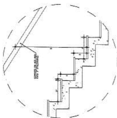
DET. ESCADA/CORRIMÃO
