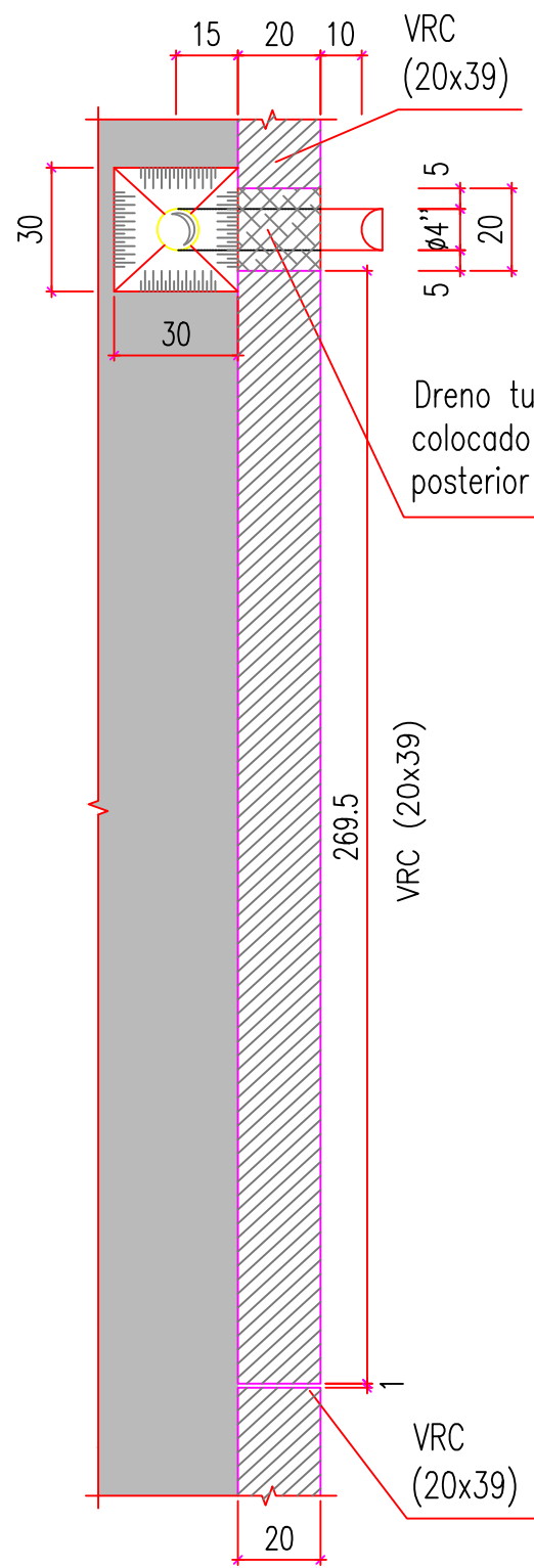
DRENAGEM TRANSVERSAL DAS LAJES DE TRANSIÇÃO Esc.: 1:25 (A1) Esc.: 1:50 (A3)
