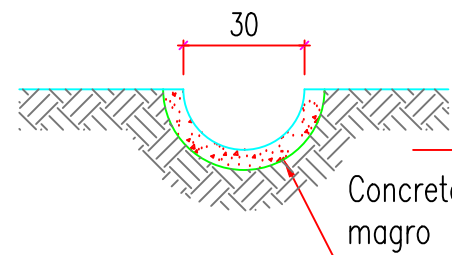
CALEIRA DE DESCIDA DE ÁGUAS NOS TALUDES Esc.: 1:25 (A1) Esc.: 1:50 (A3)
