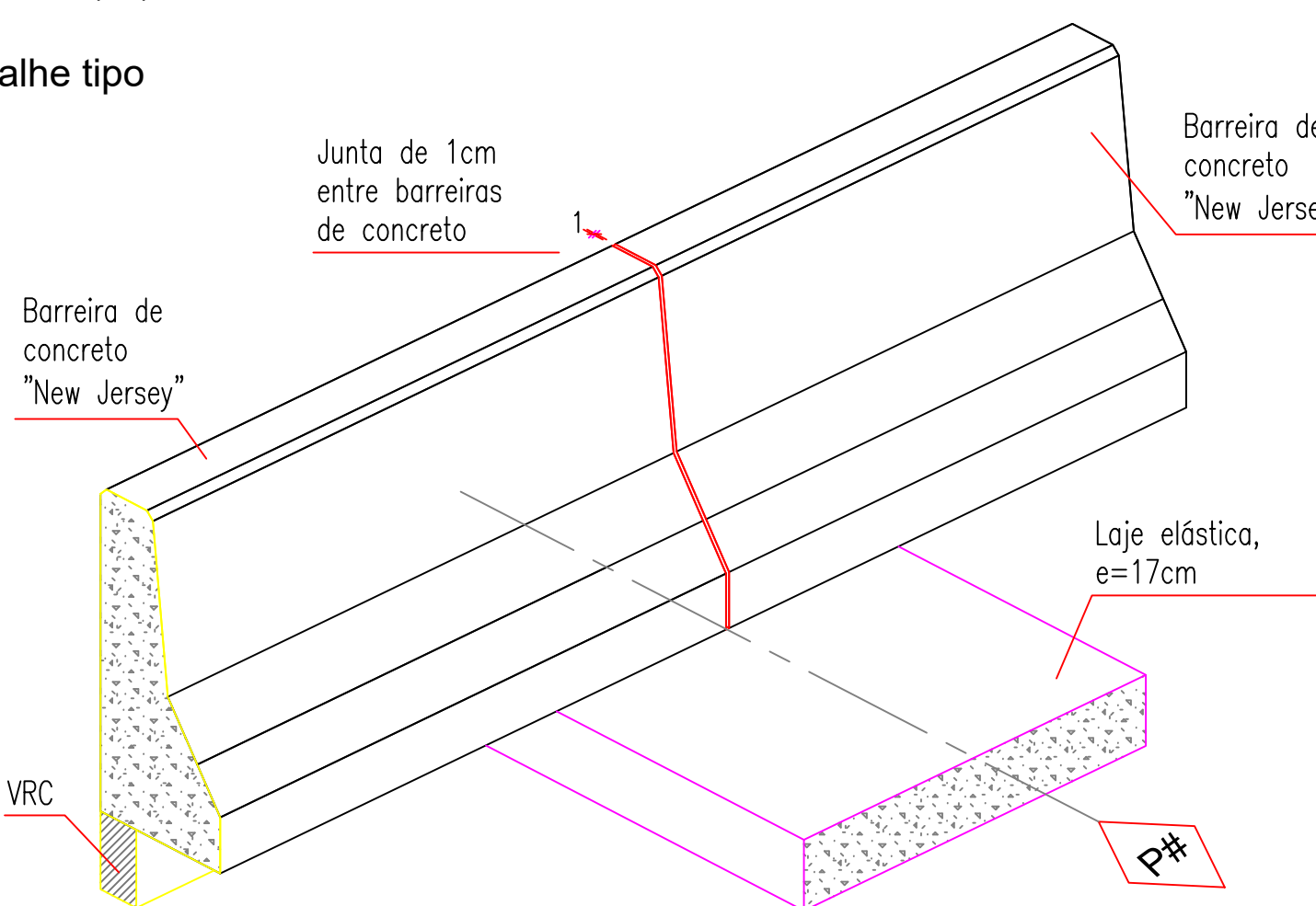
BARREIRAS DE CONCRETO "NEW JERSEY" SOBRE A LAJE ELÁSTICA Esc.: 1:25 (A1) Esc.: 1:50 (A3)
