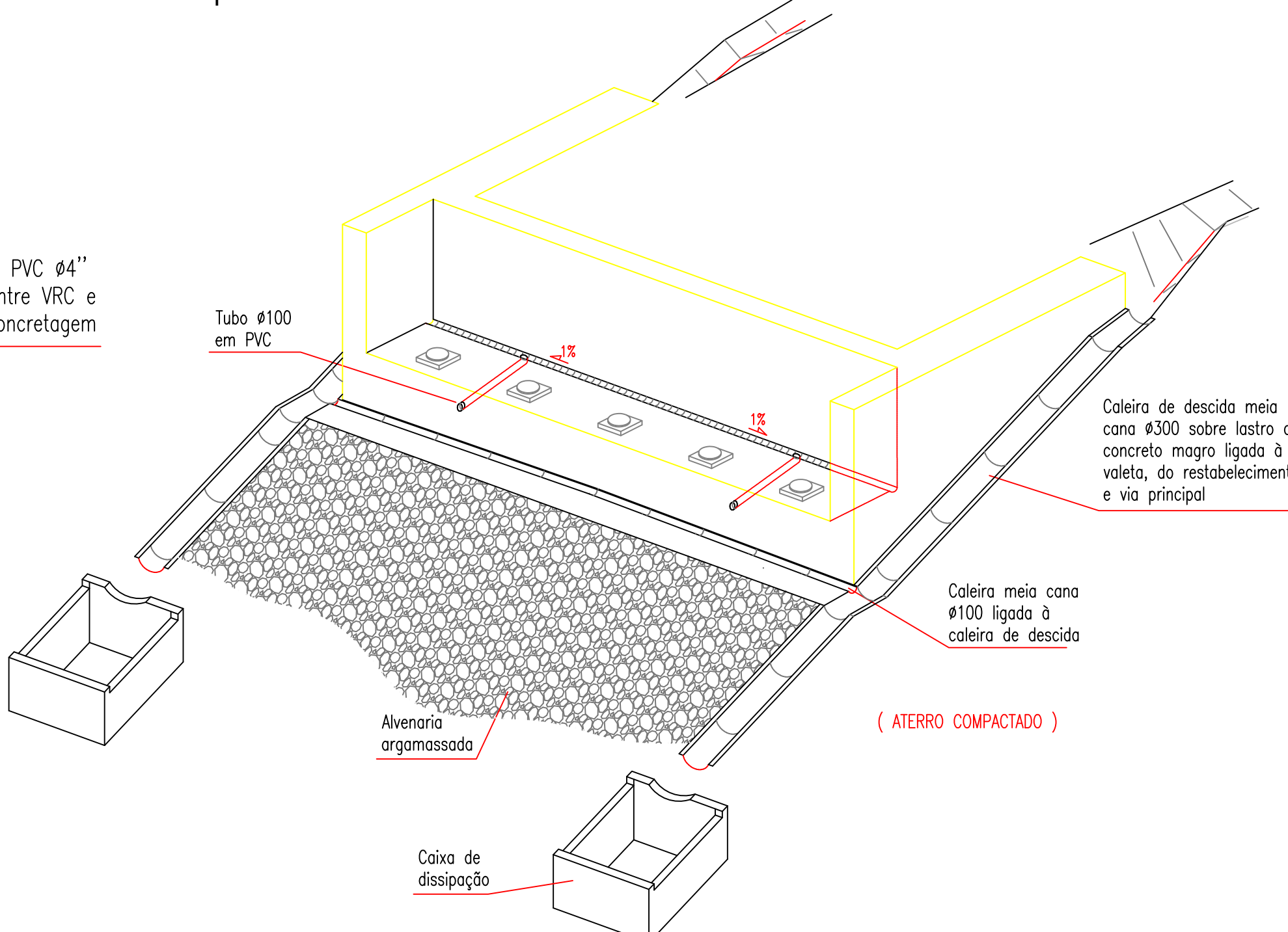
DRENAGEM DOS ENCONTROS S/ESC.
