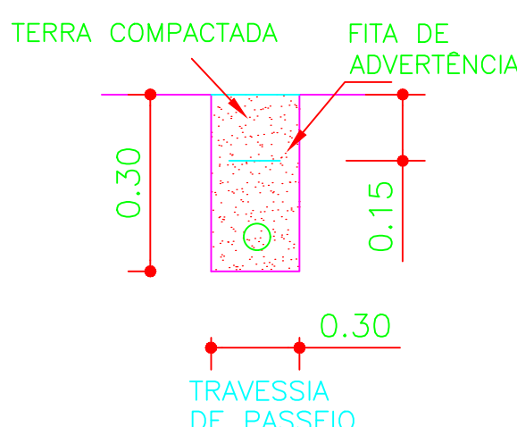
06 DETALHE DE TRAVESSIA SEM ESCALA
