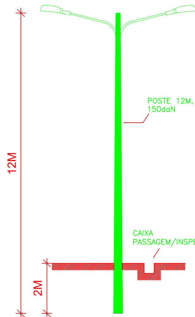
05 DETALHE DE POSTE SEM ESCALA
