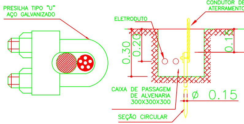
06 DETALHE DE CAIXA DE INSPEÇÃO /PASSAGEM P/ ATERRAMENTO SEM ESCALA
