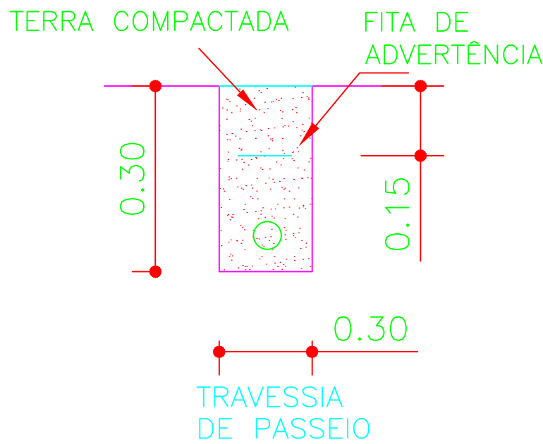
06 DETALHE DE TRAVESSIA SEM ESCALA
