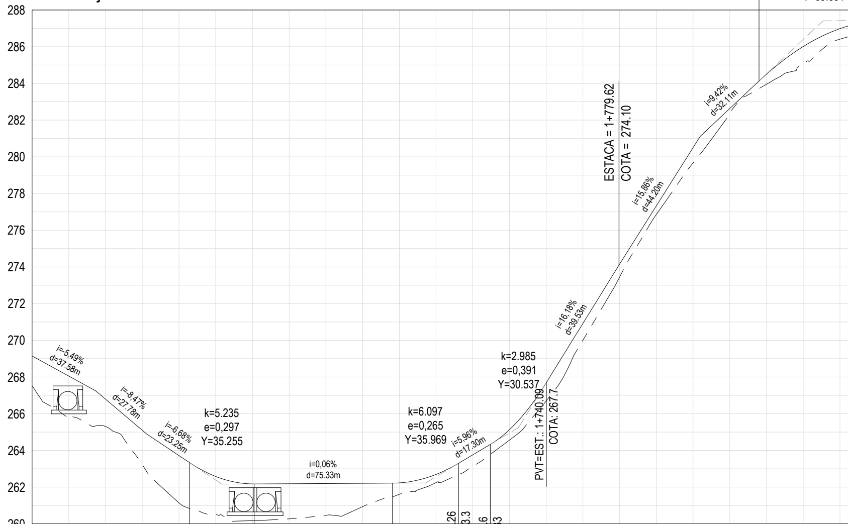
EIXO - PIÇARRAMENTO PROFILE
