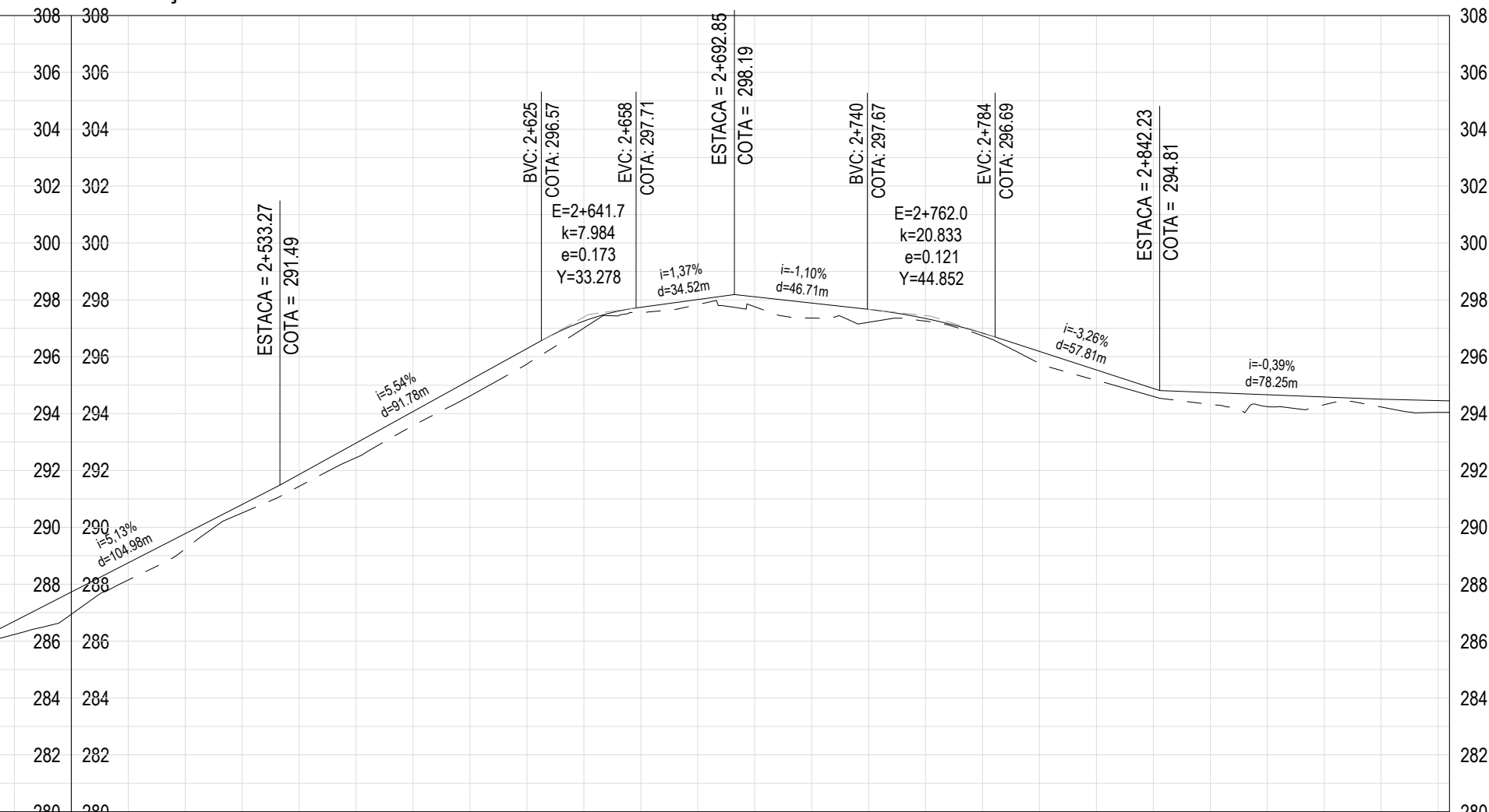
EIXO - PIÇARRAMENTO PROFILE
