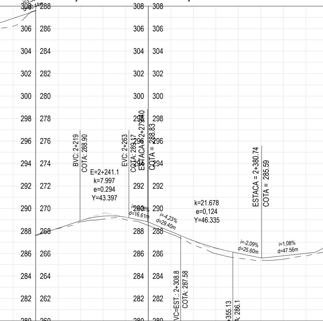
EIXO - PIÇARRAMENTO PROFILE
