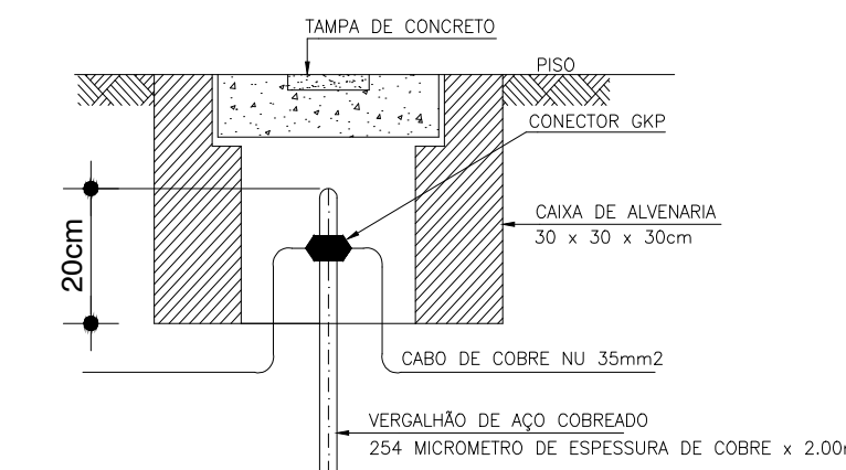
DETALHE ATERRAMENTO - SEM ESCALA
