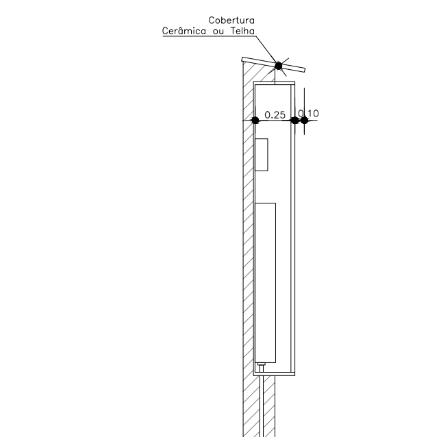
VISTA EM CORTE
