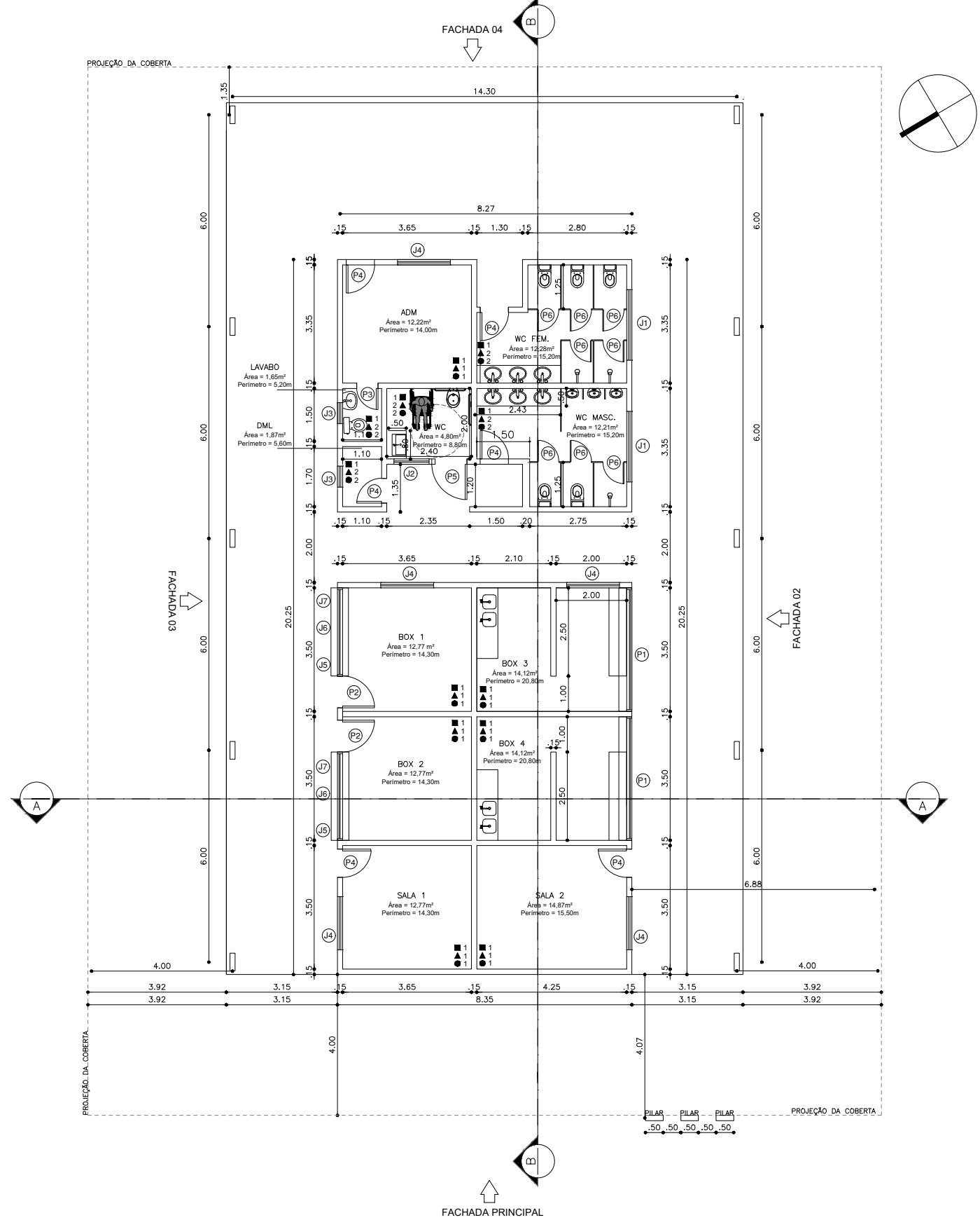
03 PLANTA BAIXA ESC. 1/75
