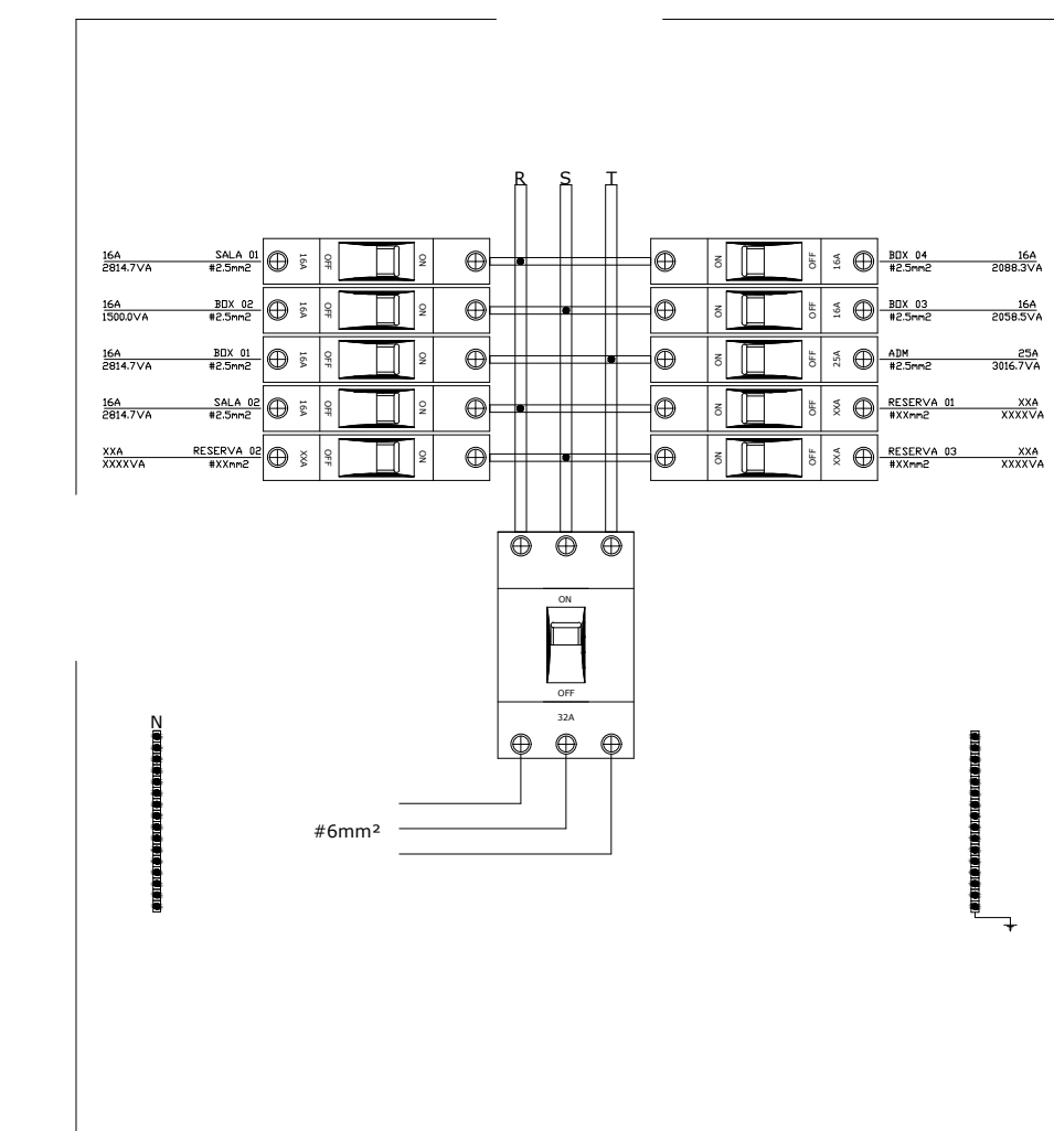
DETALHE BARRAMENTO - SEM ESCALA
